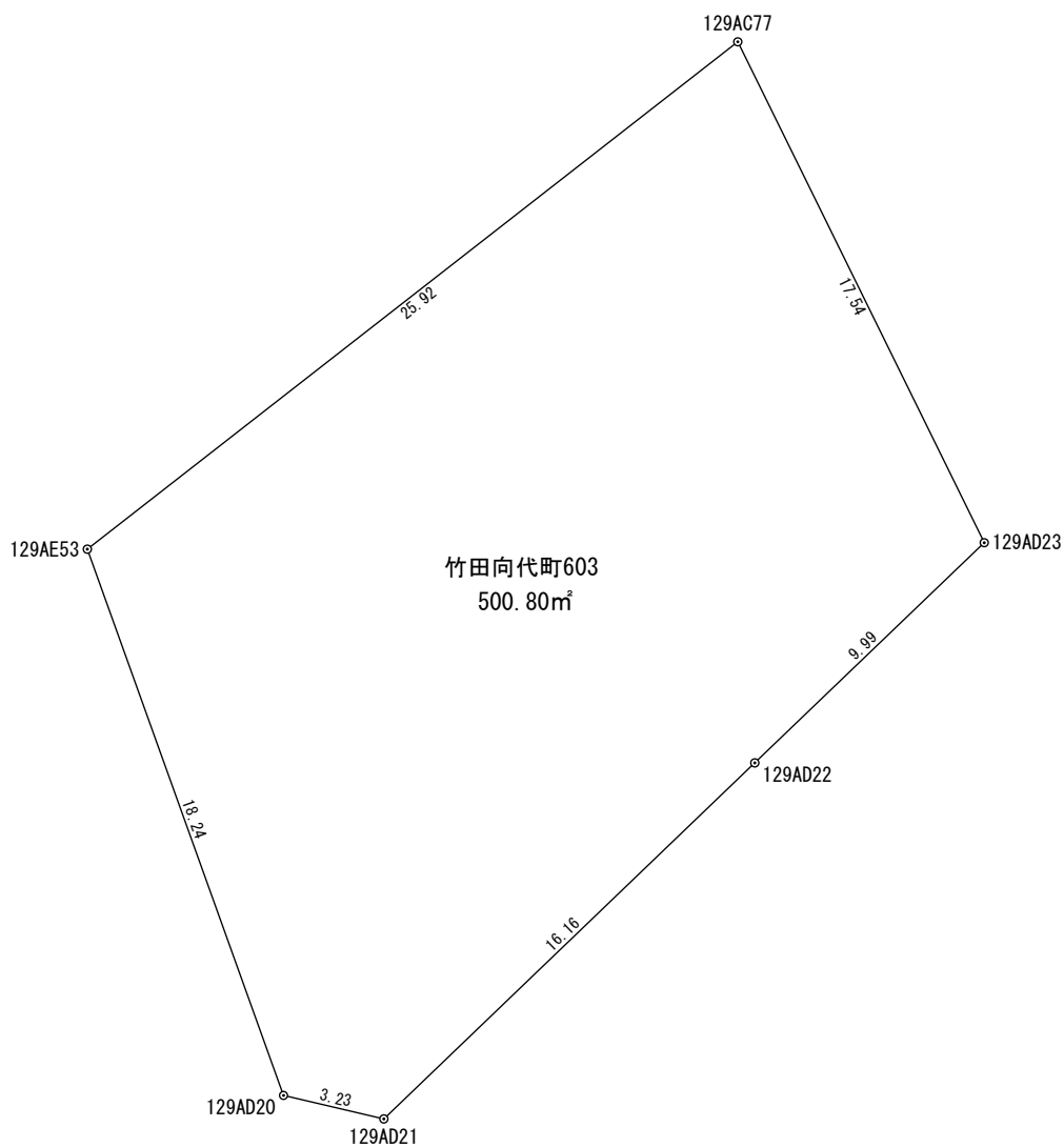
座 標 求 積 表
