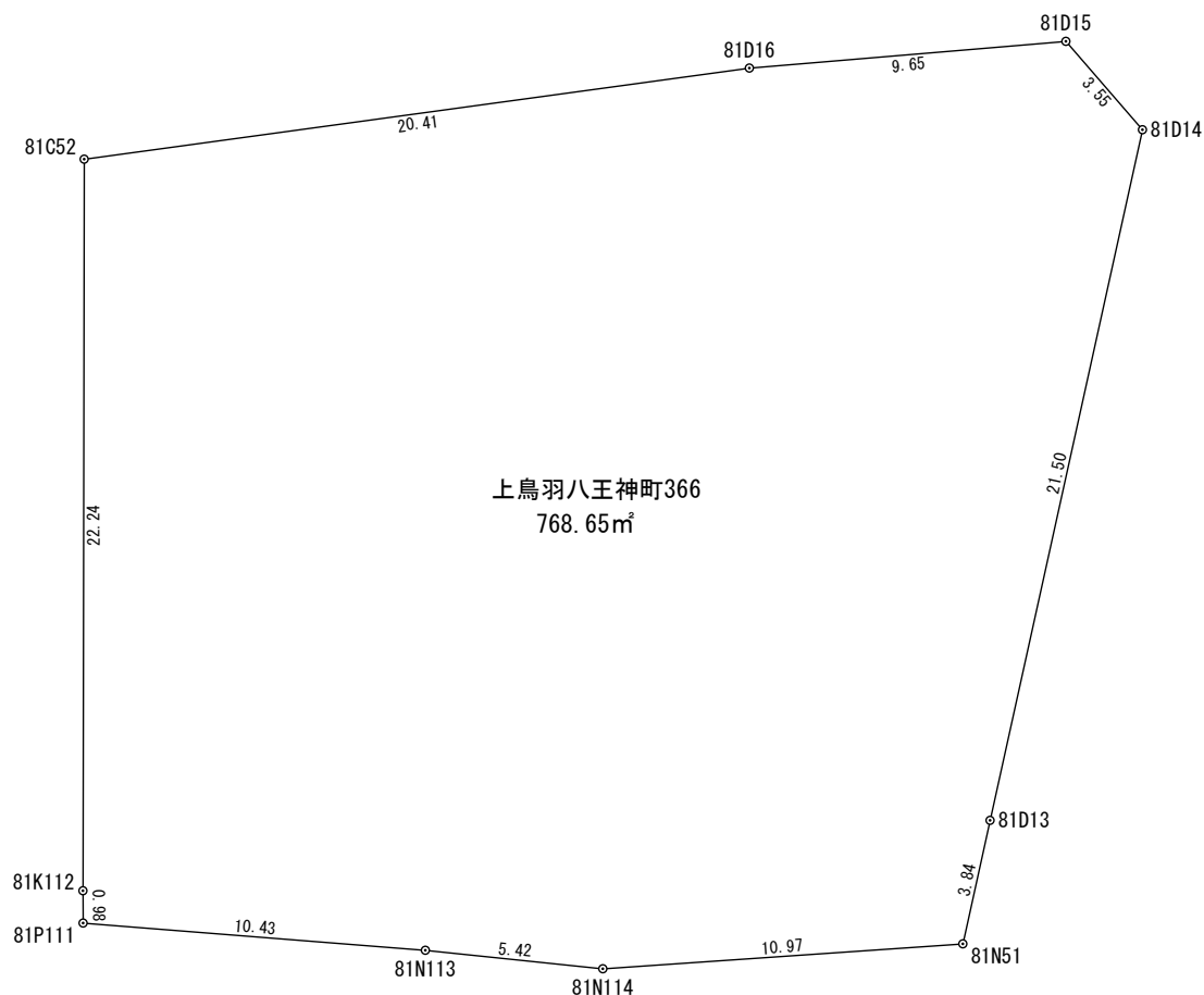
座 標 求 積 表
