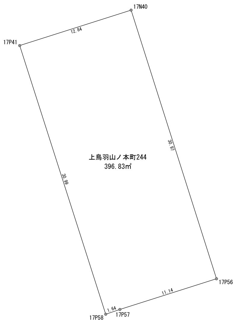
座 標 求 積 表
