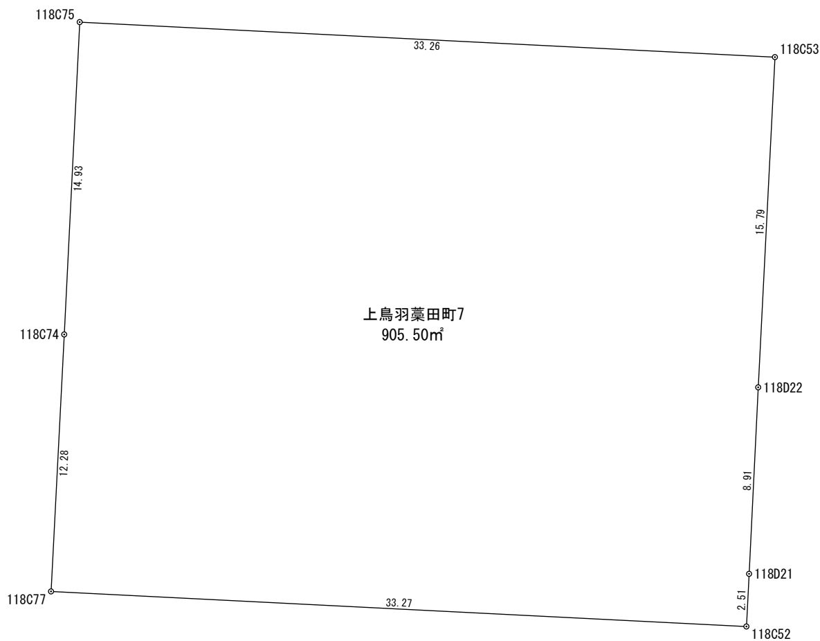
座 標 求 積 表
