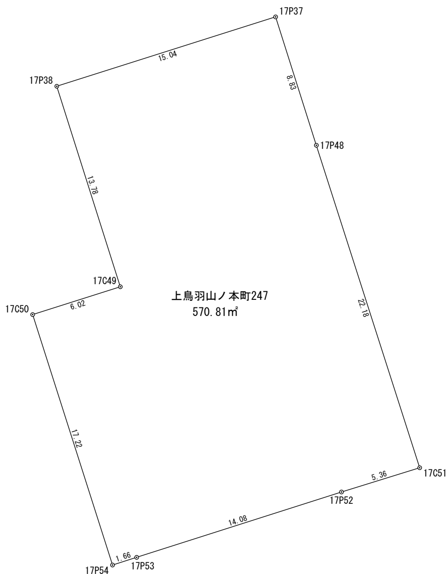
座 標 求 積 表
