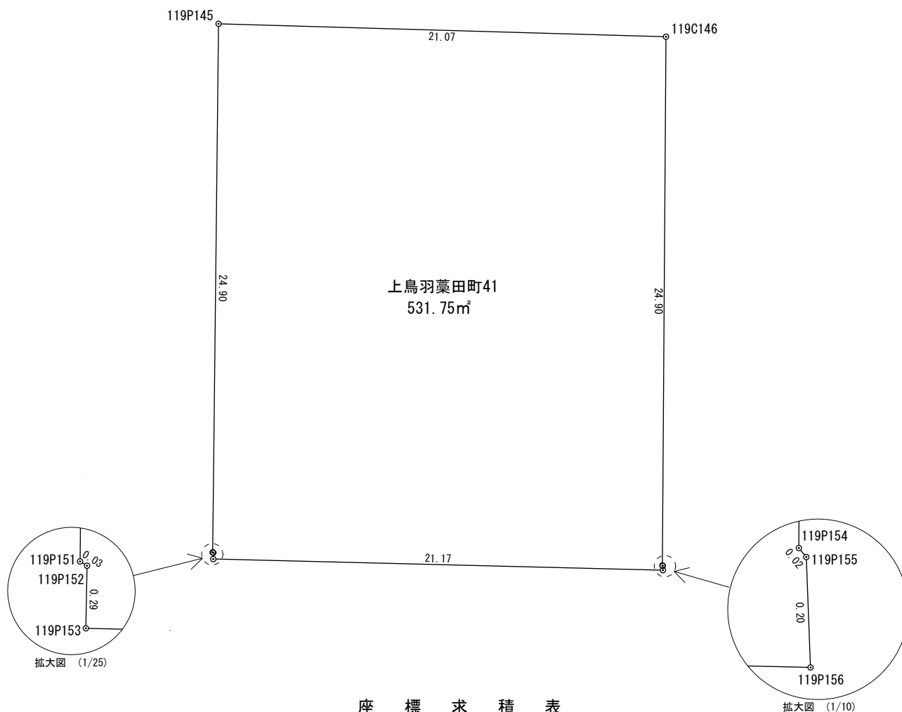
座 標 求 積 表
