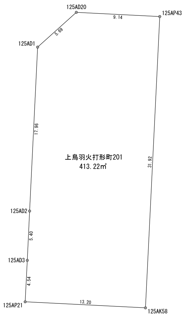
座 標 求 積 表
