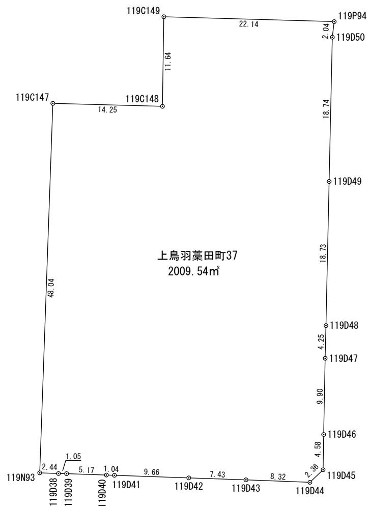
座 標 求 積 表
