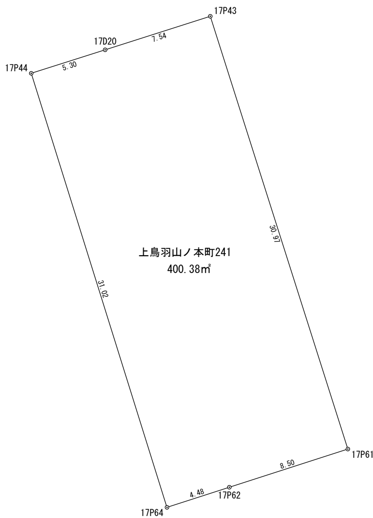
座 標 求 積 表
