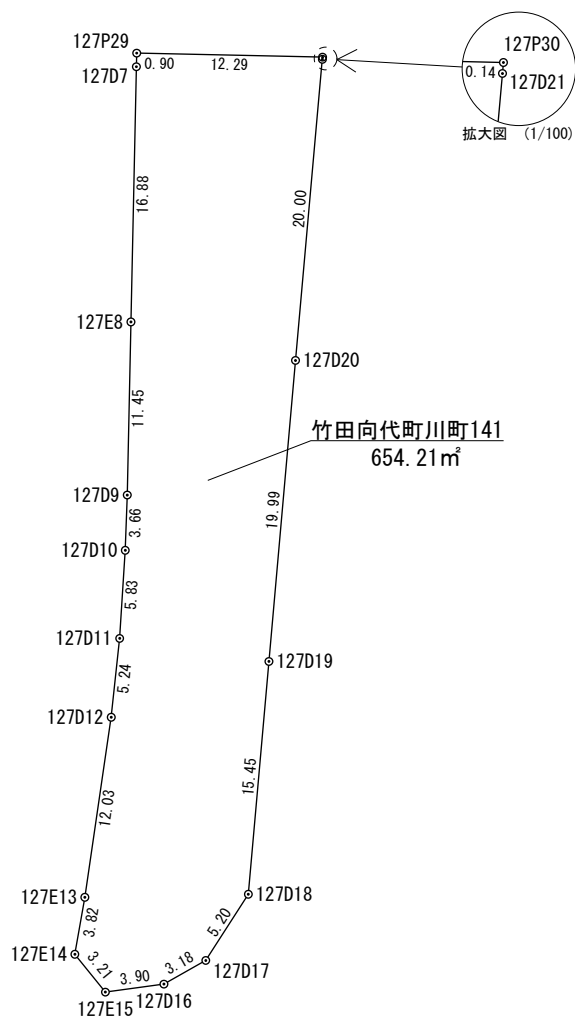
座 標 求 積 表
