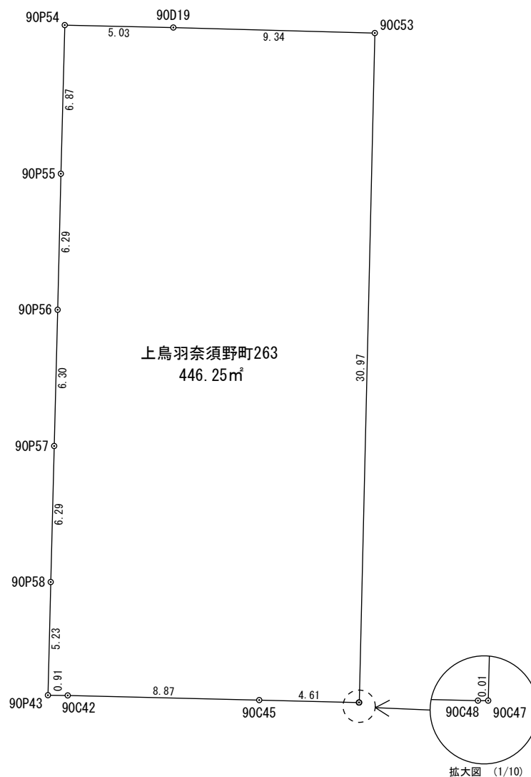
座 標 求 積 表
