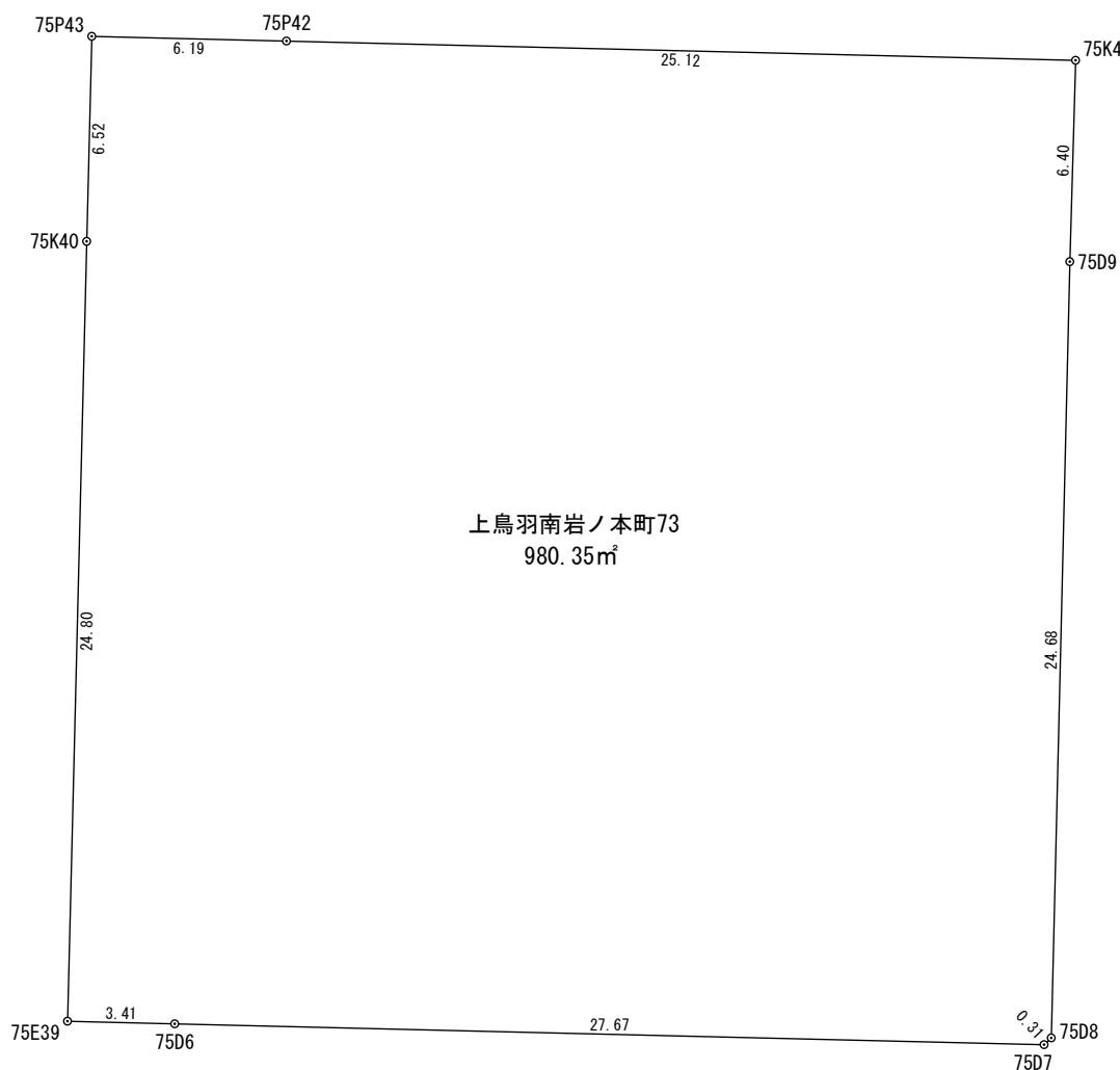
座 標 求 積 表
