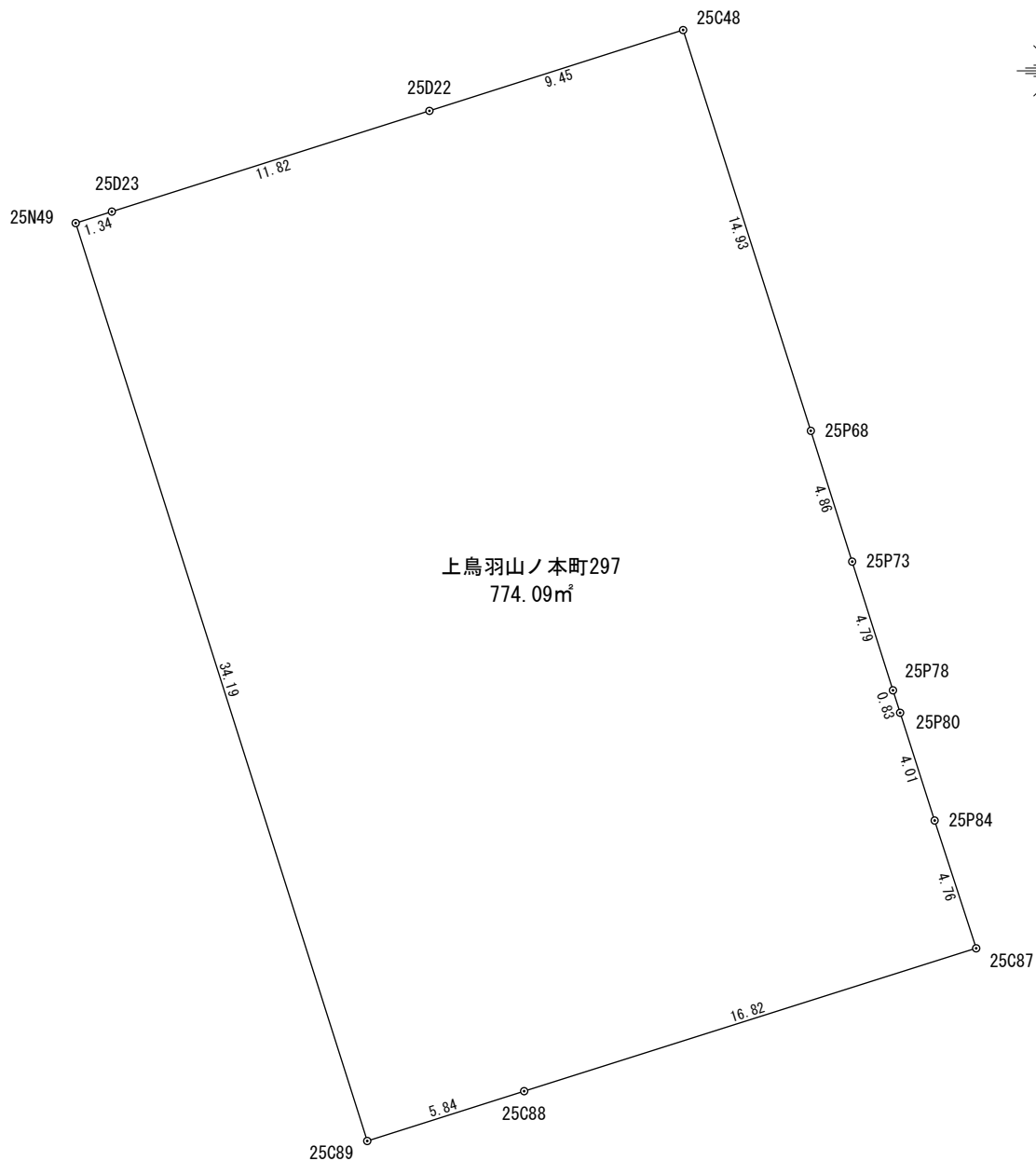
座 標 求 積 表
