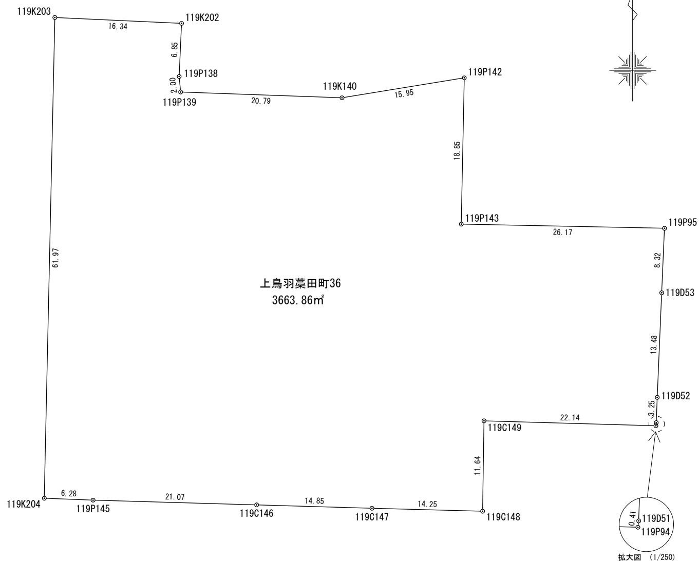
座 標 求 積 表
