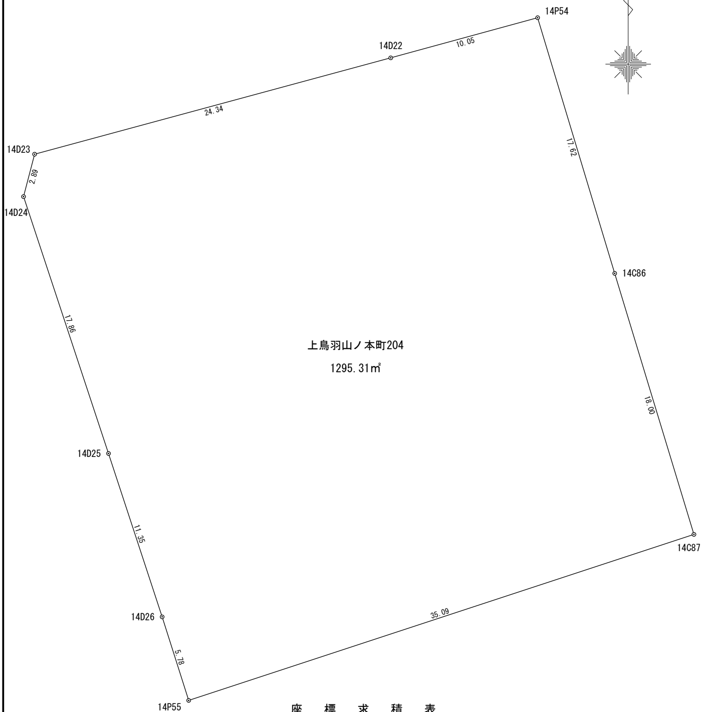
座 標 求 積 表
