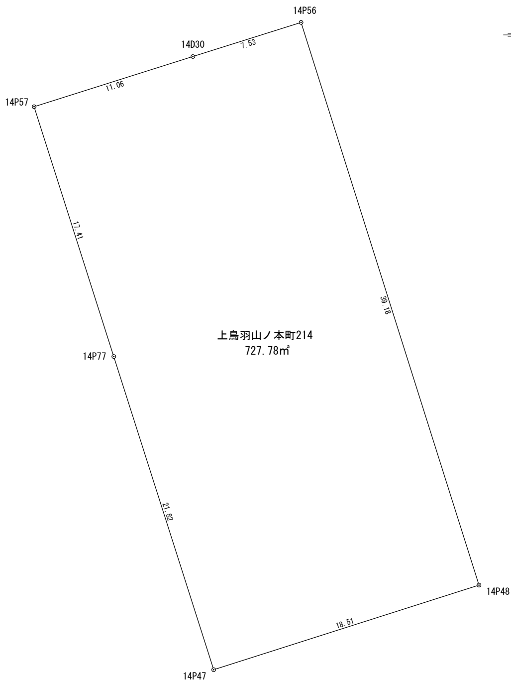
座 標 求 積 表
