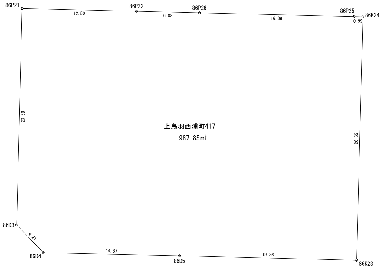
座 標 求 積 表
