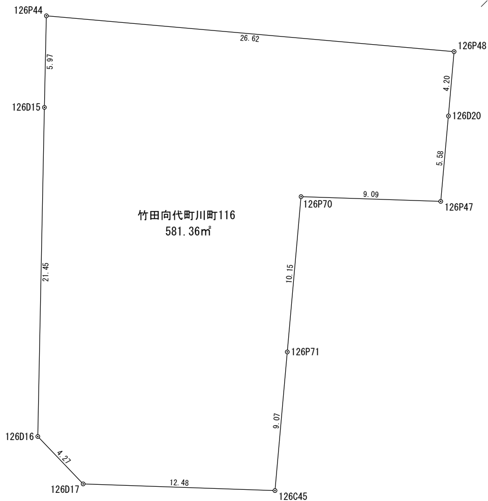
座 標 求 積 表
