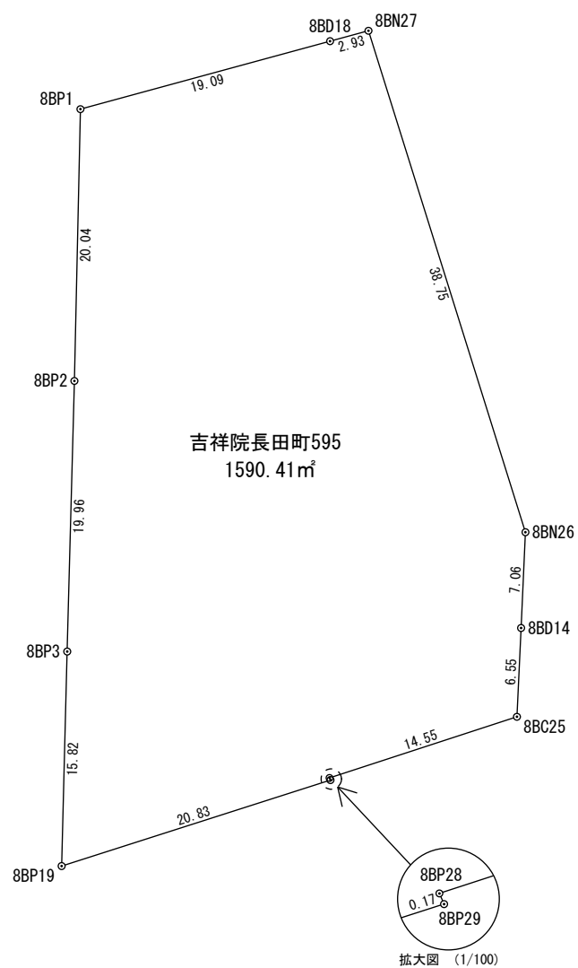
座 標 求 積 表
