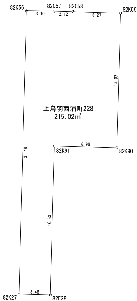
座 標 求 積 表
