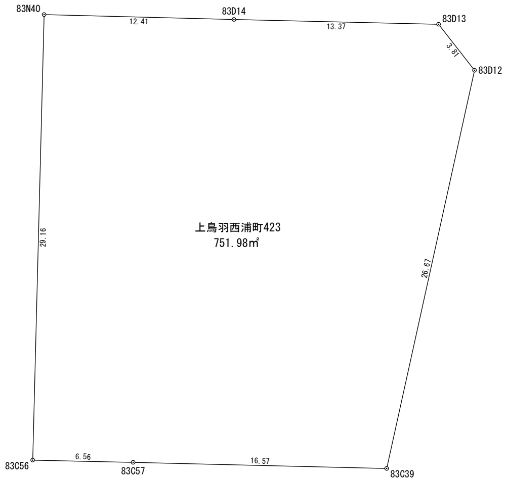
座 標 求 積 表
