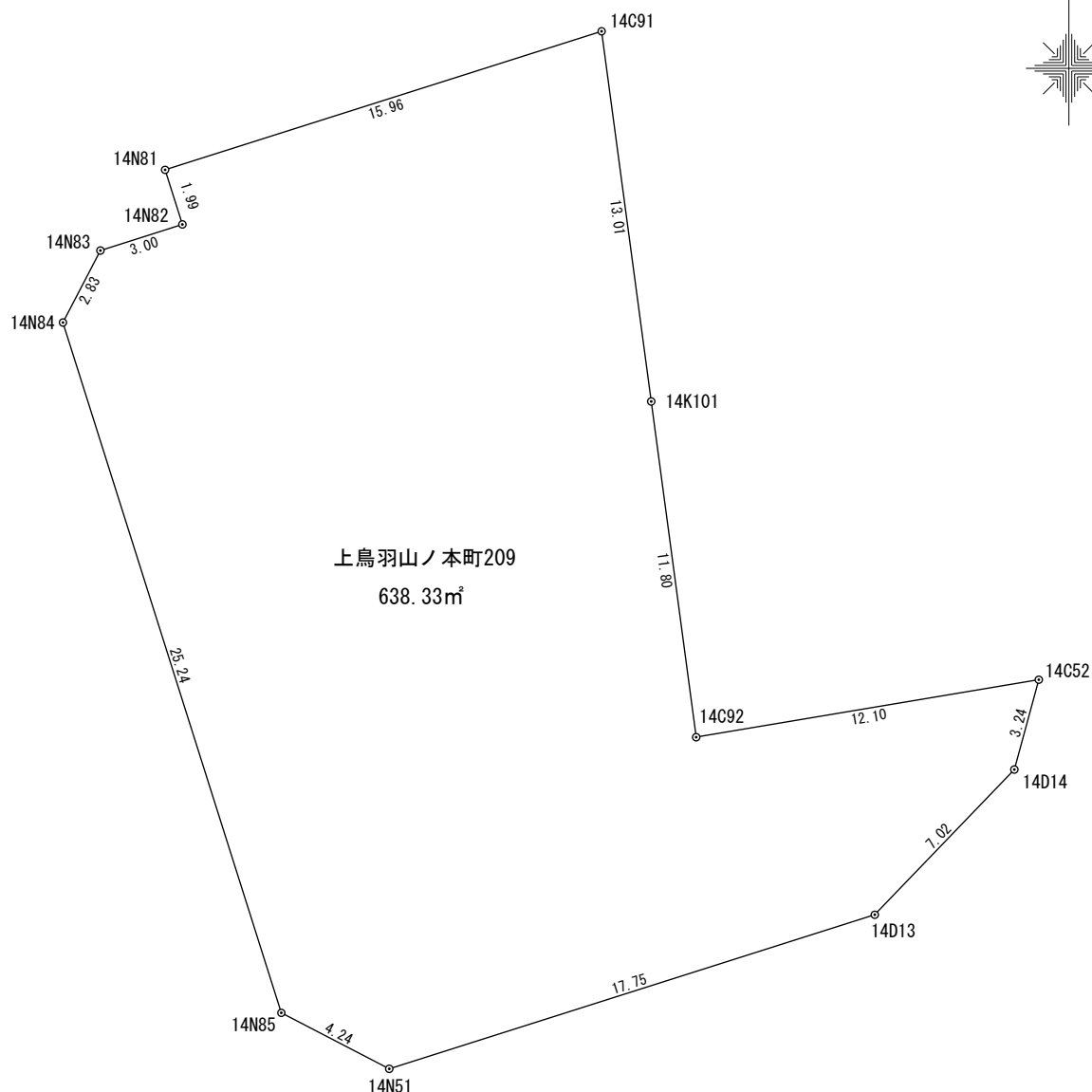
座 標 求 積 表
