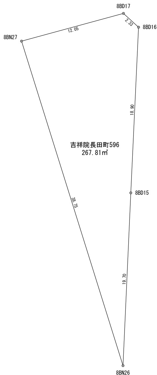
座 標 求 積 表
