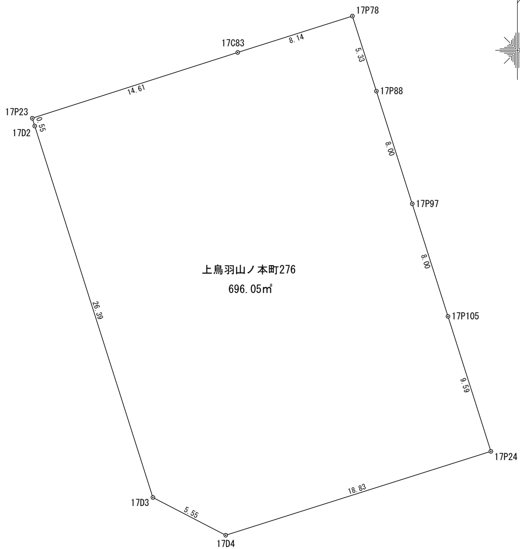
座 標 求 積 表
