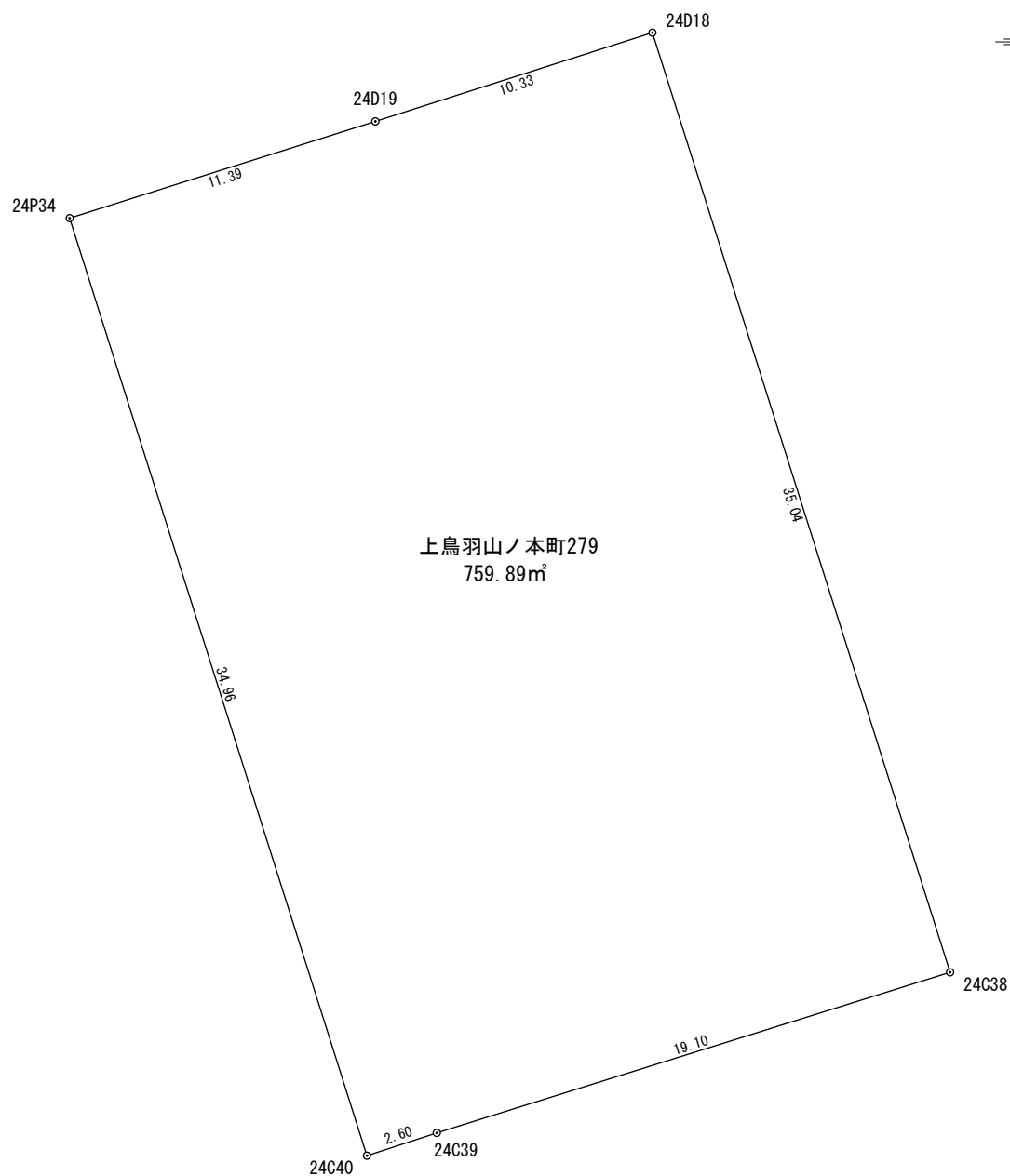
座 標 求 積 表
