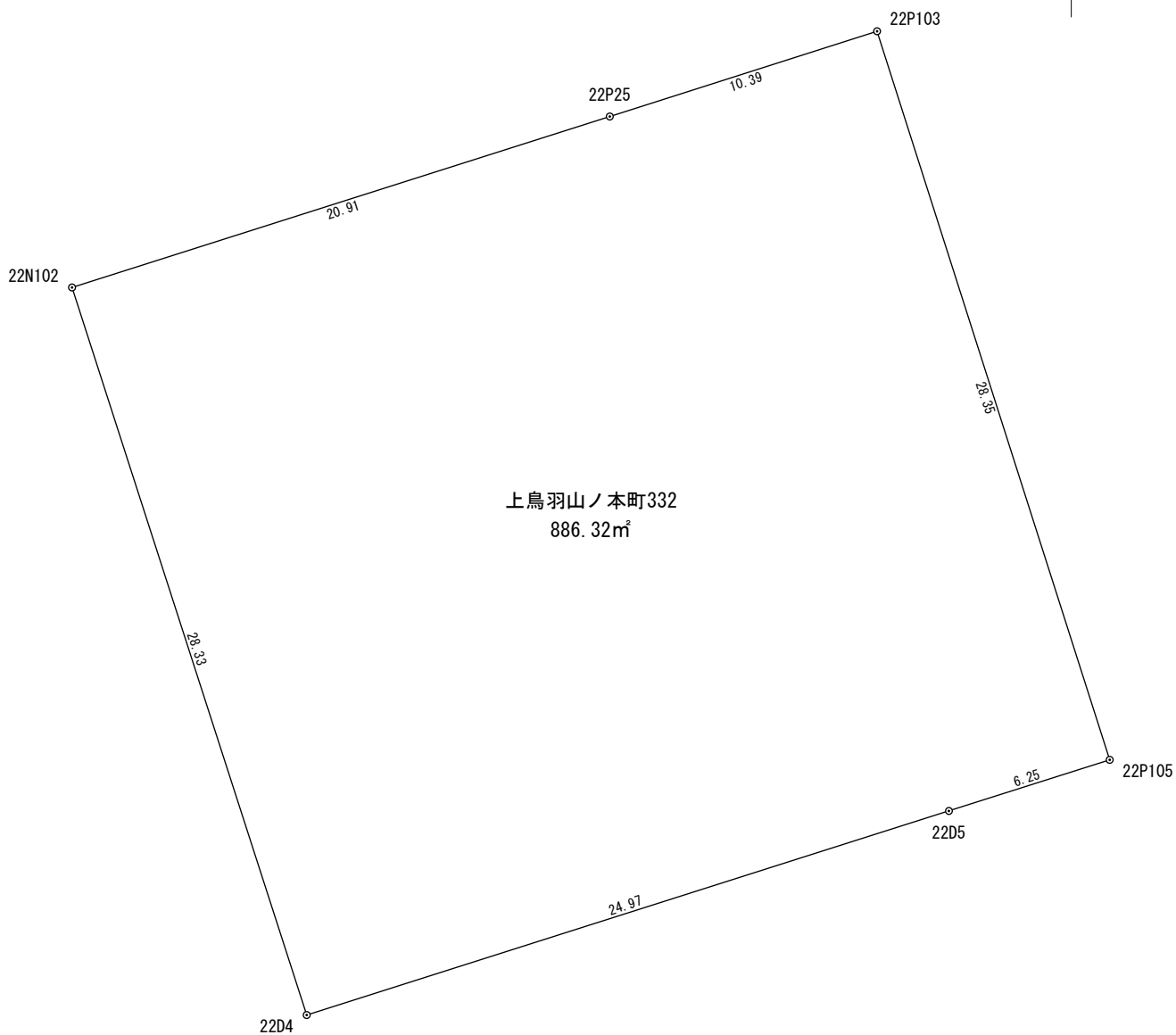
座 標 求 積 表
