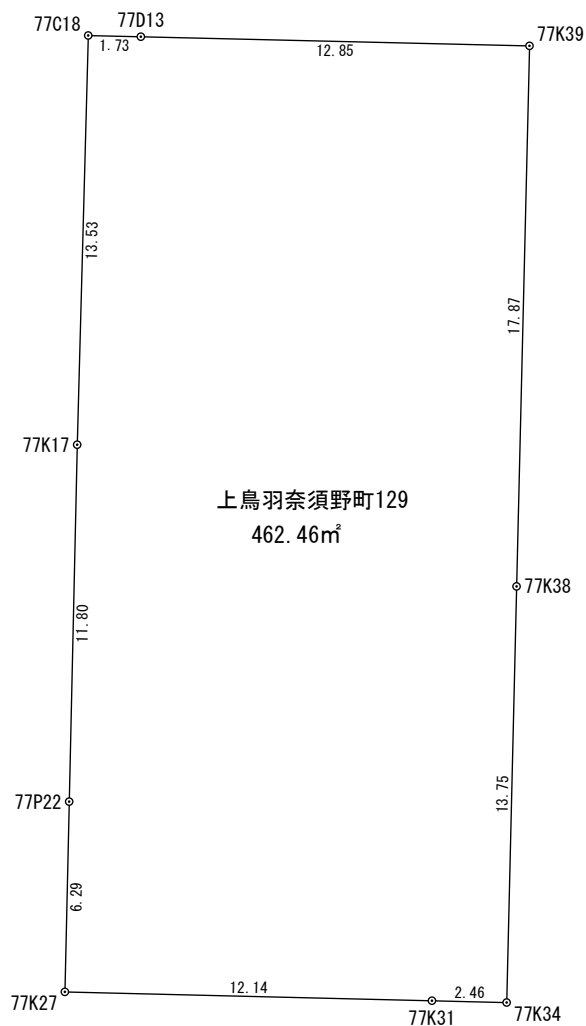
座 標 求 積 表
