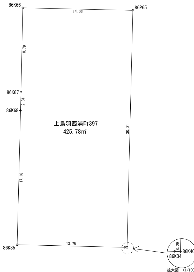
座 標 求 積 表
