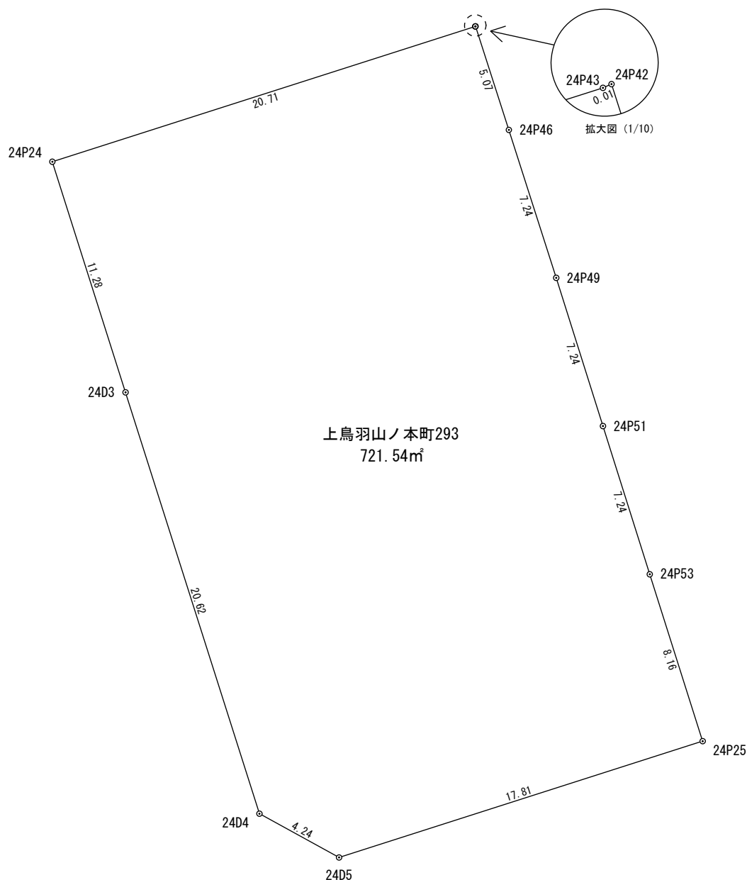
座 標 求 積 表
