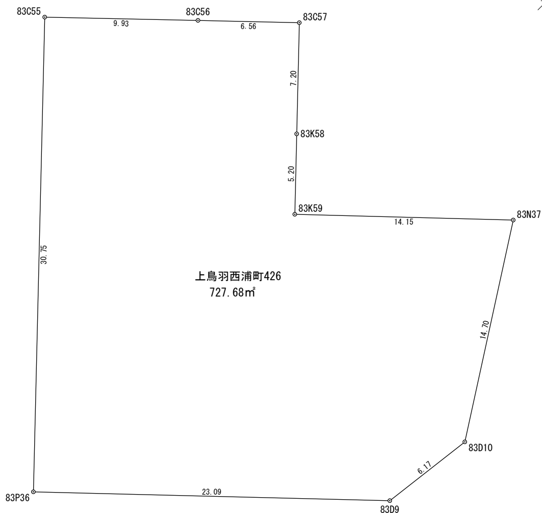
座 標 求 積 表
