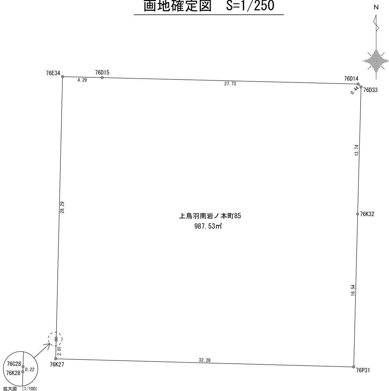
座 標 求 積 表
