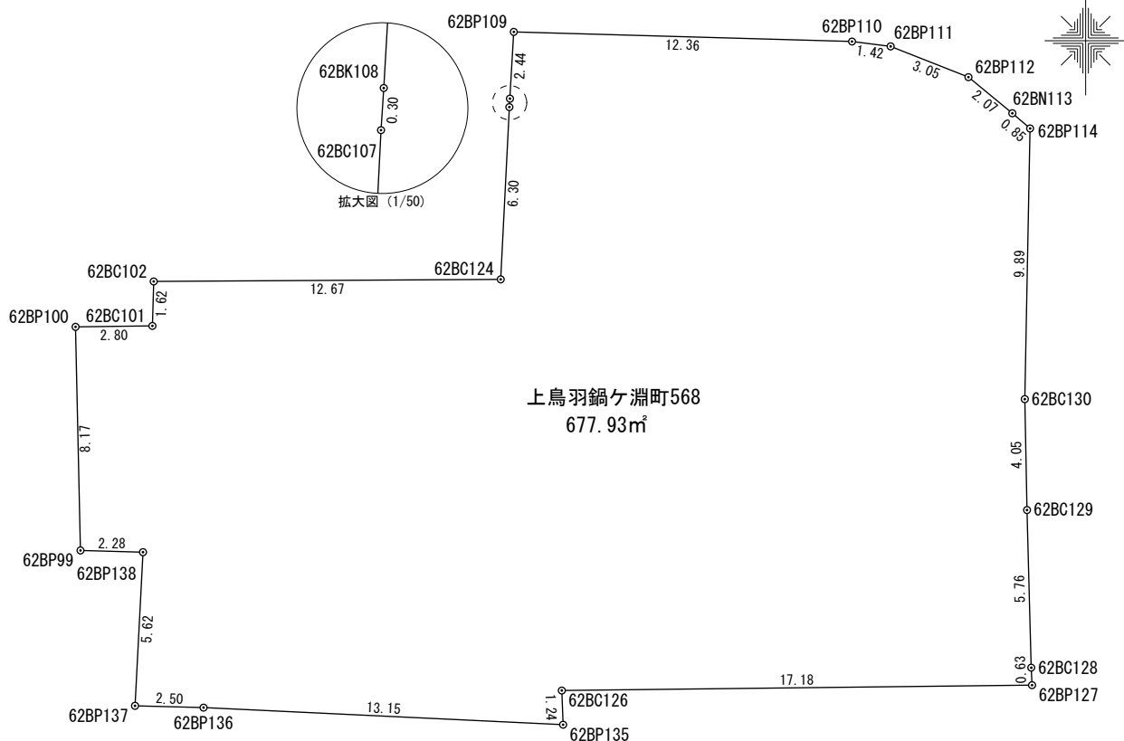
座 標 求 積 表
