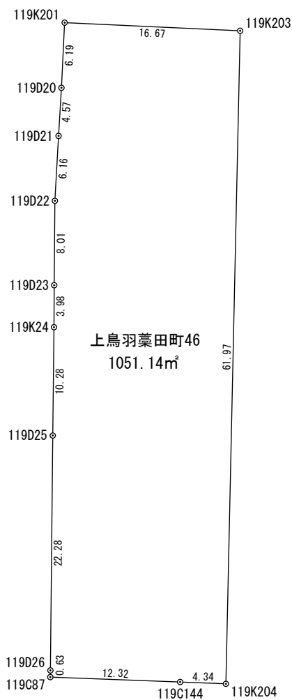
座 標 求 積 表
