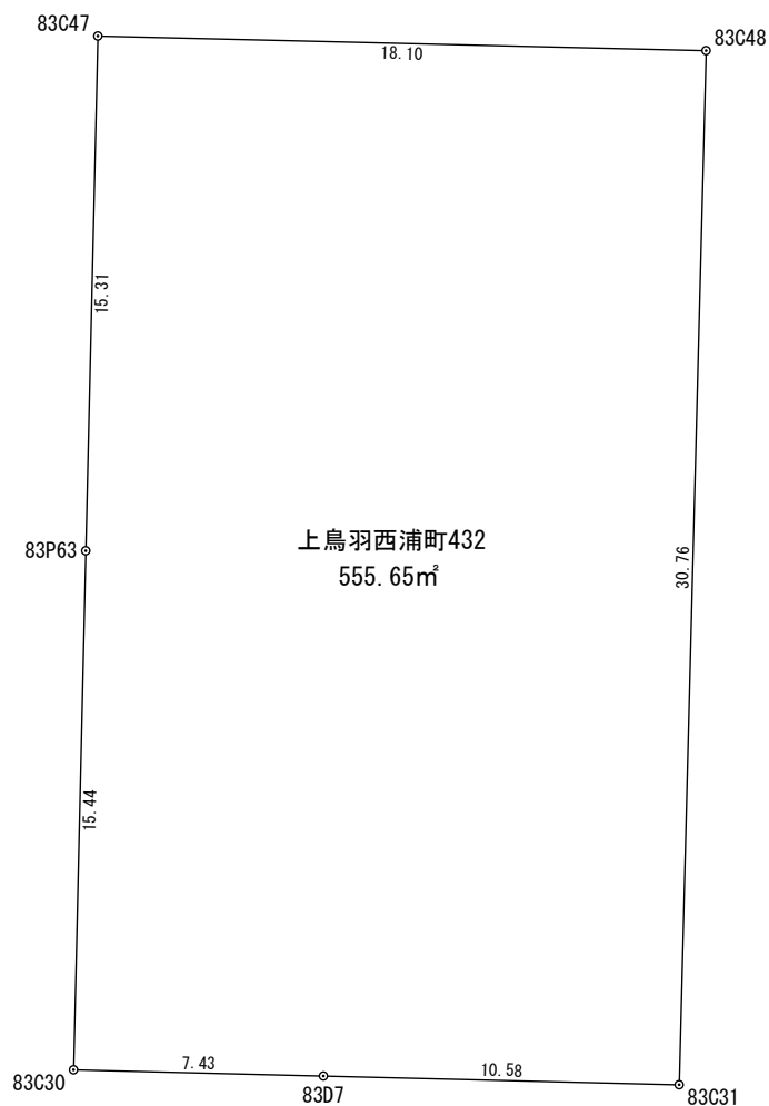
座 標 求 積 表
