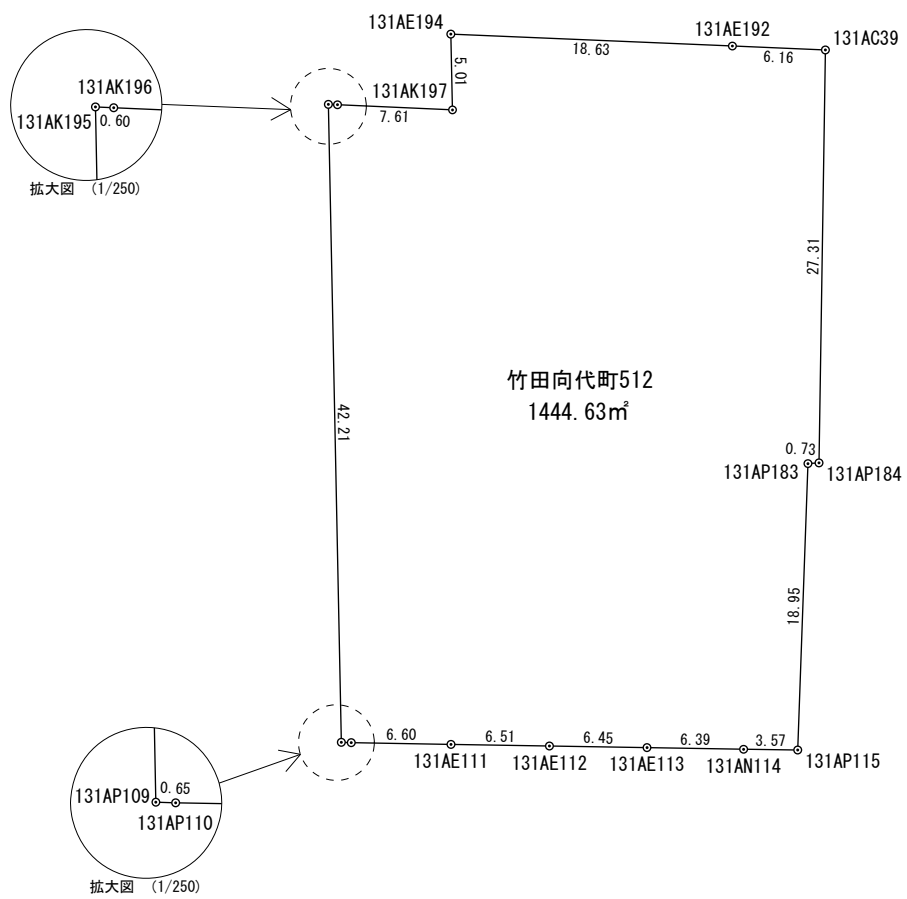
座 標 求 積 表
