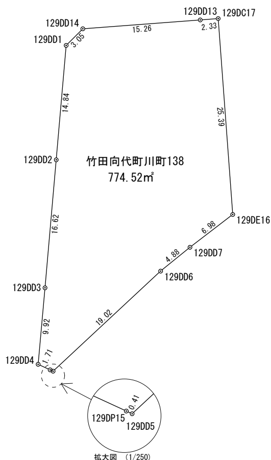
座 標 求 積 表
