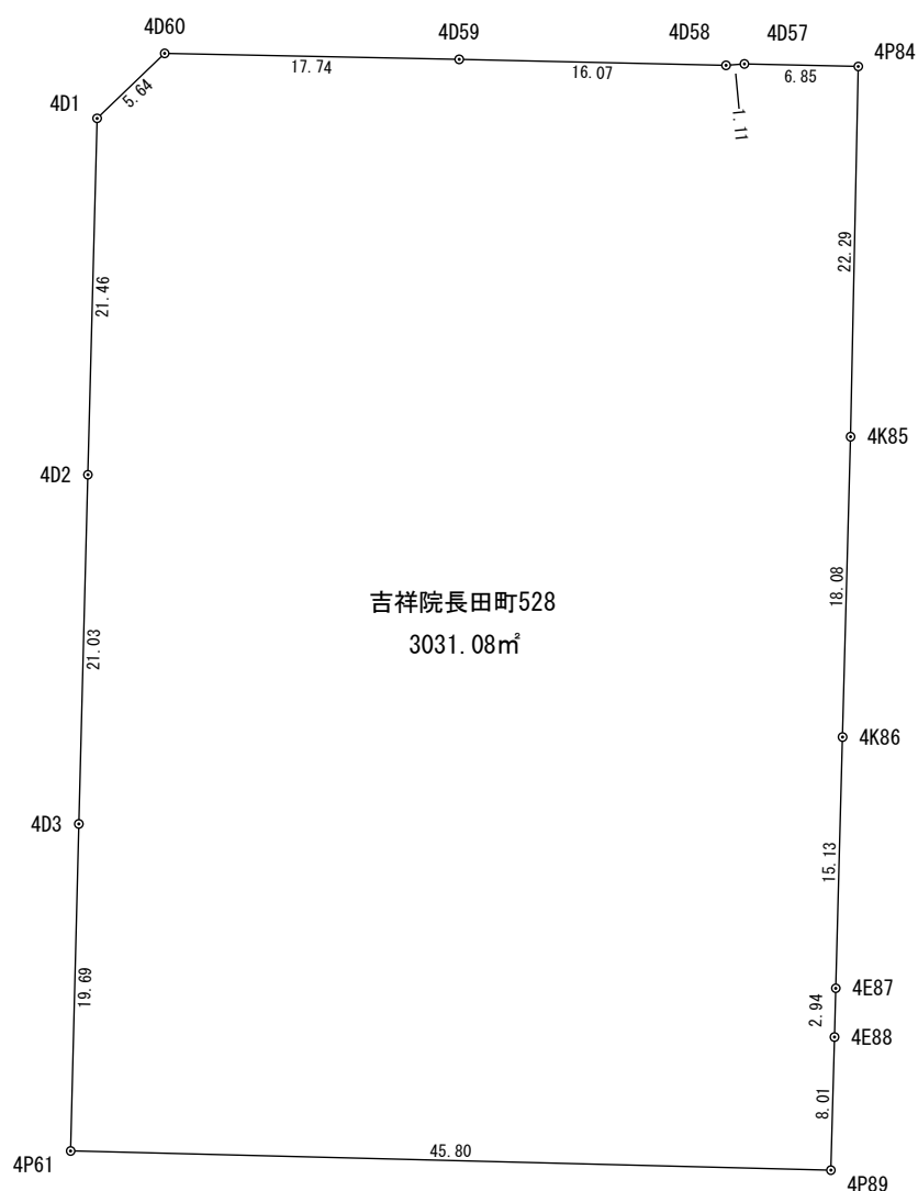
座 標 求 積 表
