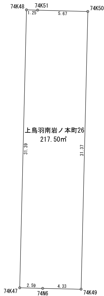
座 標 求 積 表
