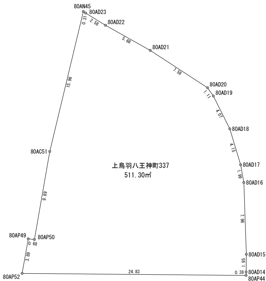
座 標 求 積 表
