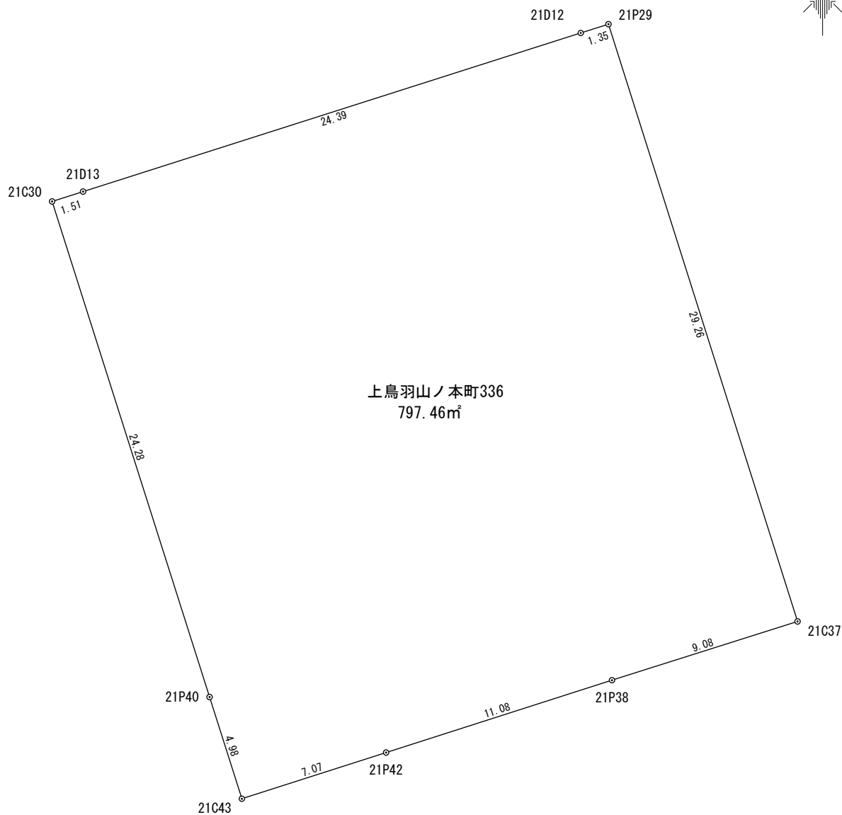
座 標 求 積 表
