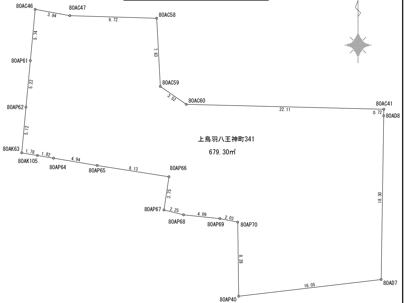
座 標 求 積 表
