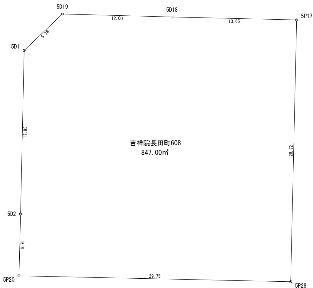
座 標 求 積 表
