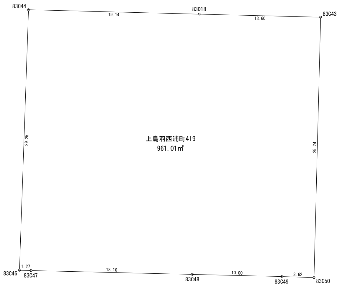
座 標 求 積 表
