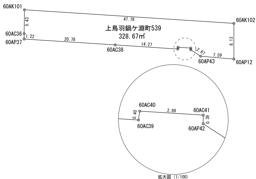
座 標 求 積 表
