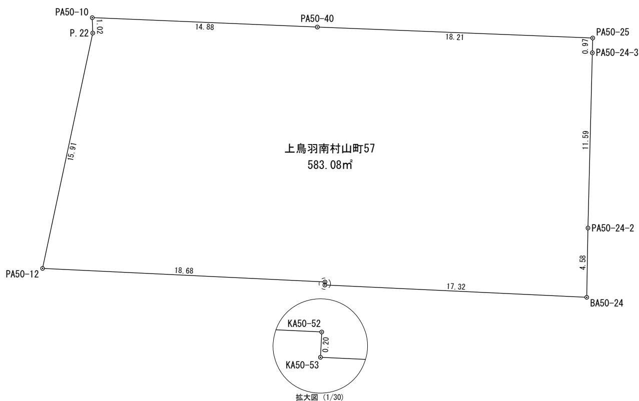
座 標 求 積 表
