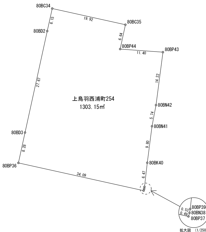
座 標 求 積 表
