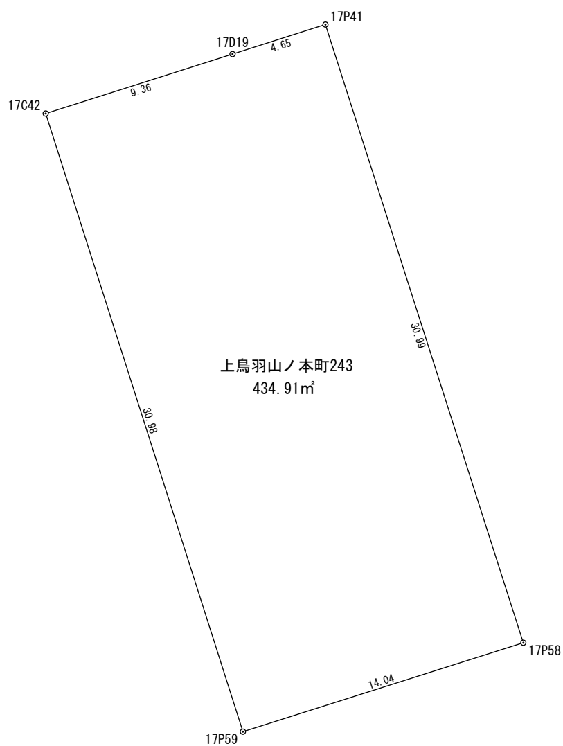
座 標 求 積 表
