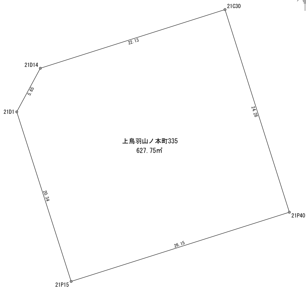
座 標 求 積 表
