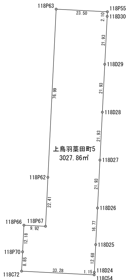
座 標 求 積 表
