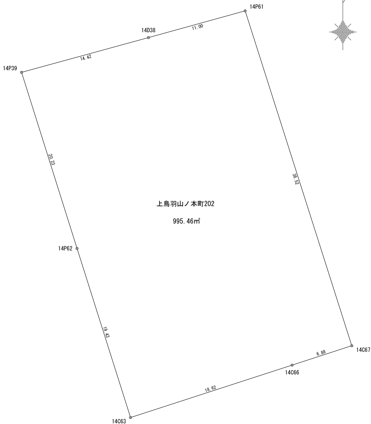
座 標 求 積 表
