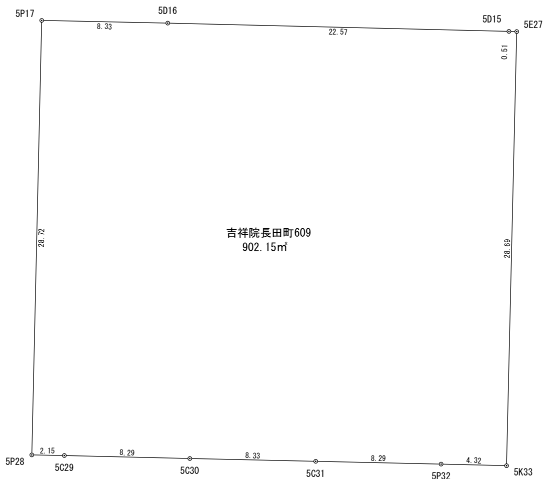
座 標 求 積 表
