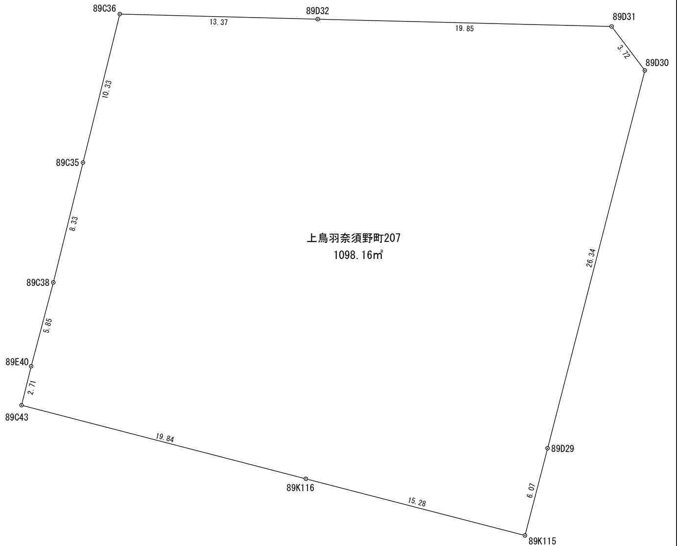
座 標 求 積 表
