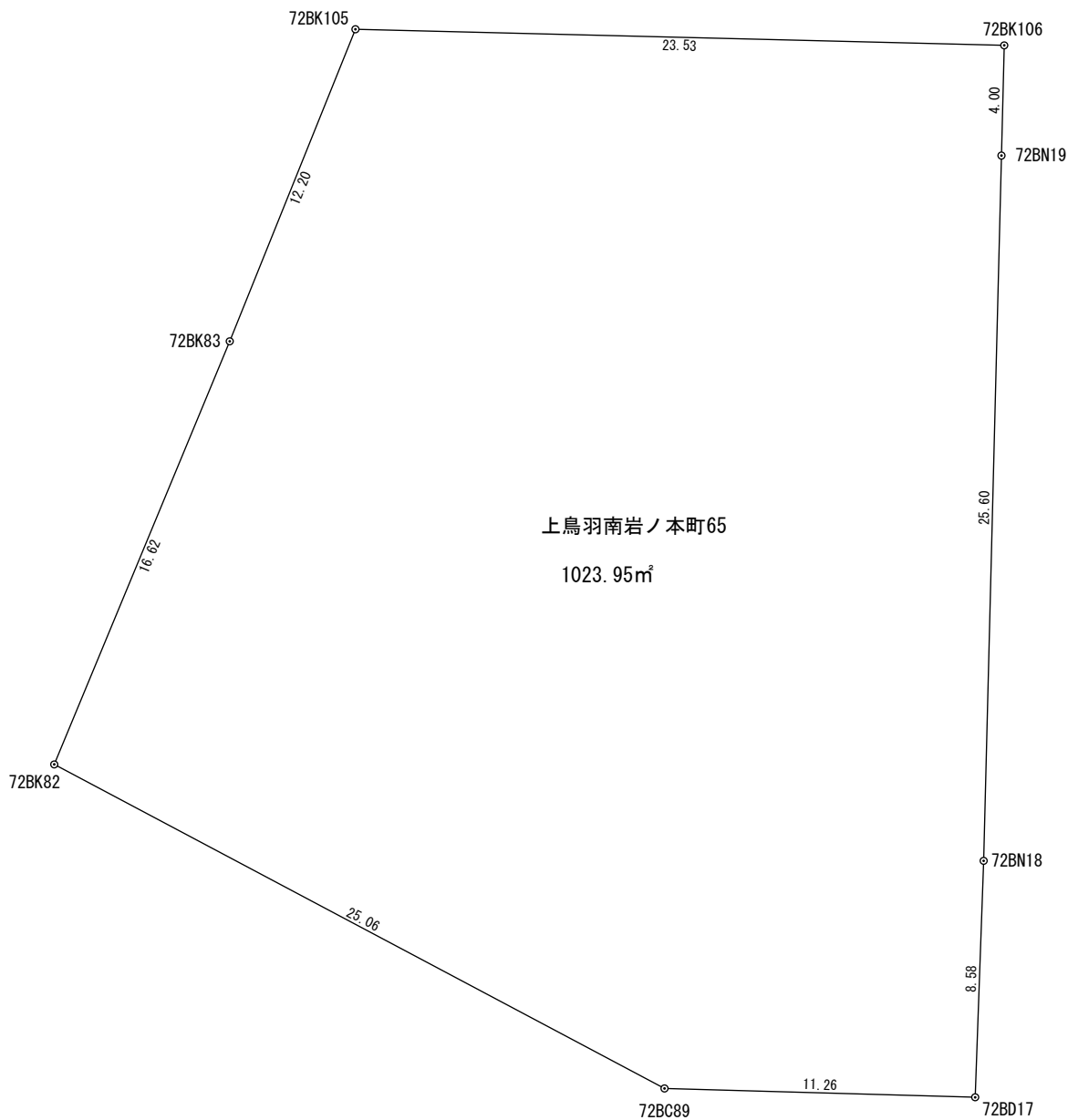
座 標 求 積 表
