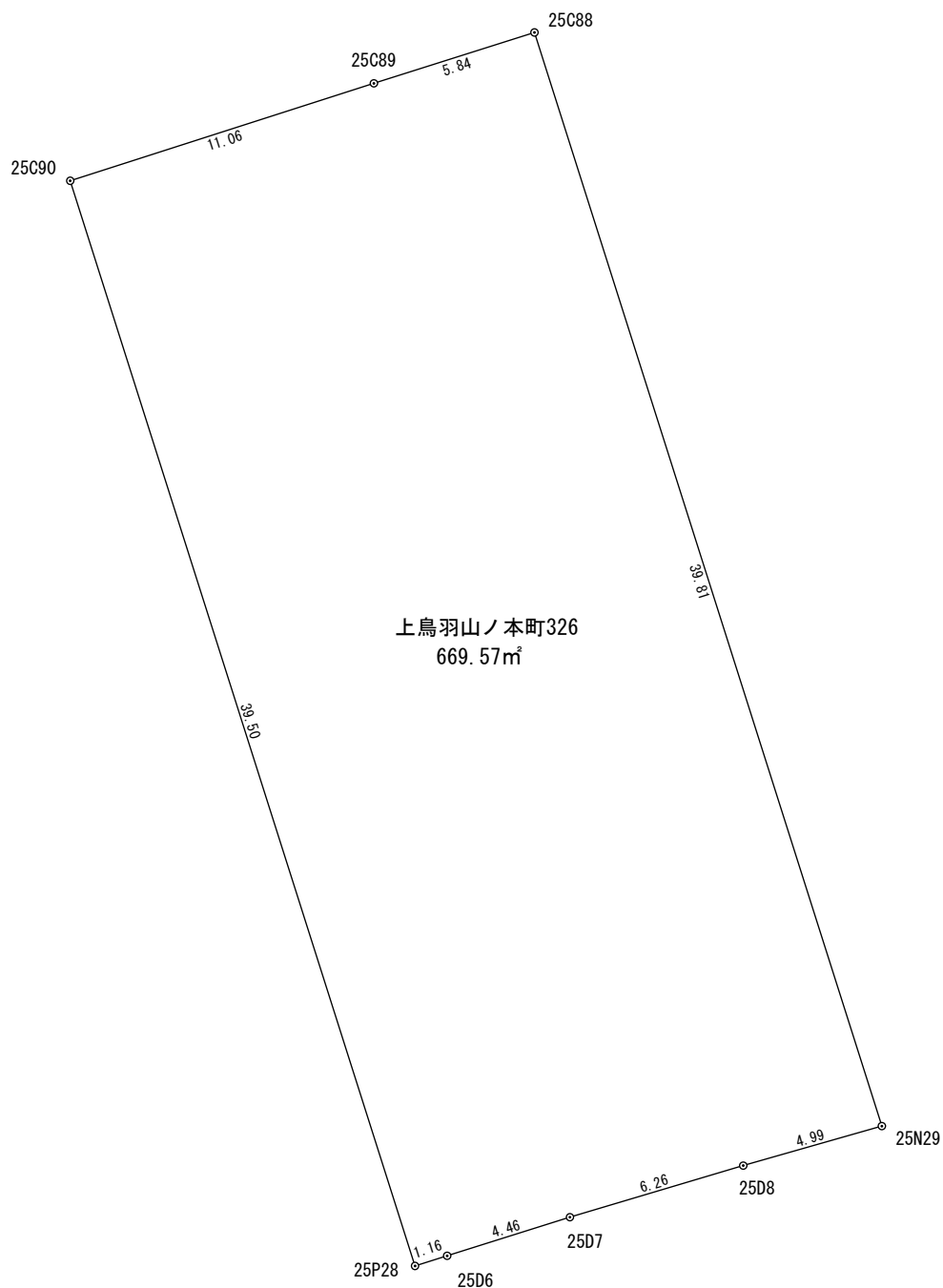
座 標 求 積 表
