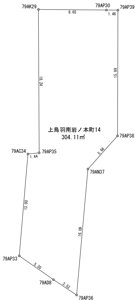
座 標 求 積 表
