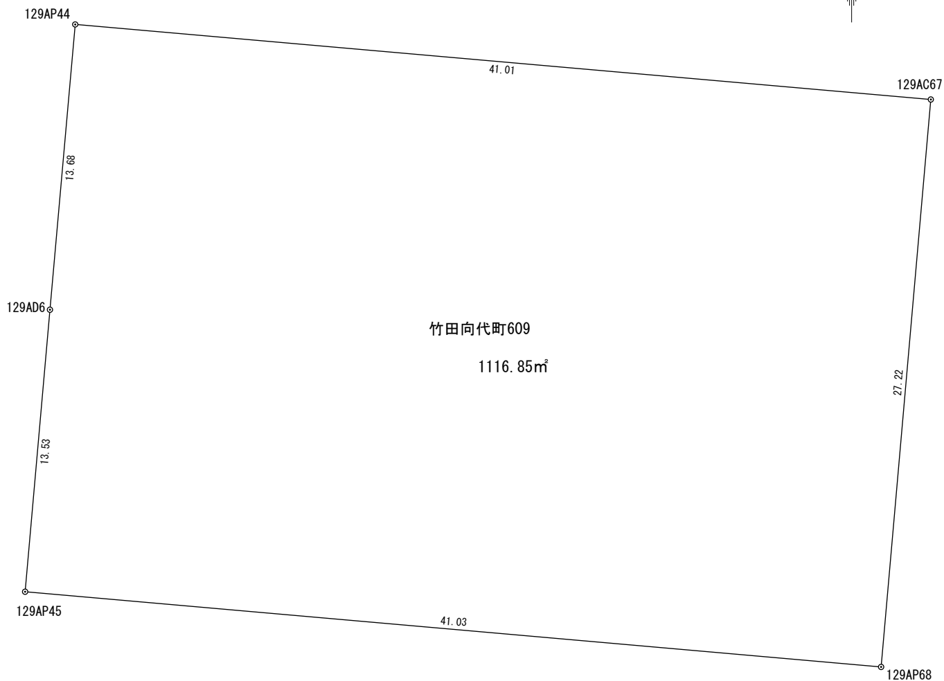
座 標 求 積 表
