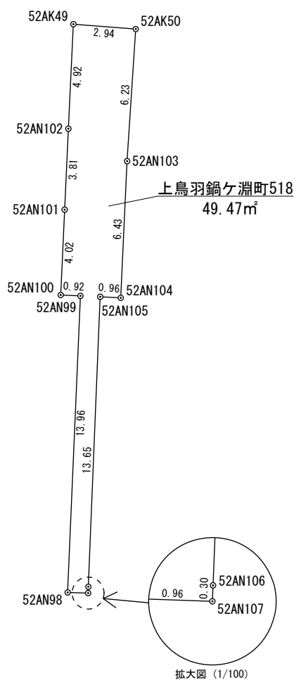
座 標 求 積 表
