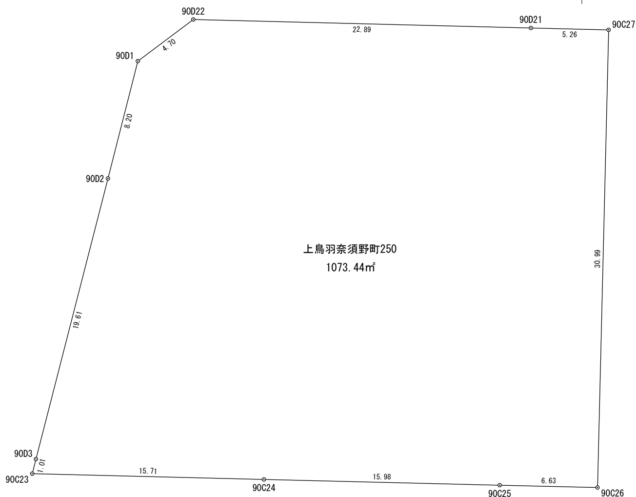
座 標 求 積 表
