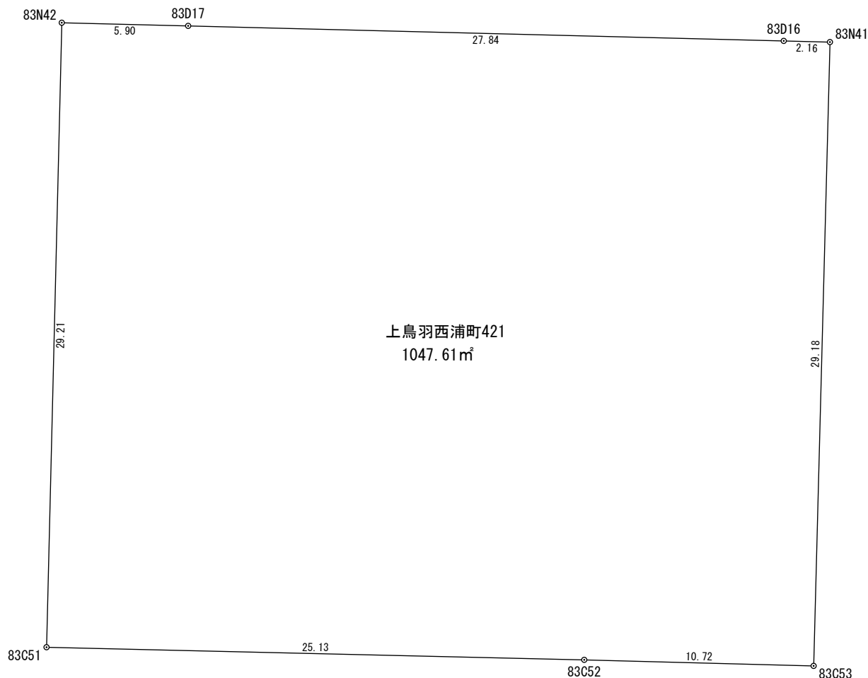
座 標 求 積 表
