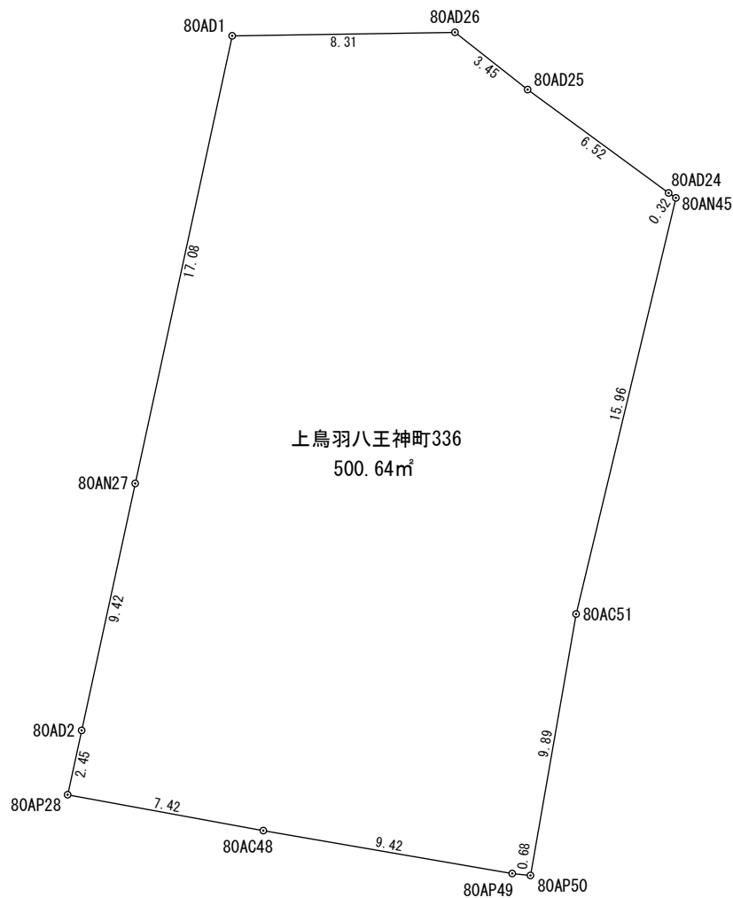
座 標 求 積 表
