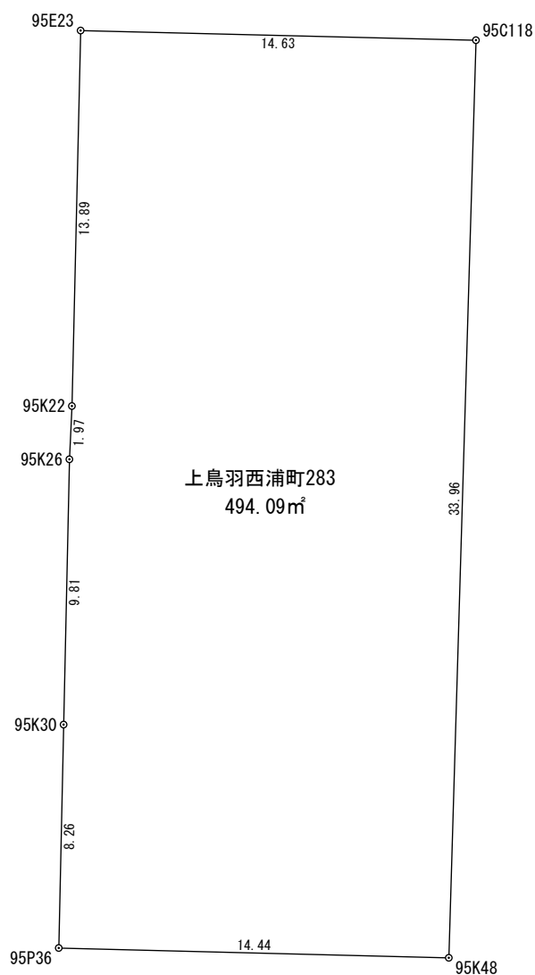
座 標 求 積 表
