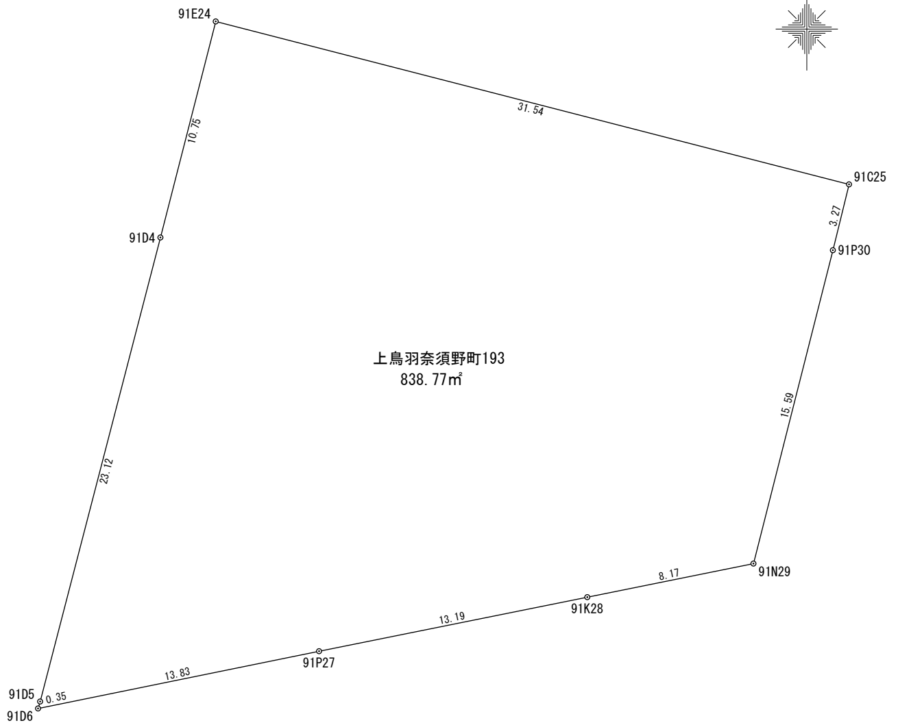
座 標 求 積 表
