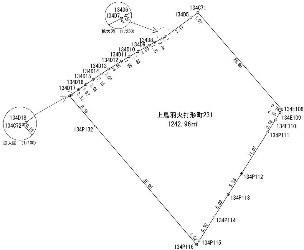
座 標 求 積 表
