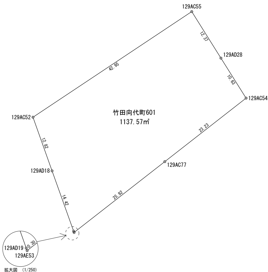
座 標 求 積 表
