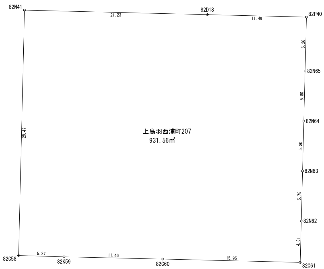
座 標 求 積 表
