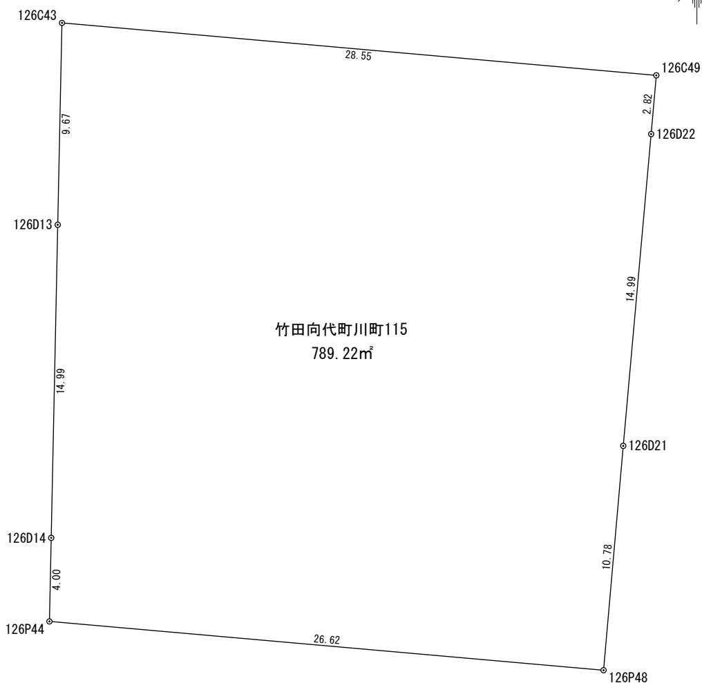
座 標 求 積 表
