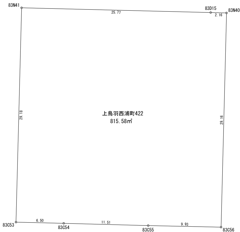
座 標 求 積 表
