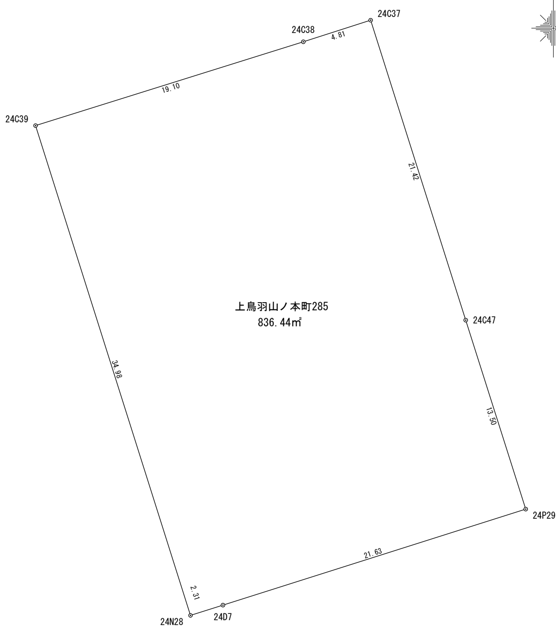
座 標 求 積 表
