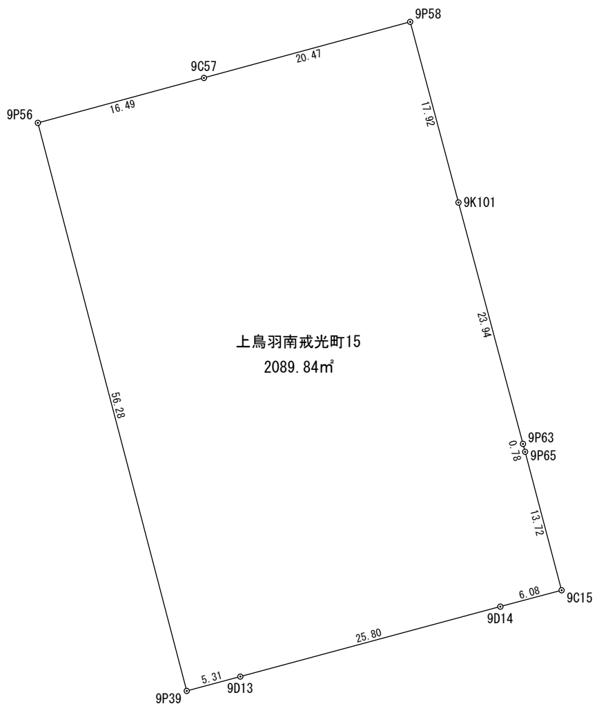
座 標 求 積 表
