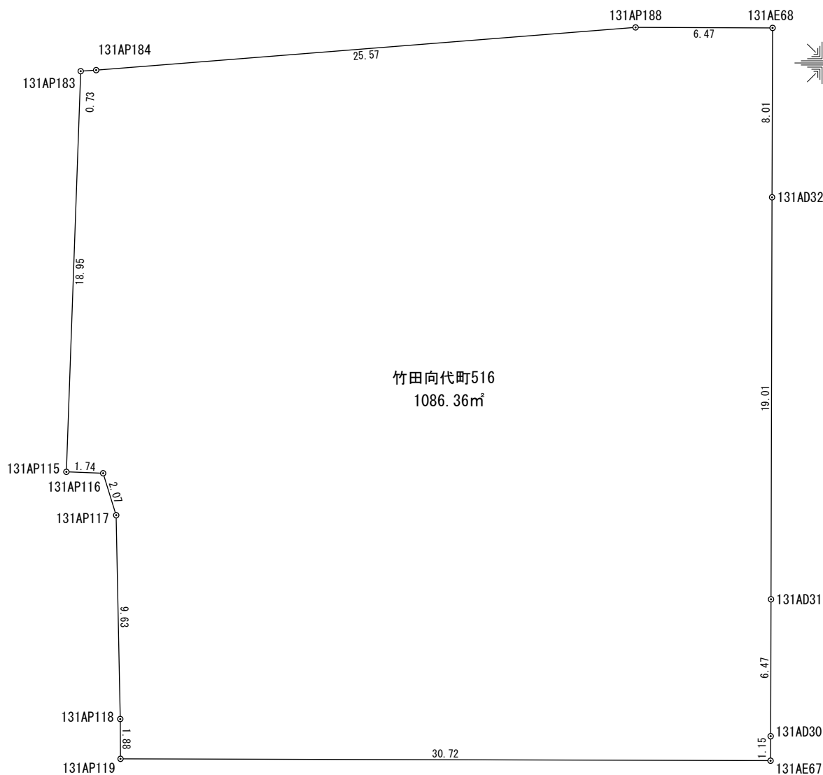
座 標 求 積 表
