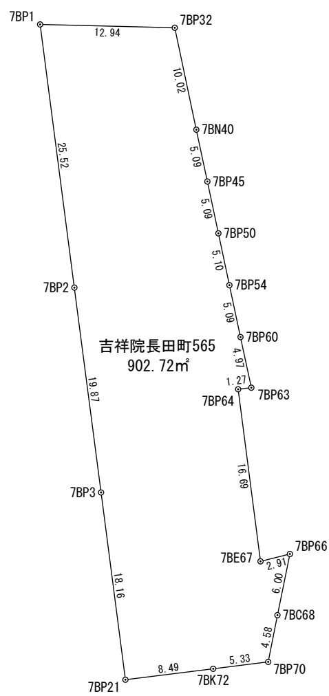
座 標 求 積 表
