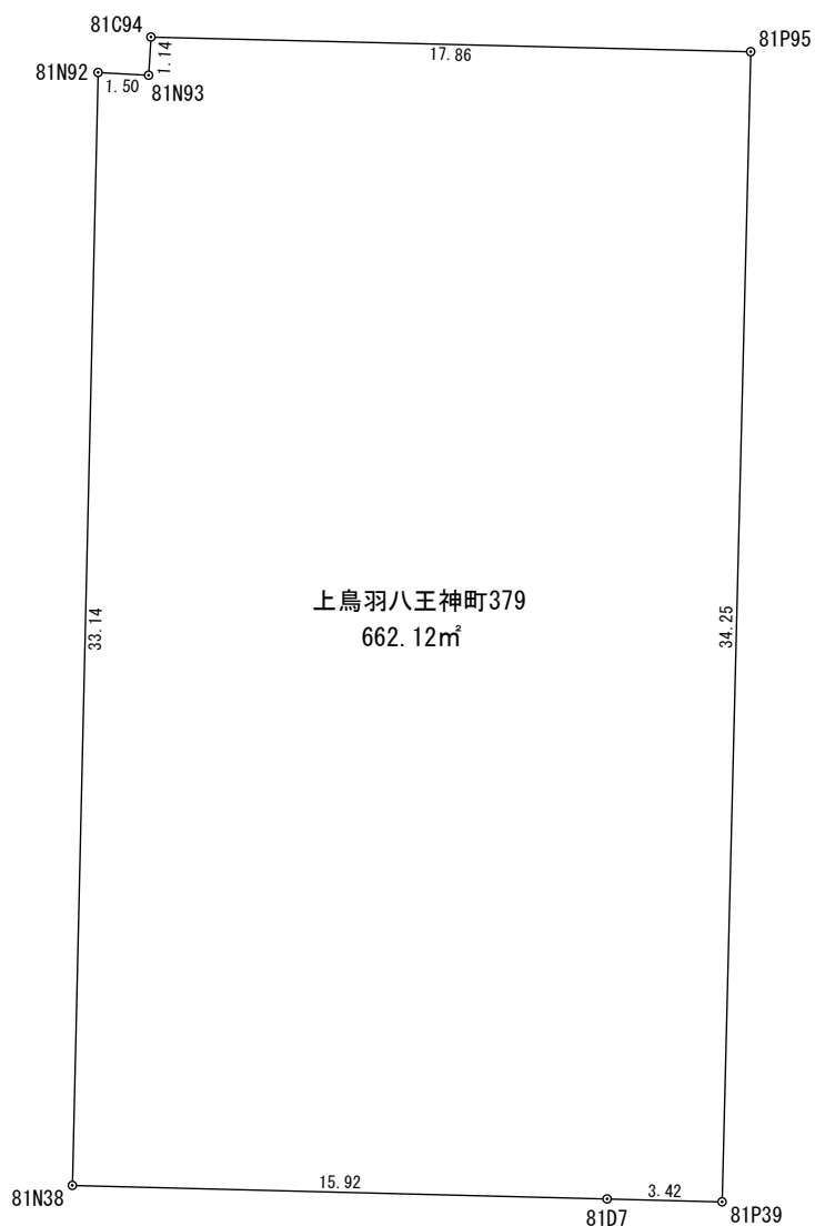
座 標 求 積 表
