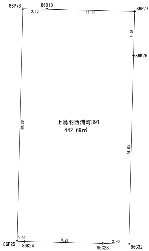
座 標 求 積 表
