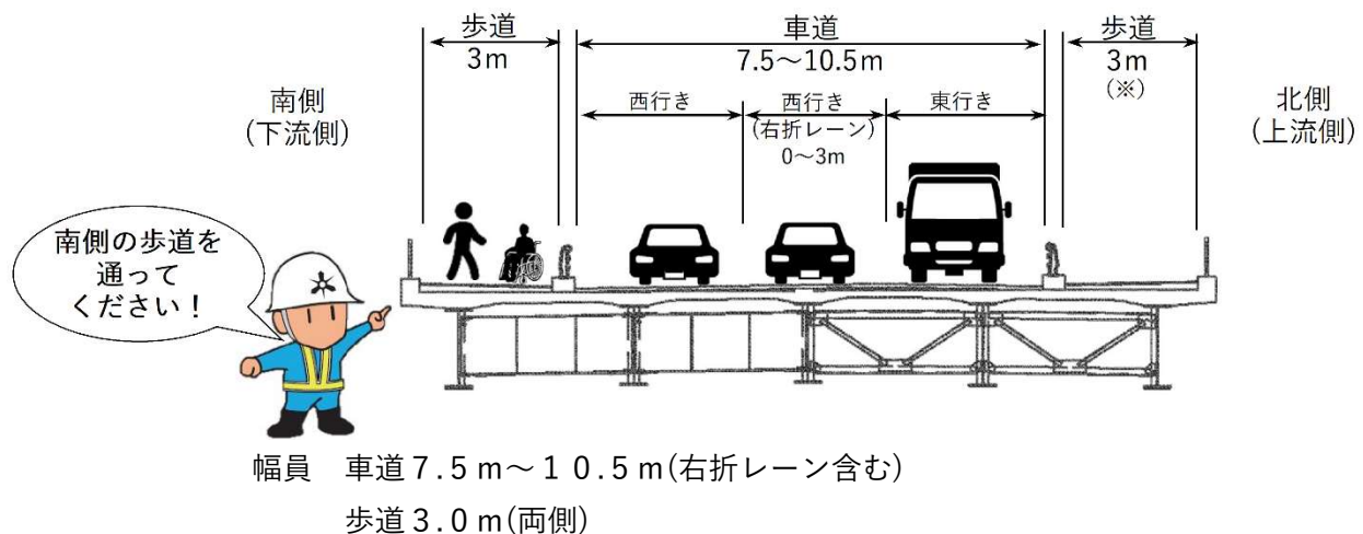
【断面図】
