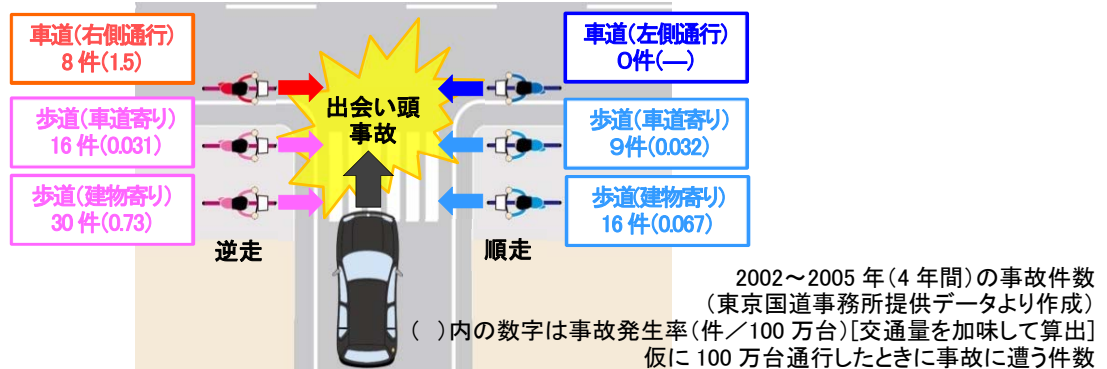
図 3.20 幹線道路と細街路との交差点における自転車と自動車との出会い頭事故の発生状況
