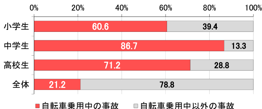
図 3.27 小中高生の交通事故の内訳
