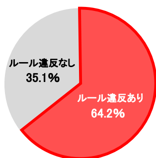
図 3.28 自転車乗用者（第1・2当事者）の法令違反別死傷者割合（2011年）
