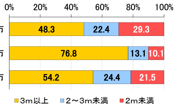
図 3.11 歩道(自転車歩行者道を含む。)幅員別割合
