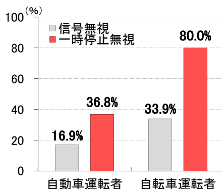
図 3.29 信号無視率、一時停止無視率の数値（各無視の件数／自転車事故の件数）（1993～2001年）
