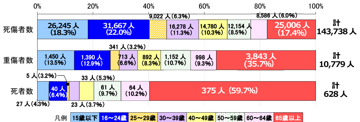
図 3.25 平成 23 年自転車乗用中の年齢層別死傷者数、重傷者数及び死者数
