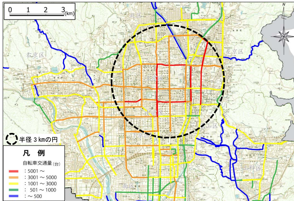
図 3.8 自転車交通量図（昼間 12 時間）
