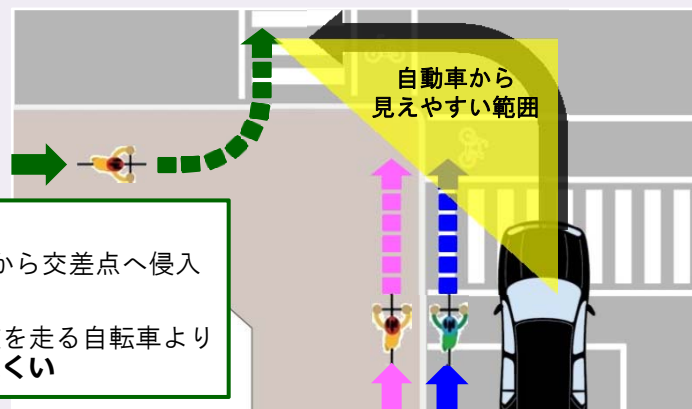
図 5.4 幹線道路交差点の整備の留意点
