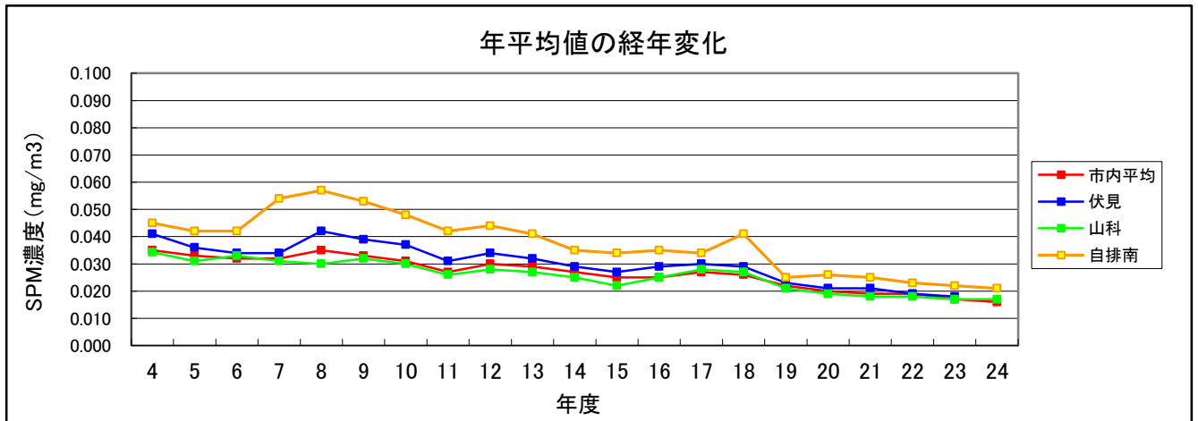
・一般大気測定局における浮遊粒子状物質 (SPM) の測定結果 (年平均値) (単位: mg/m 3 )
