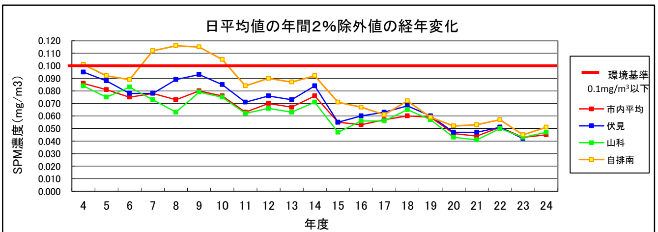
・一般大気測定局における浮遊粒子状物質 (SPM) の測定結果 (日平均値の年間2%除外値) (単位: mg/m 3 )
