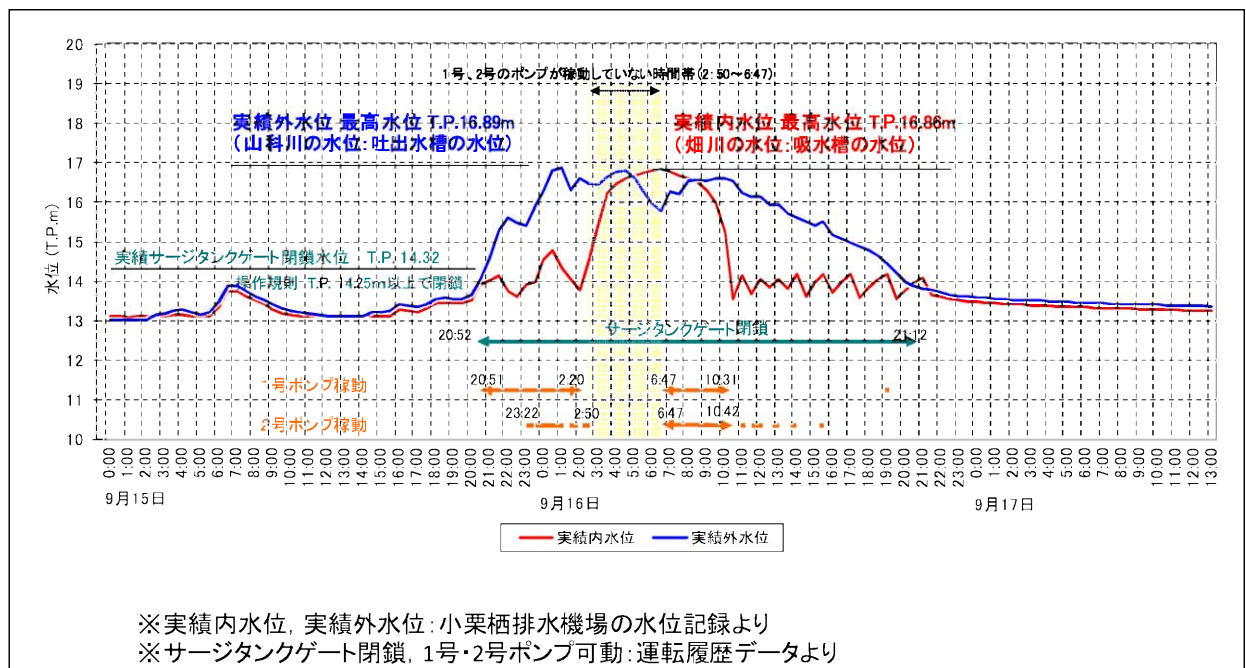
図 6-2-1 観測水位及び排水機場の運転状況
