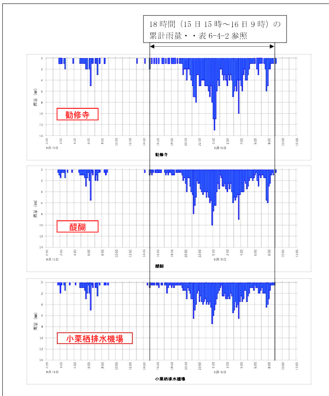
図 6-4-5 小栗栖排水機場，醍醐，勧修寺各雨量観測所の雨量相関図
