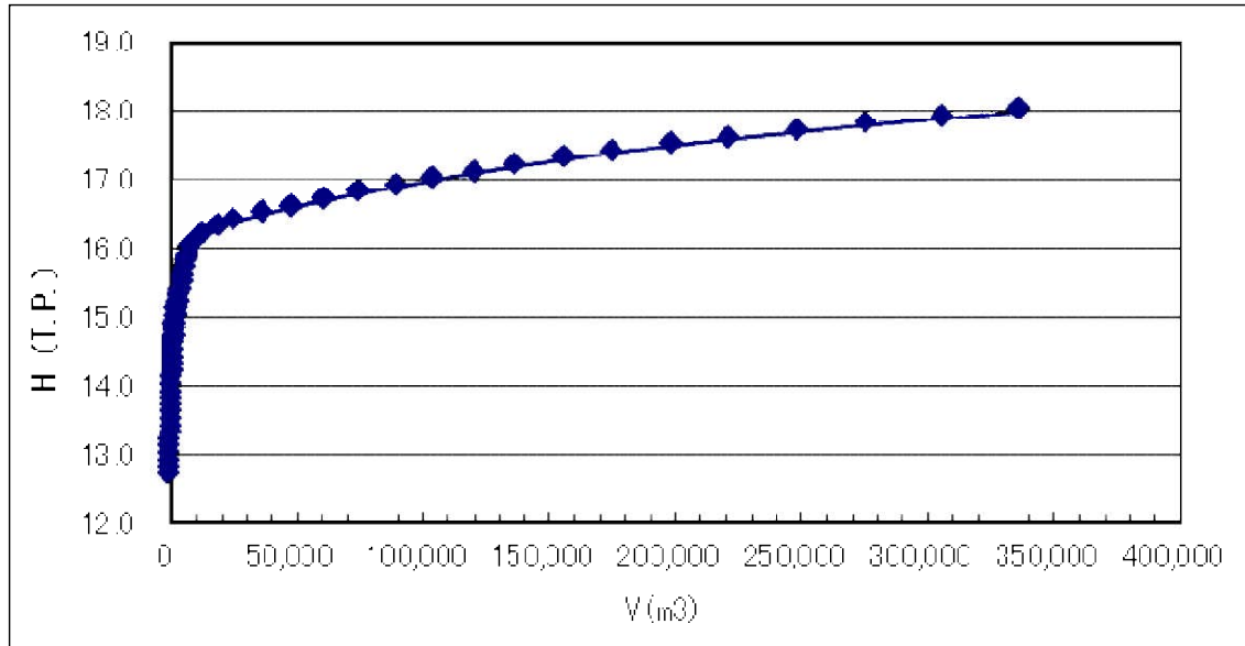
図 6-4-9 H-V 曲線図
