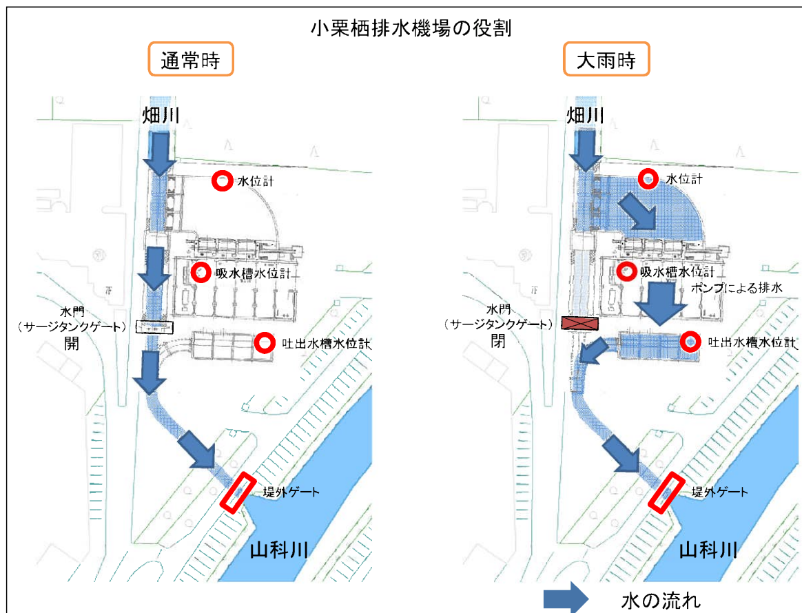
図 5-2-1 小栗栖排水機場の役割
