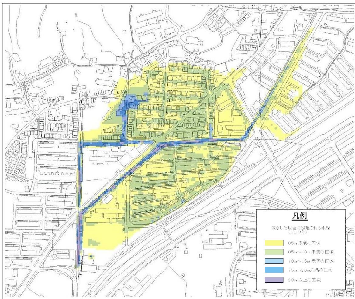
図 6-4-11 浸水予測コンター図 (ポンプが実績稼働したケース)
