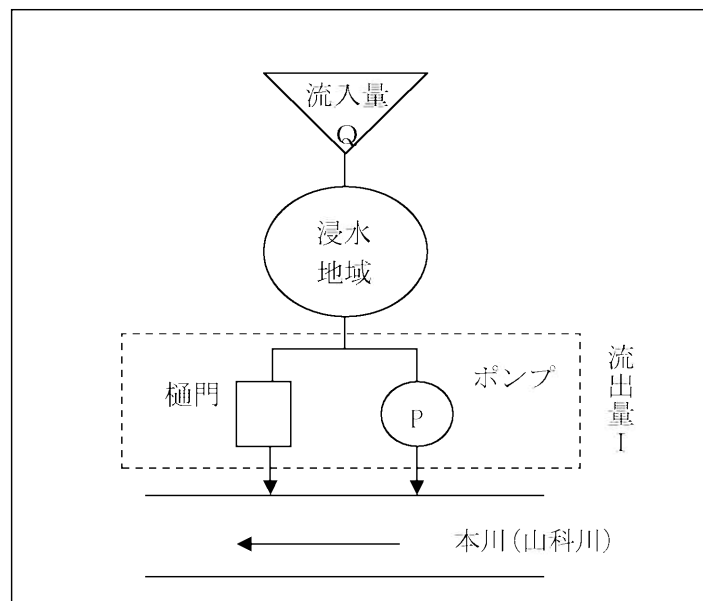
図 6-4-1 内水モデル (1 池モデル)
