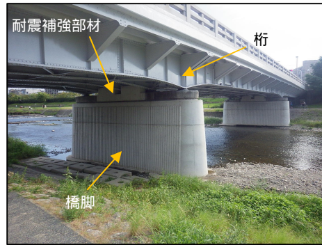
「老朽化修繕」 二条大橋 二条通にある鴨川に架かる橋りょう
