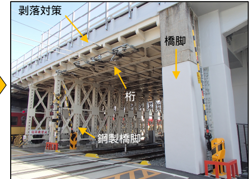
「耐震補強」 九条跨線橋 九条通にあるJR奈良線・京阪本線・鴨川を跨ぐ橋りょう
