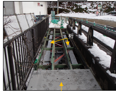
新しい床版
