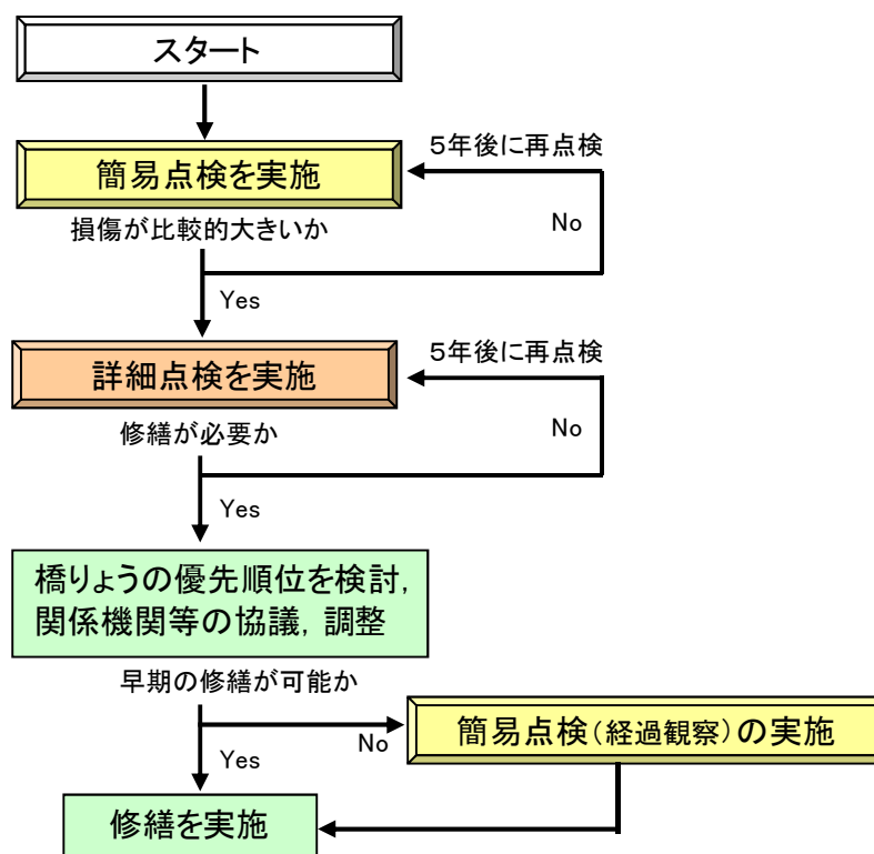
図 4.1 橋りょう点検の基本的な考え方
