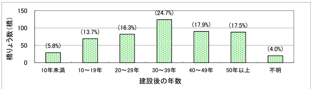
図 1.3 建設年別橋長 15m 以上の橋りょう数
