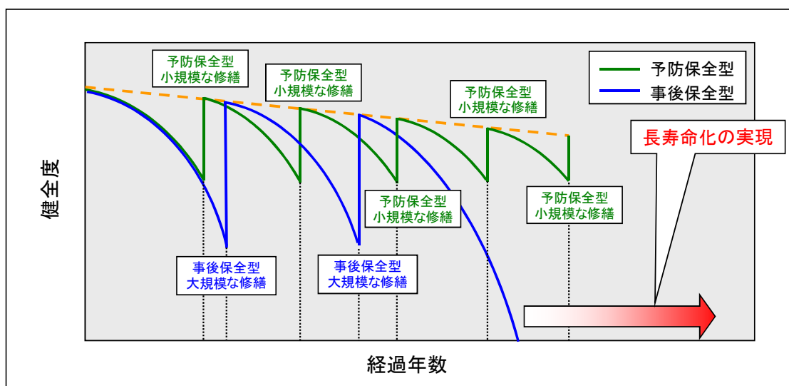
図 5.2 経過年数と健全度(鋼橋の場合)
