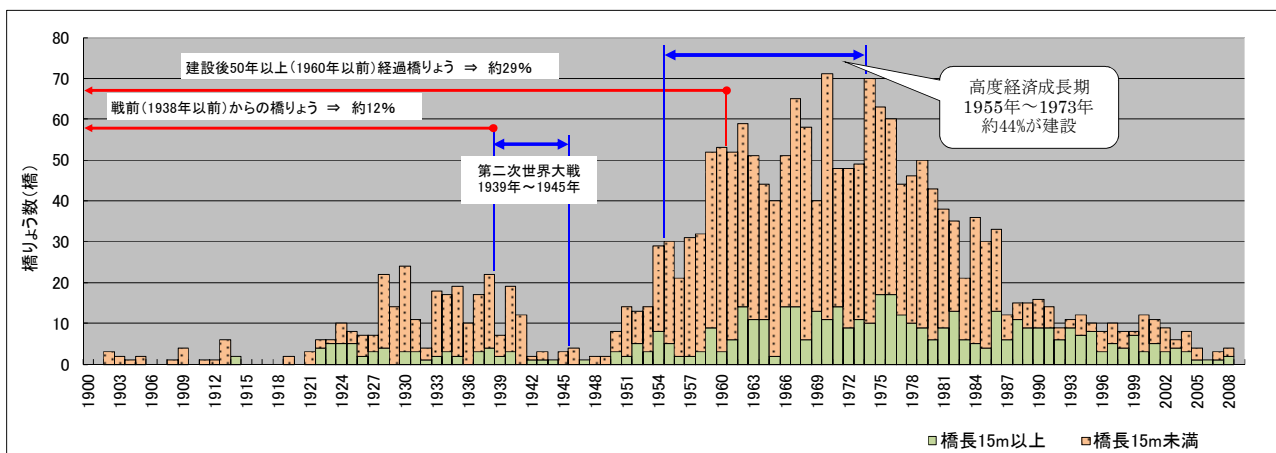
図 1.1 建設年別橋りょう数
