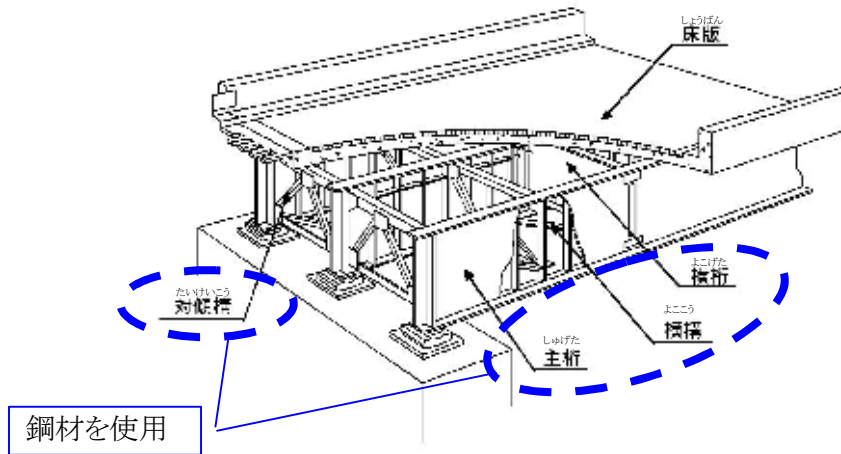
図 8.1 鋼橋の構造
