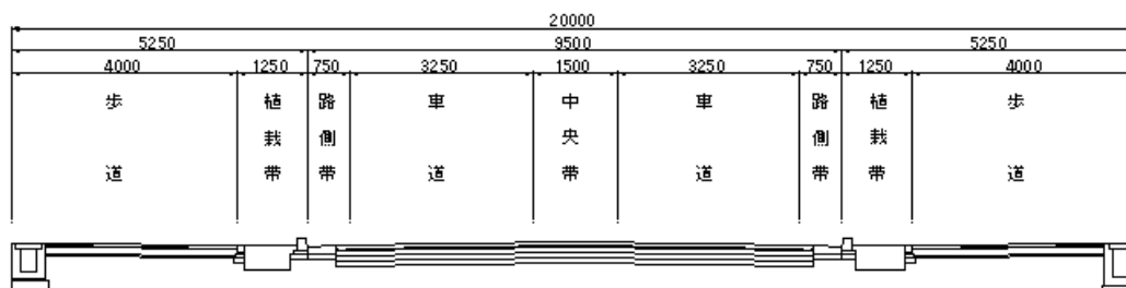
標準断面図 一般部
