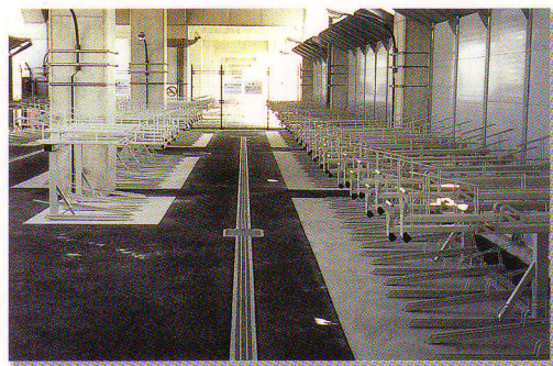
機械式2段ラック
