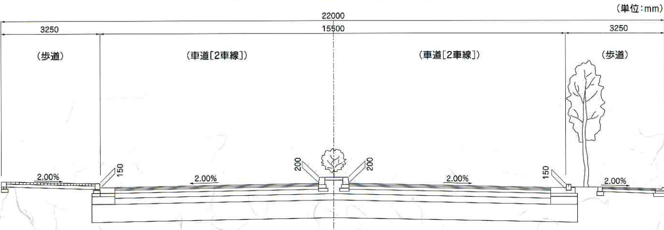
標準断面図
