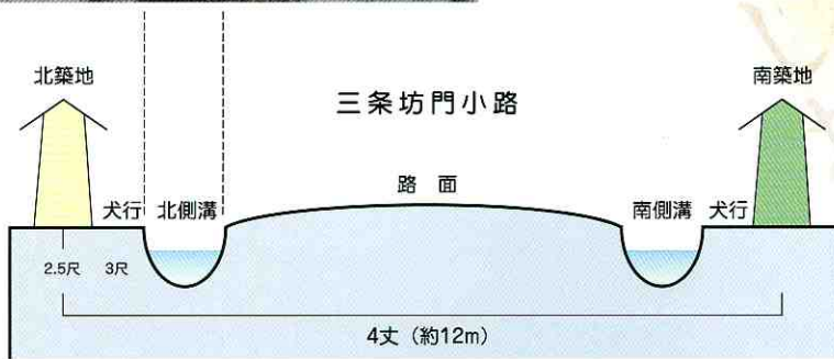
横断面図
