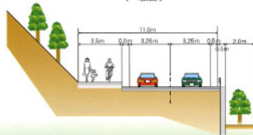
標準横断面図 （一般部）
