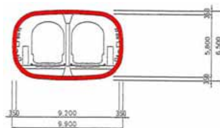
西大路駅～天神川駅・複断面シールド部
