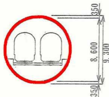
西大路～天神川駅 大型円形複線シールド工法
