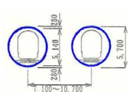
二条～西大路駅 単線シールド工法
