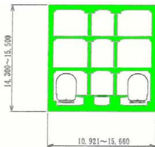
天神川駅工区断面図
