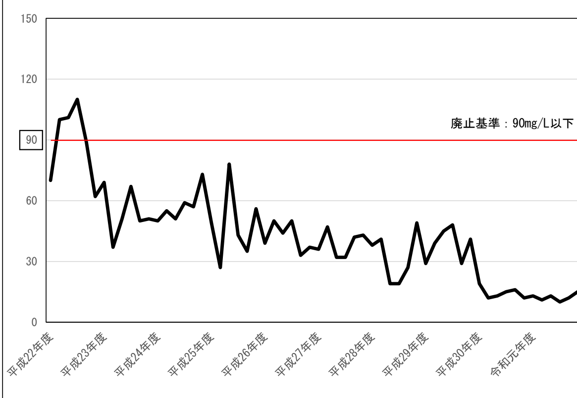
化学的酸素要求量 (COD) の推移【mg/L】
