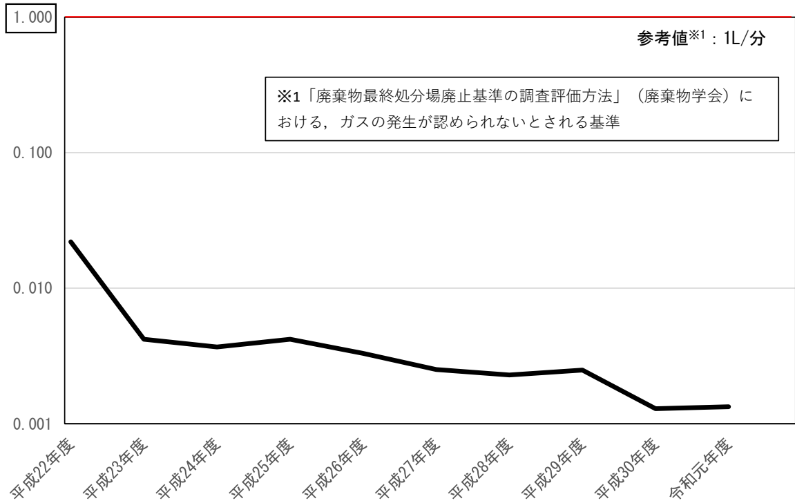
発生ガス量の推移【L/分】
