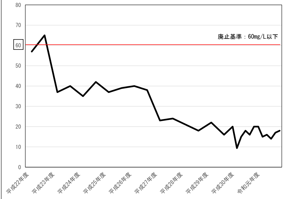
窒素含有量の推移【mg/L】
