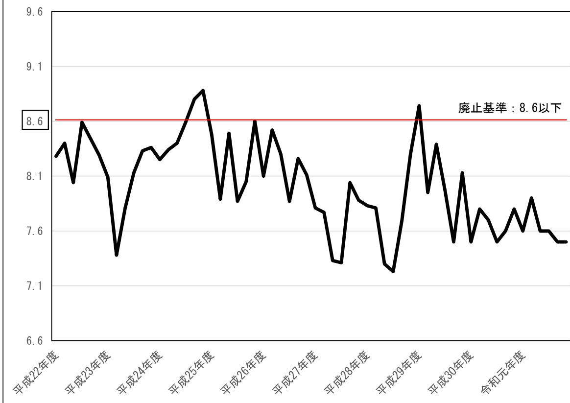
水素イオン濃度 (pH) の推移
