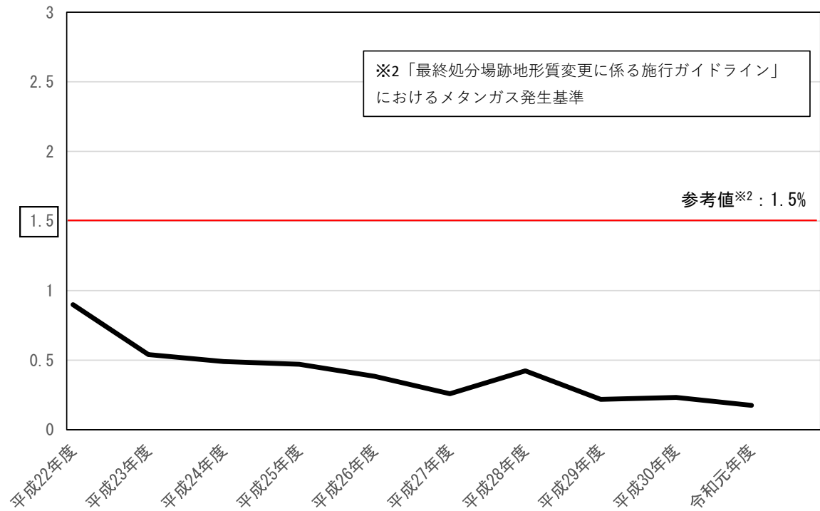
メタンガス濃度の推移【%】
