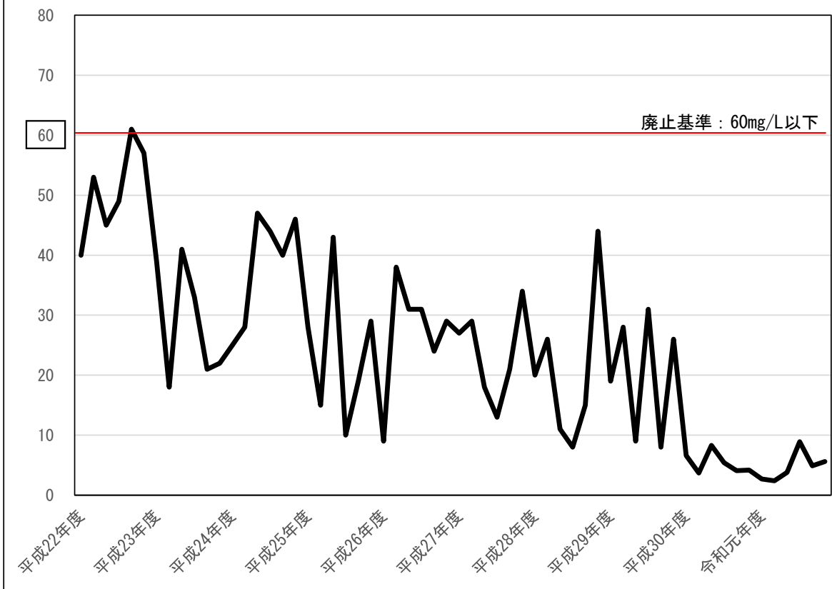
生物化学的酸素要求量 (BOD) の推移【mg/L】
