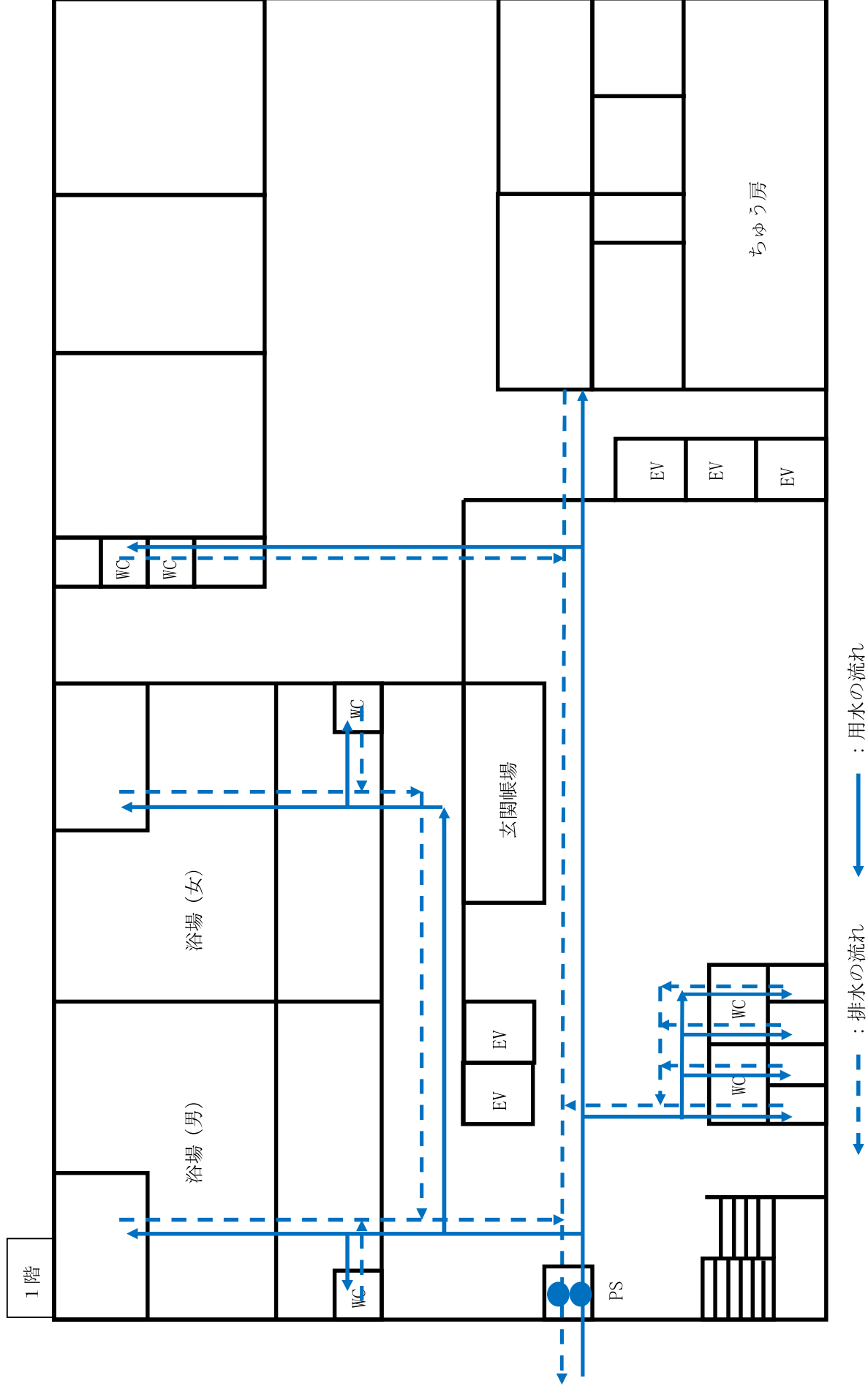
【各階平面図及び用水及び排水系統図（平面図）】
