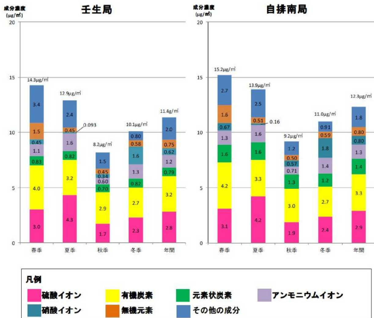
図 1－2 壬生局及び自排南局における PM2.5 の総質量濃度と各成分濃度（平成28年度）
