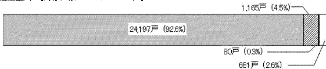
図5-2 地域区分別の環境基準達成状況
