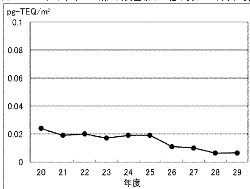
図4-1 ダイオキシン類大気調査結果の経年変化（年間平均値）
