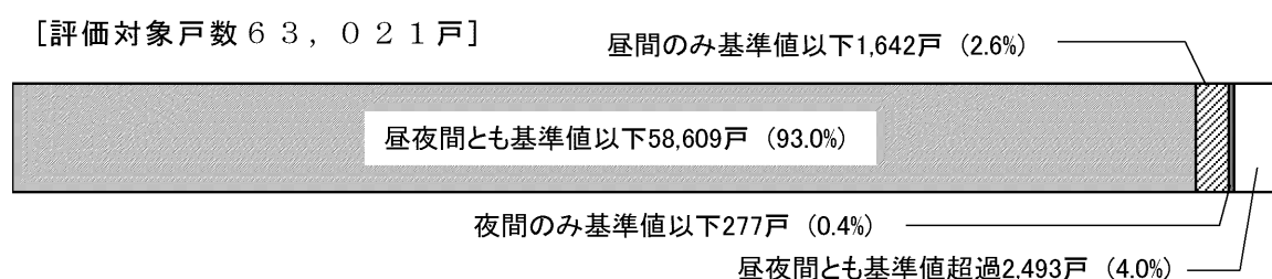
図5－1 環境基準達成状況
