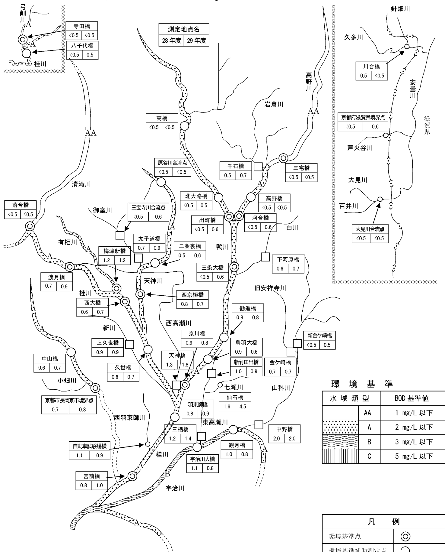
図 2-1 BODの地点別75%水質値 (平成28年度, 平成29年度 単位: mg/L)
