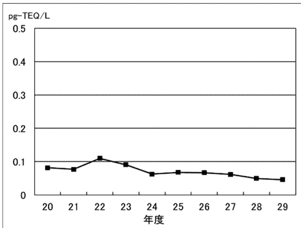
図 4－2 ダイオキシン類河川水質調査結果の経年変化（年間平均値）
