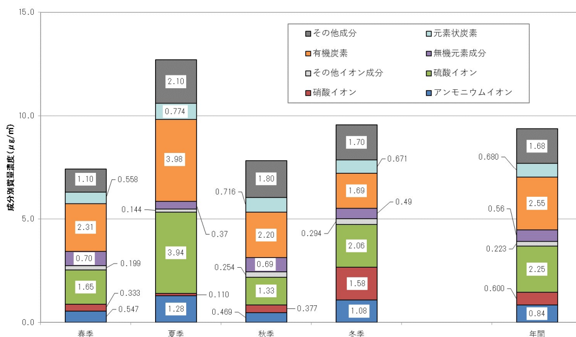
図 1-2 醍醐局におけるPM2.5の総質量濃度と各成分濃度（令和2年度）
