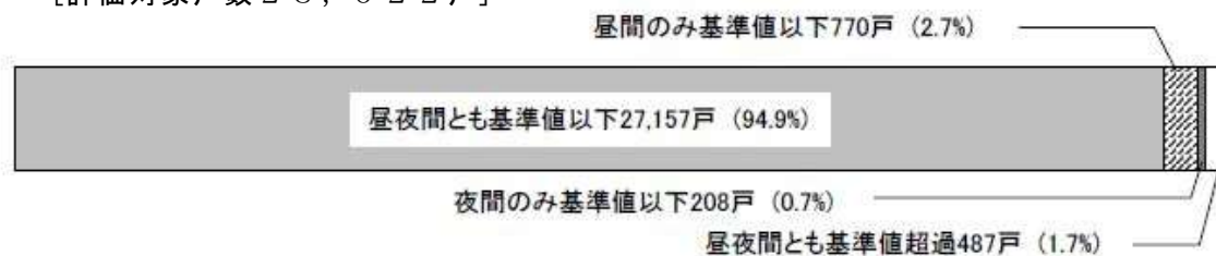
図5-1 環境基準達成状況
