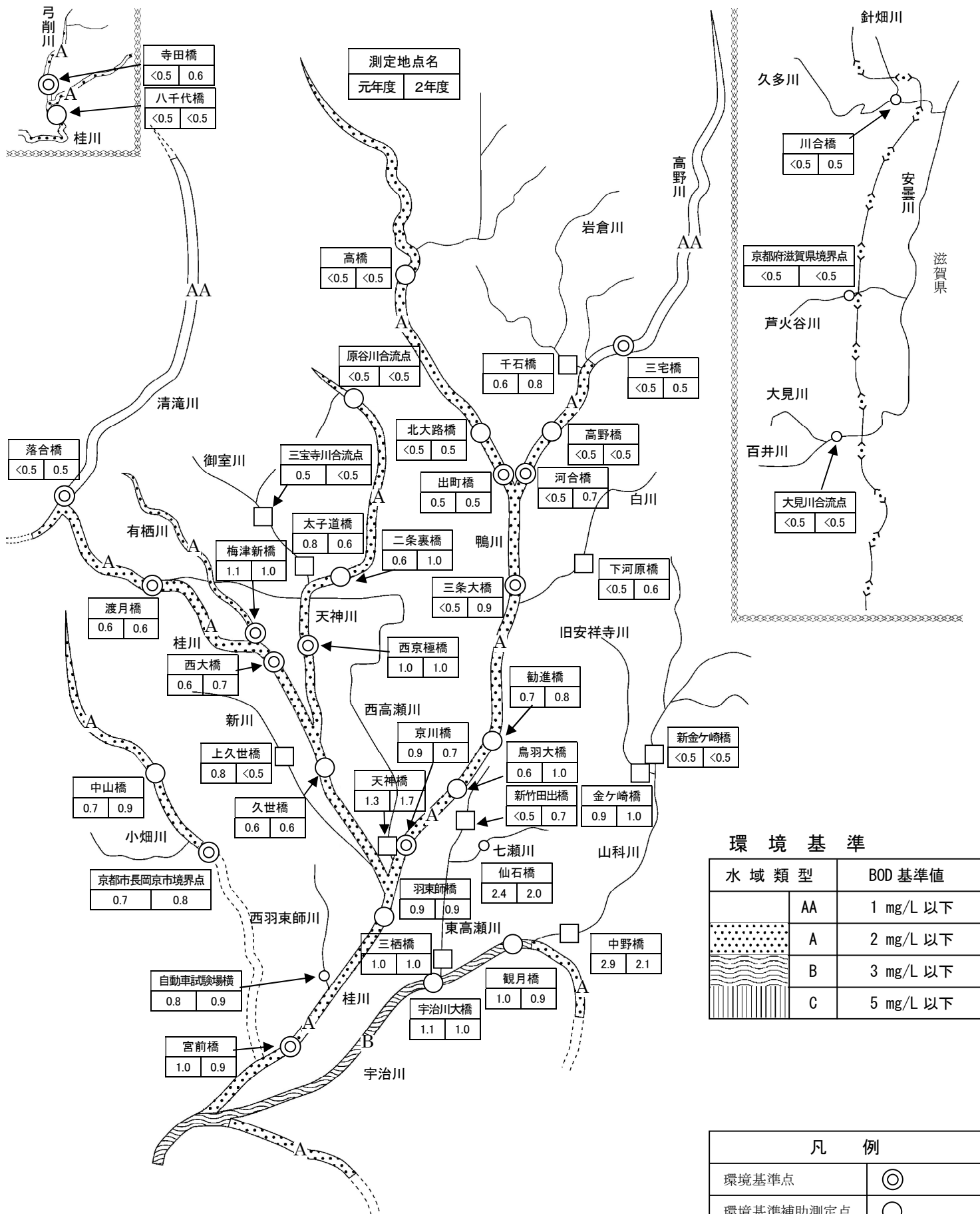
図2-1 BODの地点別75%水質値 (令和元年度, 令和2年度 単位: mg/L)
