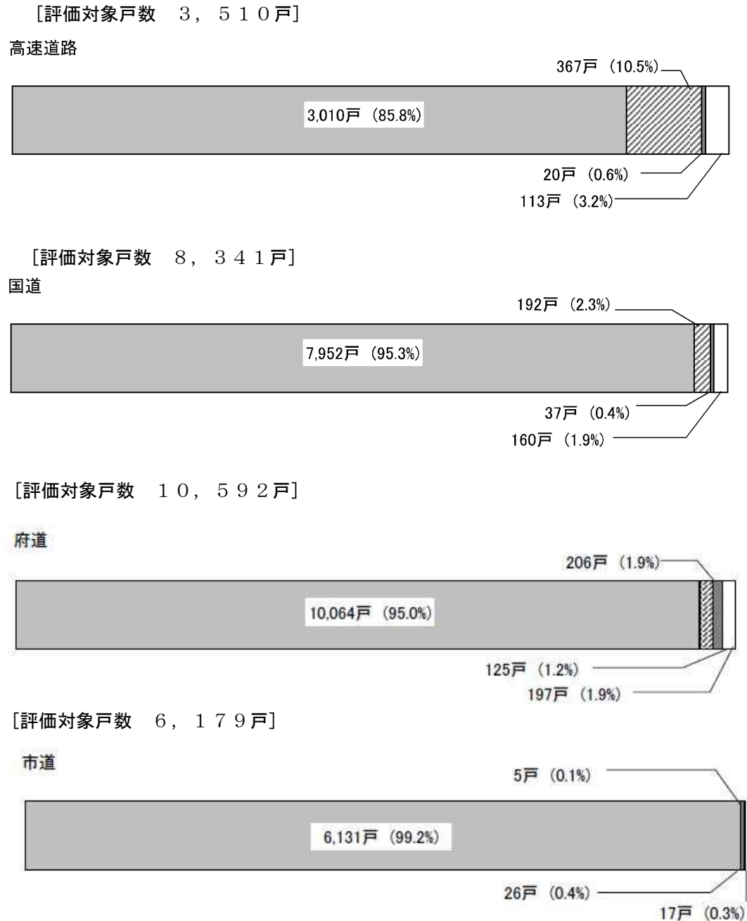
図5-3 道路の種類別の環境基準達成状況
