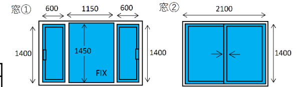
<開口面積>
