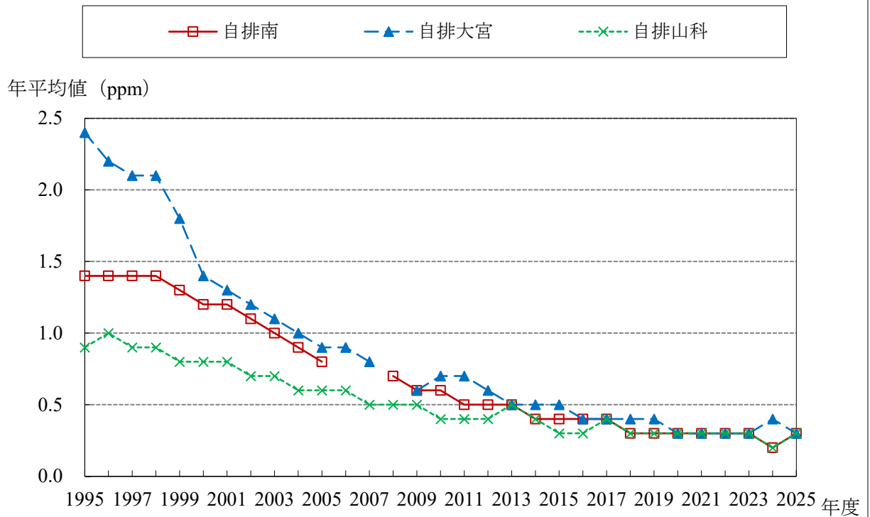
CO 経年変化グラフ (1995～2025年度)
