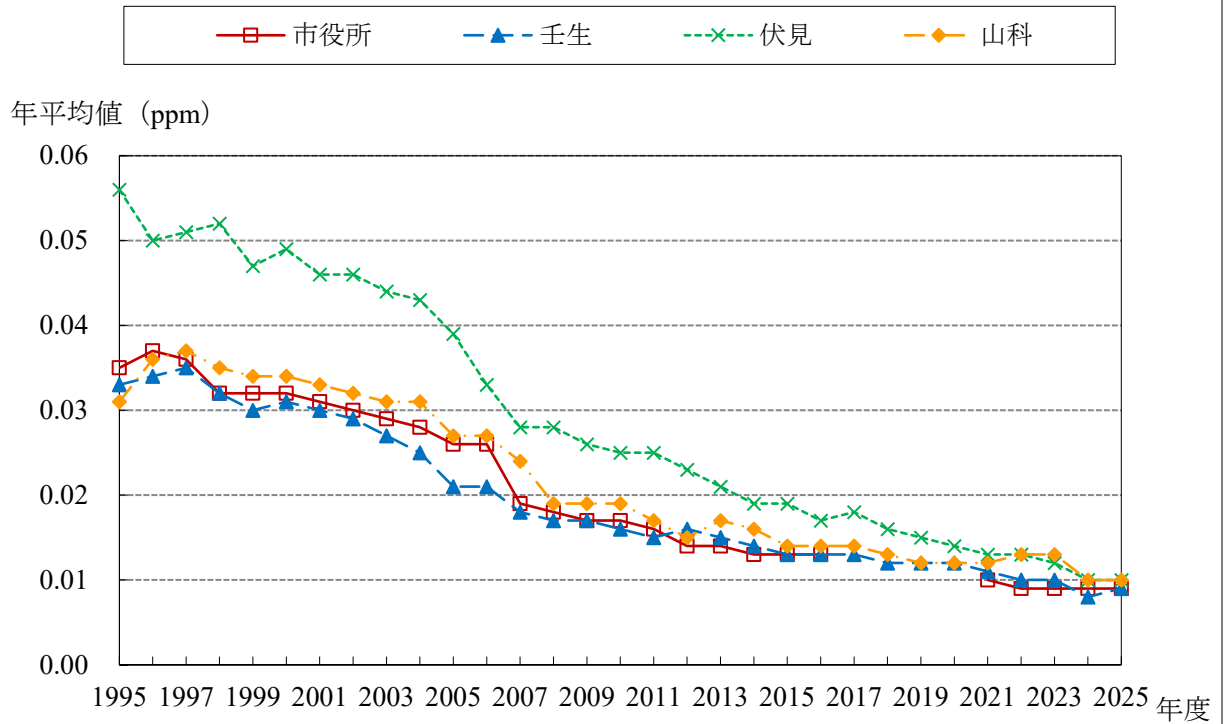
NOx 経年変化グラフ (1995～2025年度)
