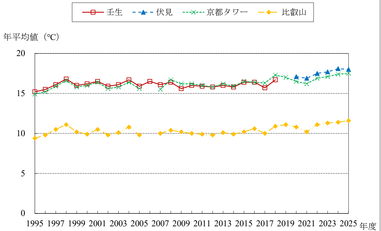
TEMP 経年変化グラフ (1995～2025年度)
