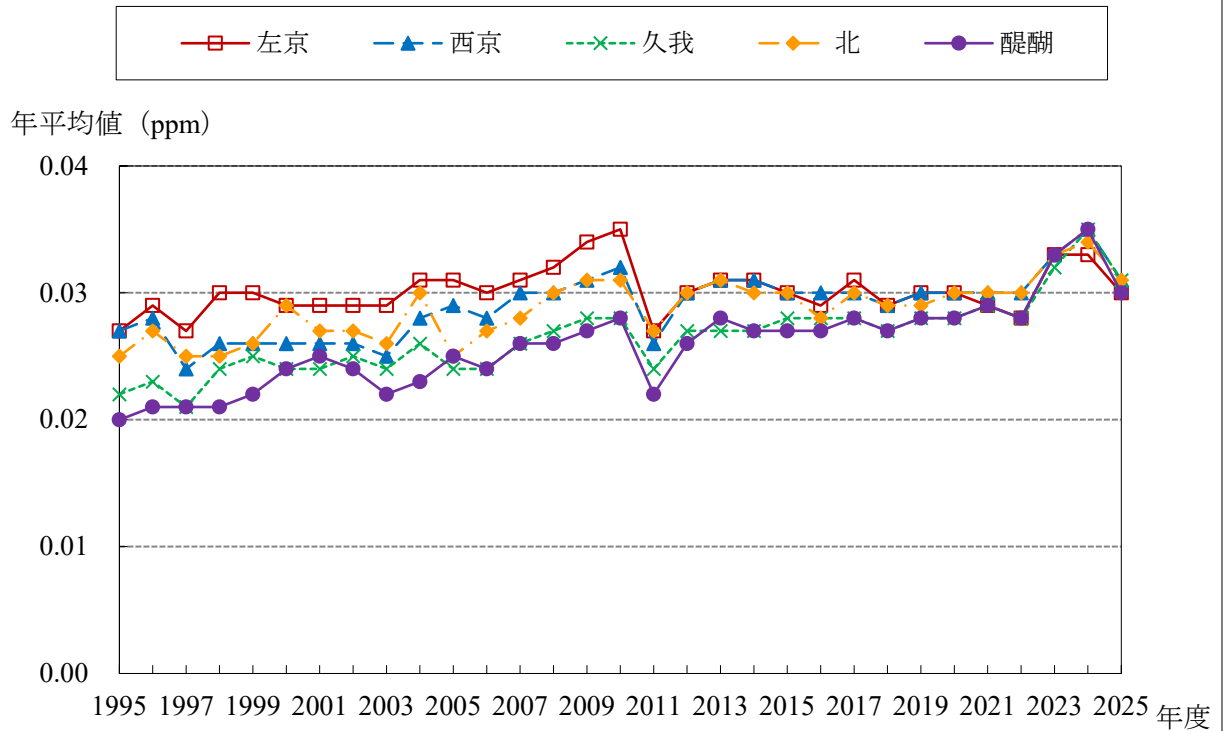
Ox 経年変化グラフ (1995～2025年度)
