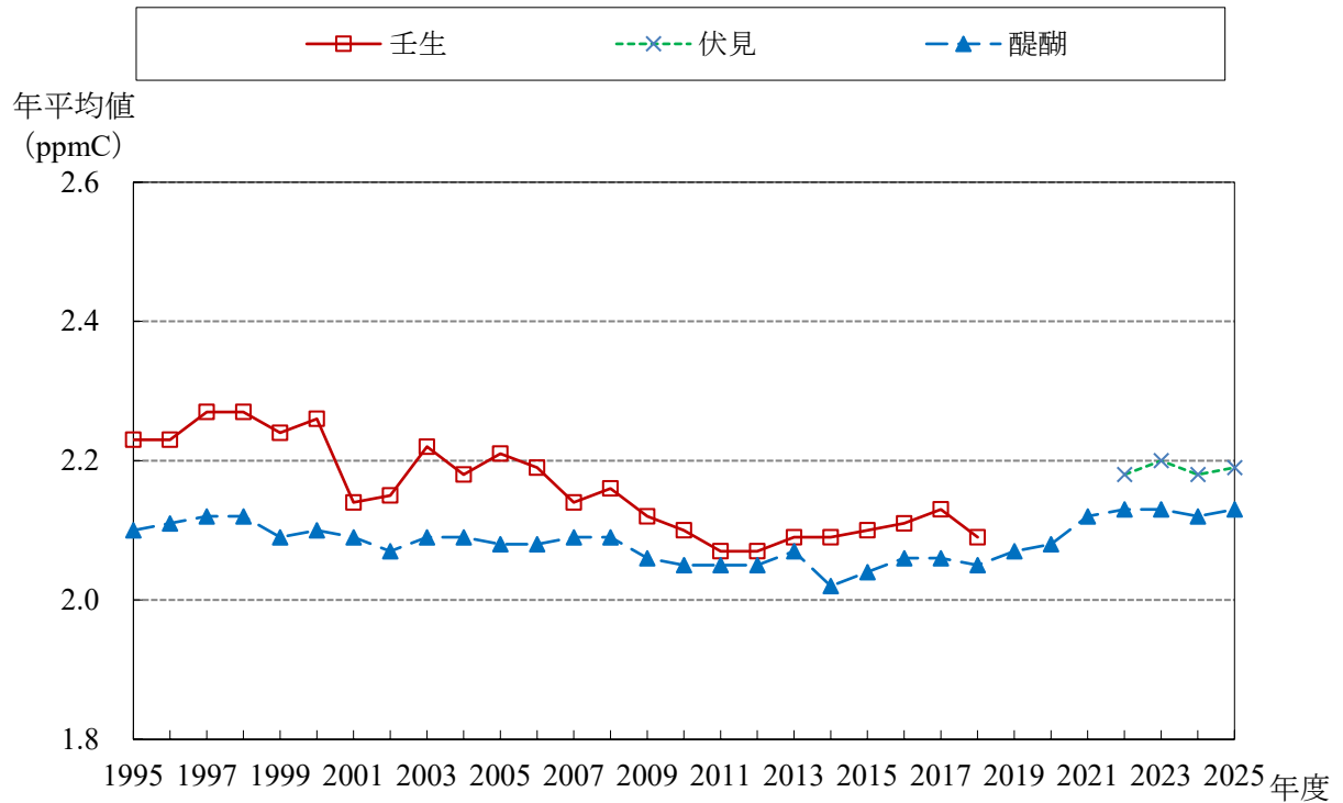
THC 経年変化グラフ (1995 ～ 2025年度)
