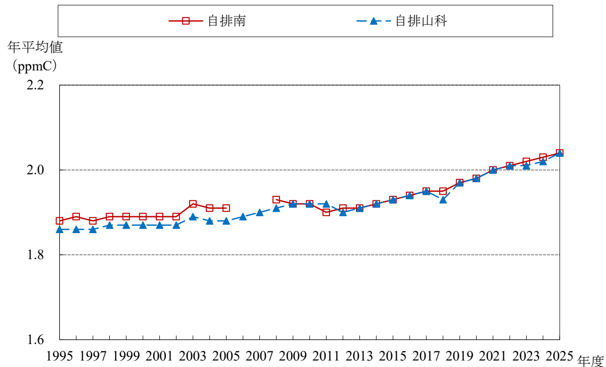
CH 4 経年変化グラフ (1995 ~ 2025年度)
