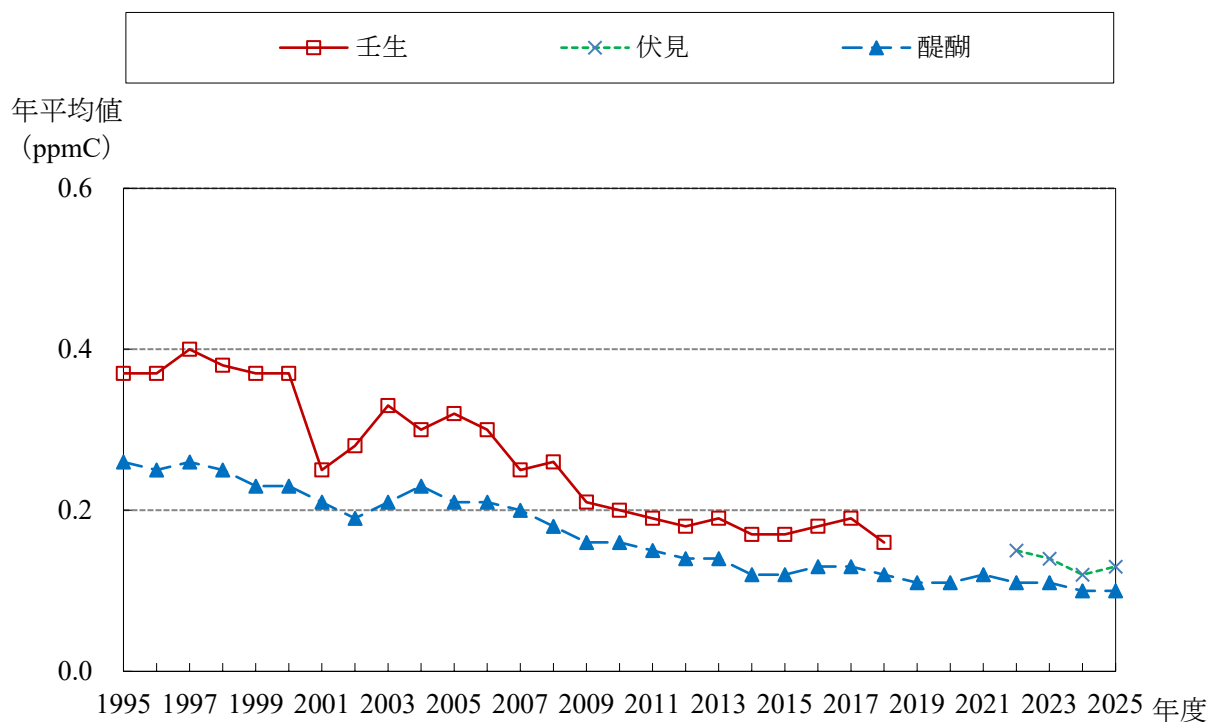
NMHC 経年変化グラフ (1995 ~ 2025年度)
