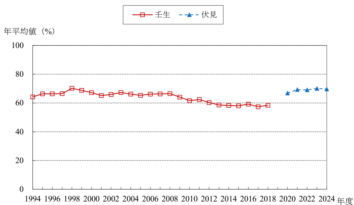
HUM 経年変化グラフ (1994～2024年度)
