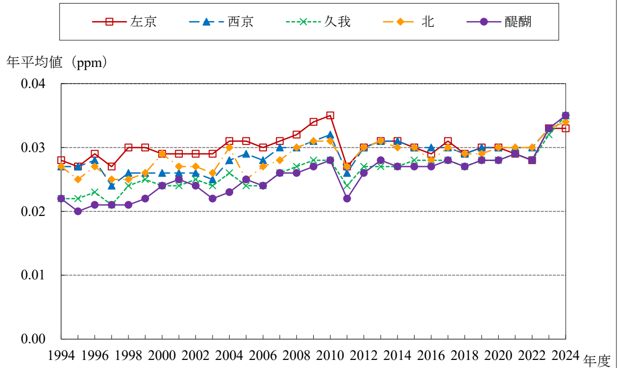
Ox 経年変化グラフ (1994～2024年度)
