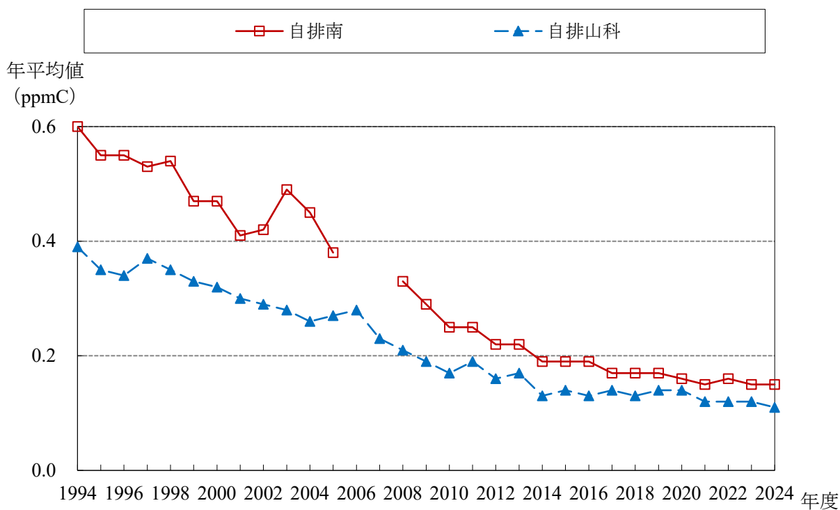
NMHC 経年変化グラフ (1994～2024年度)
