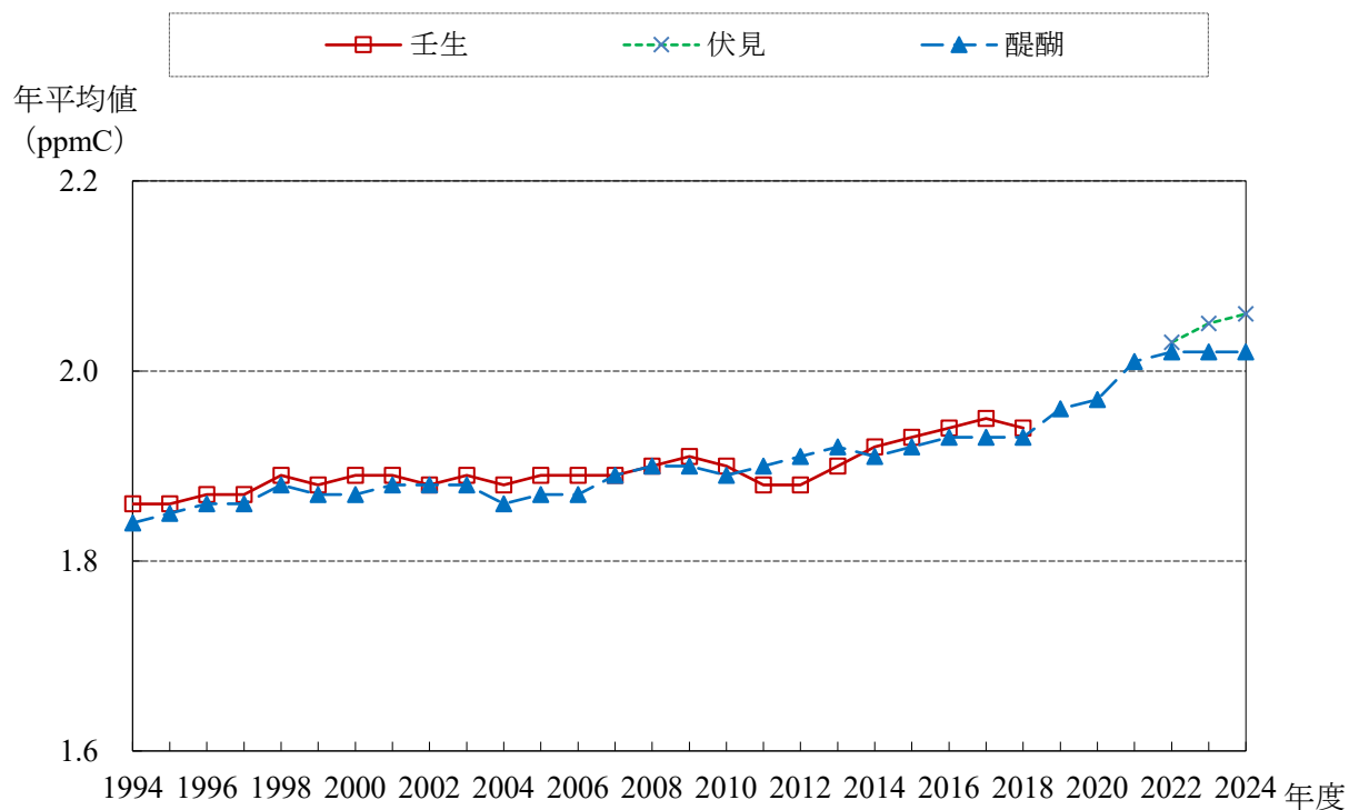
CH 4 経年変化グラフ (1994～2024年度)
