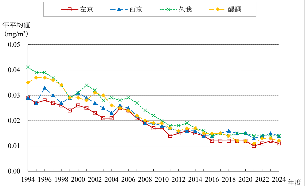
SPM 経年変化グラフ (1994～2024年度)
