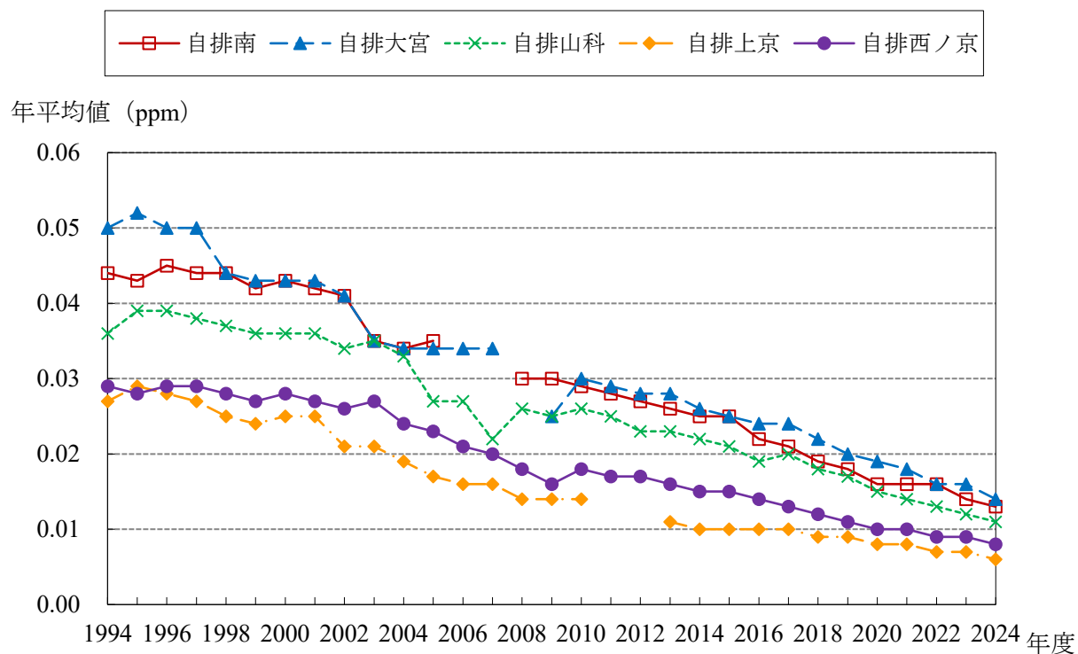
NO 2 経年変化グラフ (1994～2024年度)
