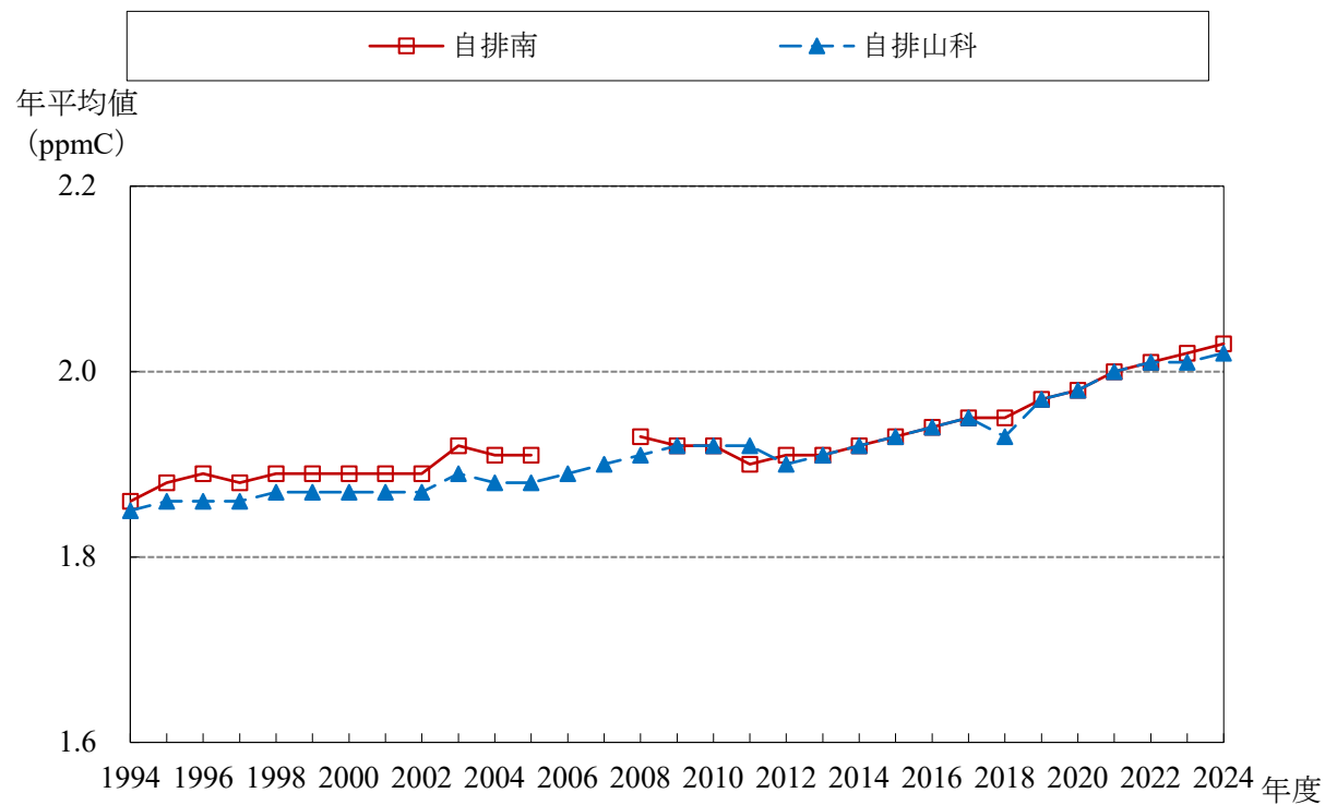
CH 4 経年変化グラフ (1994～2024年度)
