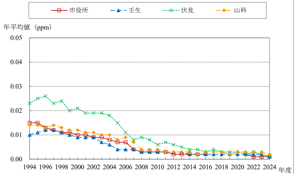
NO 経年変化グラフ (1994～2024年度)
