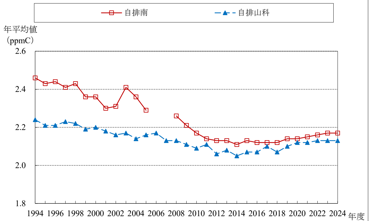
THC 経年変化グラフ (1994～2024年度)
