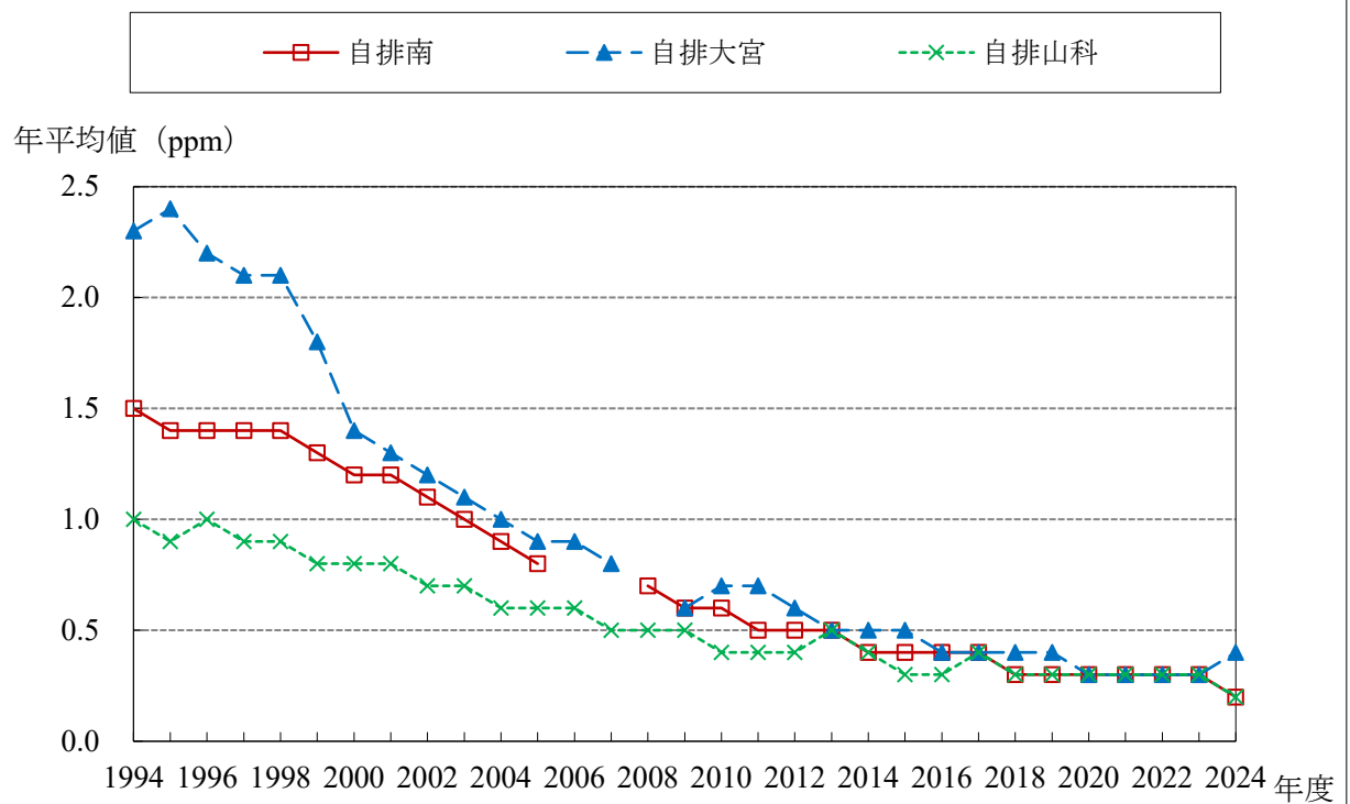
CO 経年変化グラフ (1994～2024年度)
