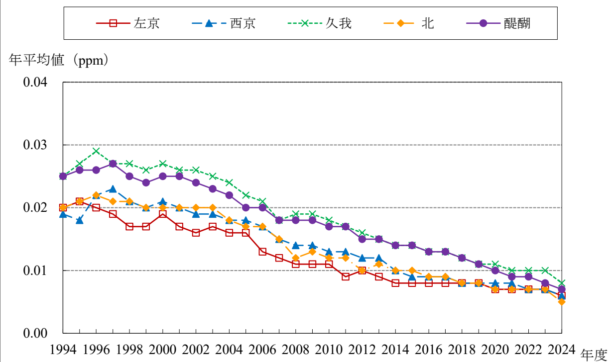
NO 2 経年変化グラフ (1994～2024年度)
