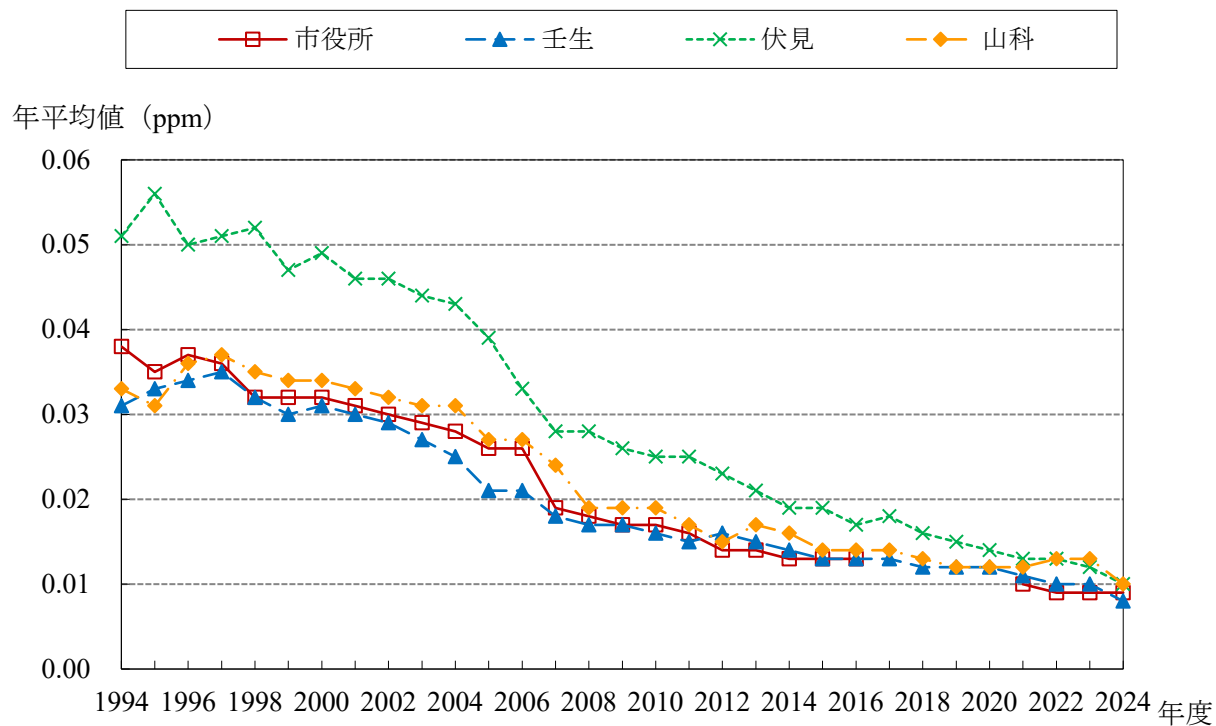
NOx 経年変化グラフ (1994～2024年度)
