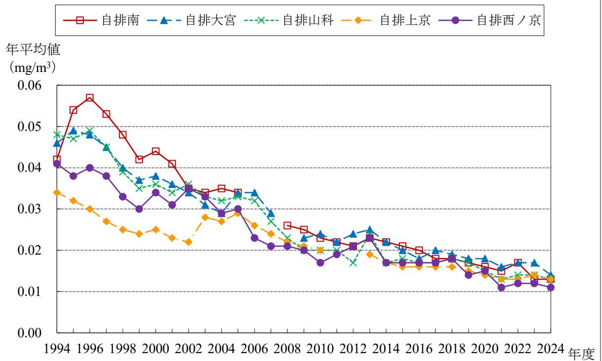
SPM 経年変化グラフ (1994～2024年度)
