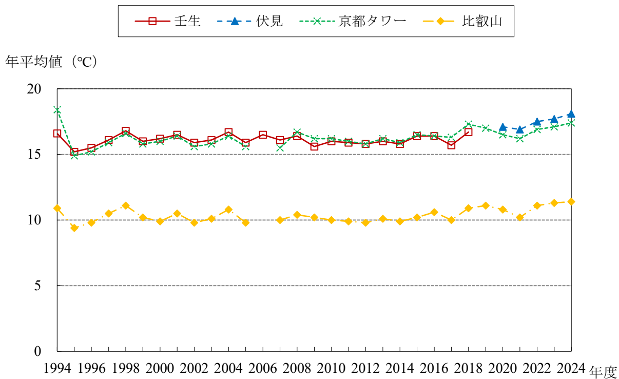
TEMP 経年変化グラフ (1994～2024年度)
