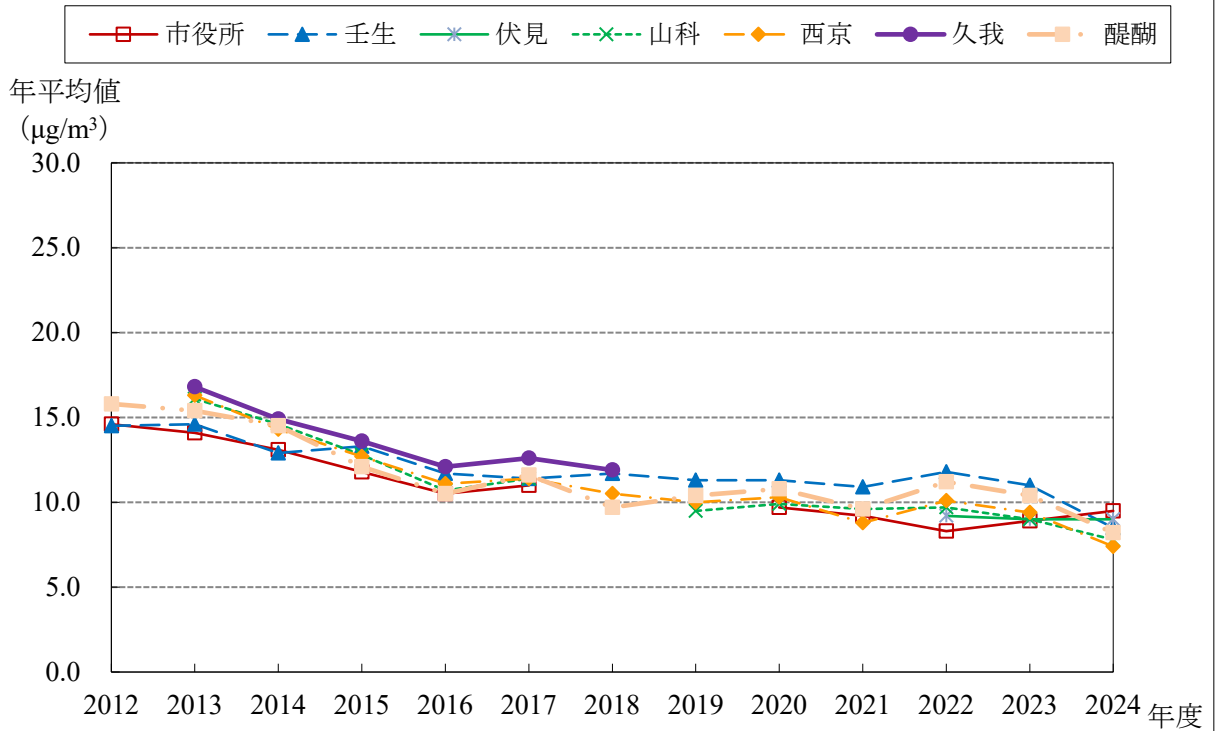
PM2.5 経年変化グラフ (2012～2024年度)
