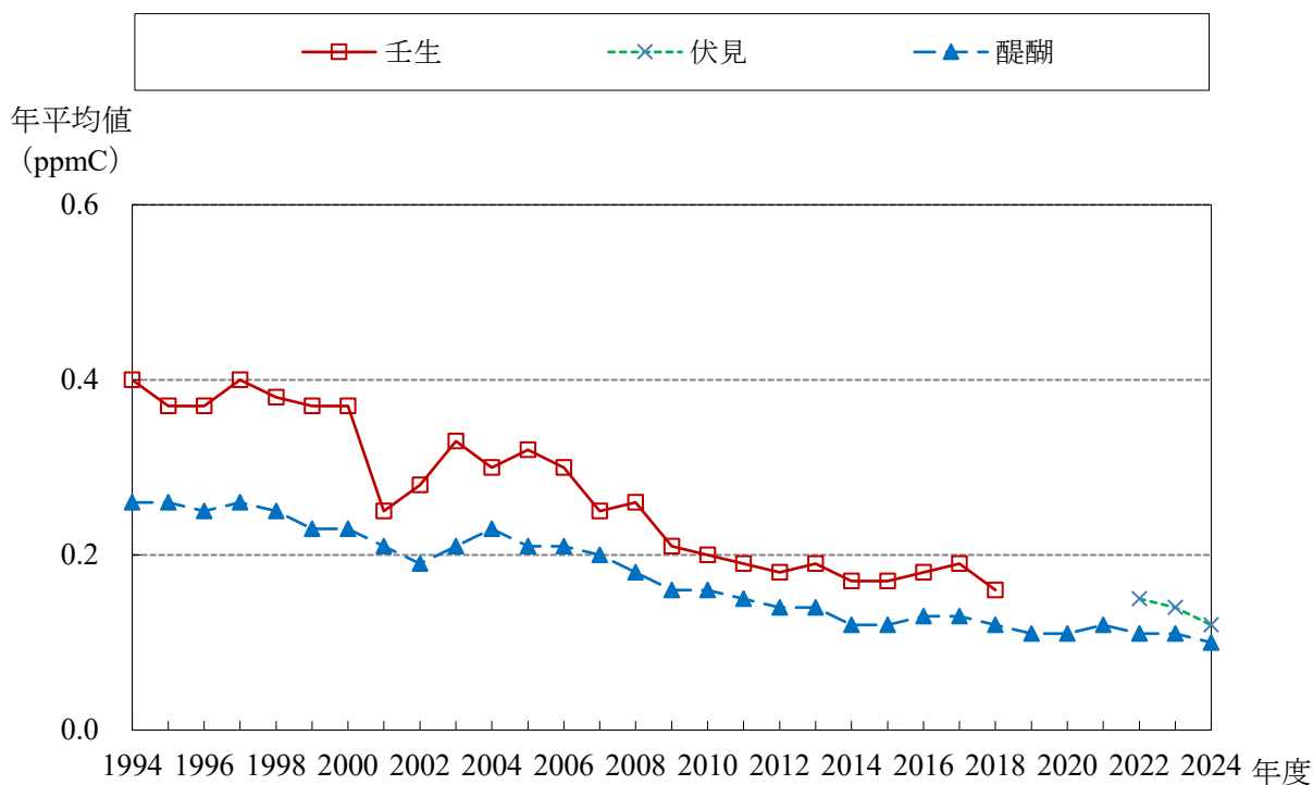
NMHC 経年変化グラフ (1994～2024年度)
