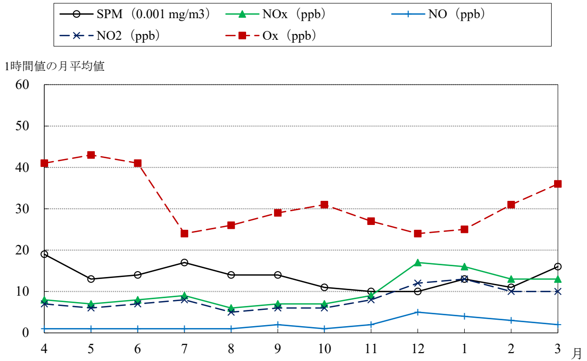
久我 経月変化グラフ (2024年4月 ~ 2025年3月)
