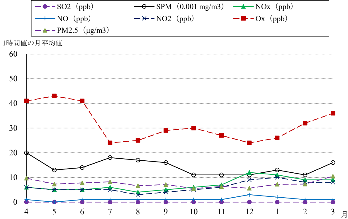
西京 経月変化グラフ (2024年4月 ~ 2025年3月)
