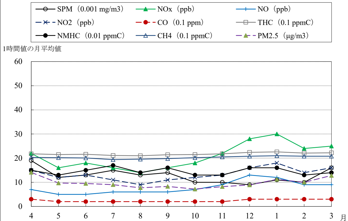
自排南 経月変化グラフ (2024年4月 ~ 2025年3月)
