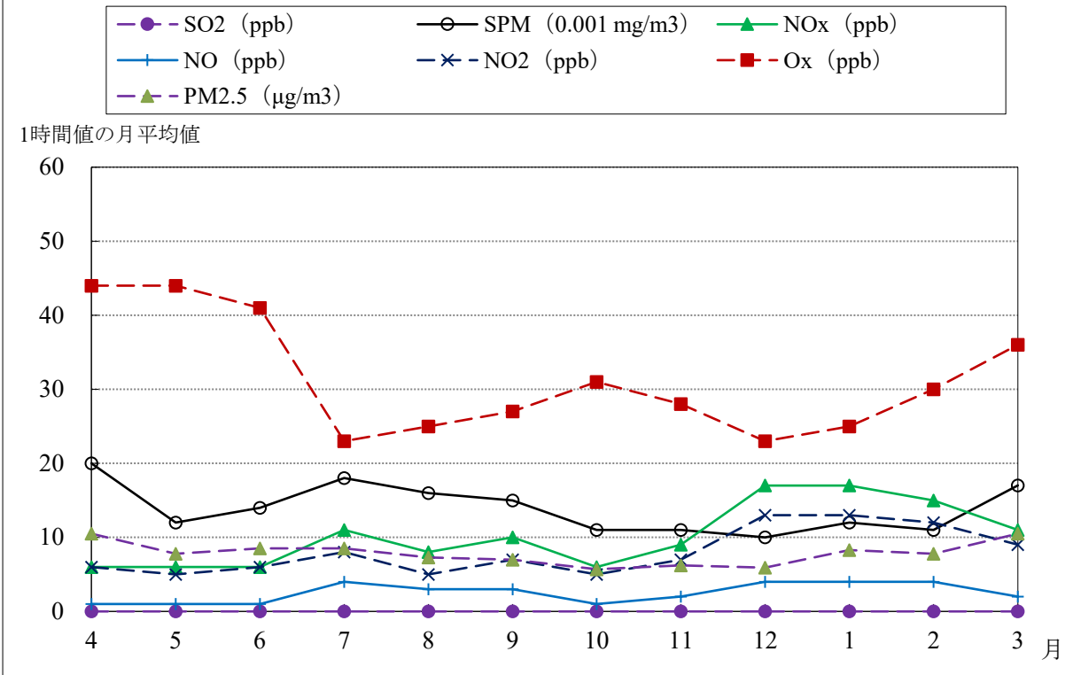
山科 経月変化グラフ (2024年4月 ~ 2025年3月)
