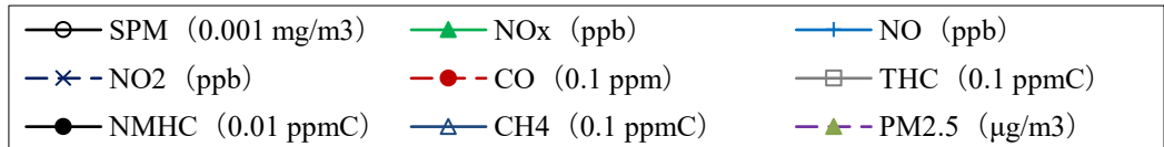
自排山科 経月変化グラフ (2024年4月 ~ 2025年3月)
