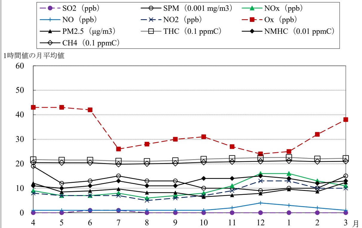
伏見 経月変化グラフ (2024年4月 ~ 2025年3月)
