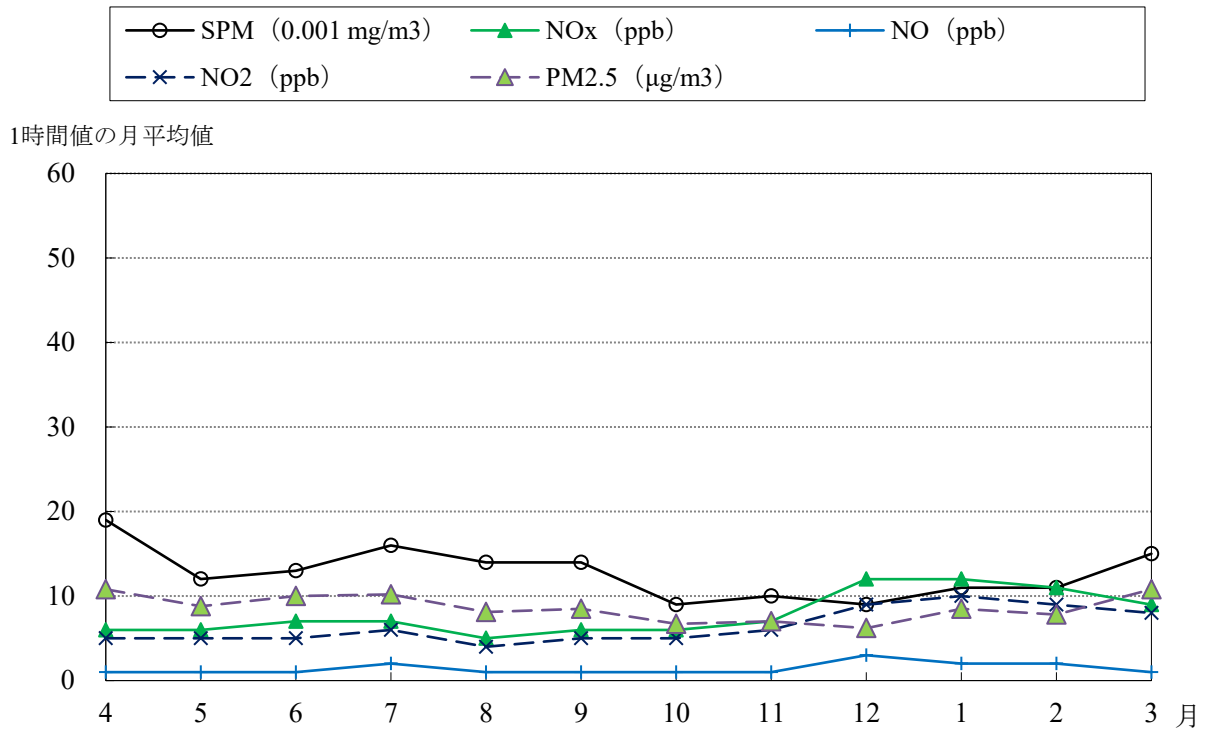
自排上京 経月変化グラフ (2024年4月 ~ 2025年3月)
