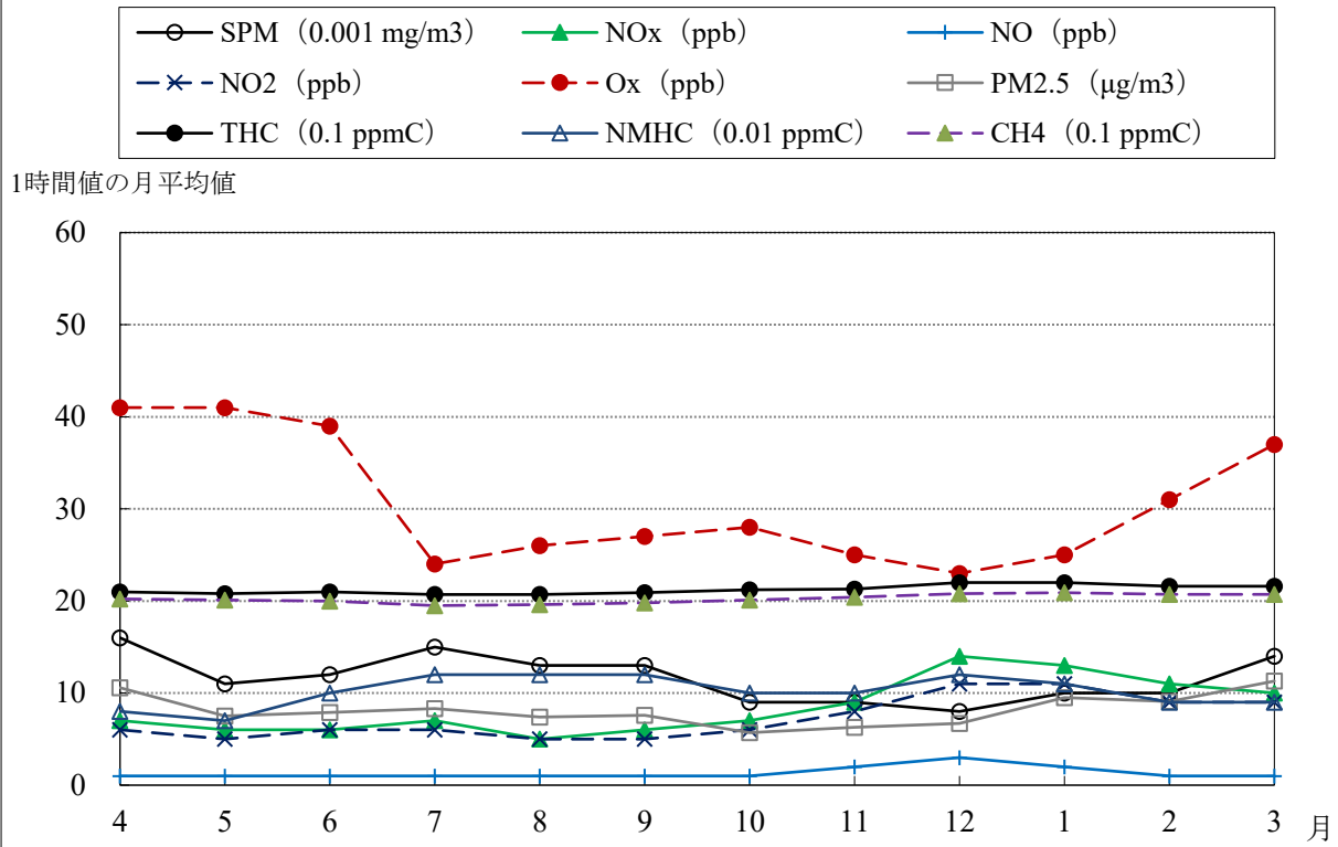
醍醐 経月変化グラフ (2024年4月 ~ 2025年3月)
