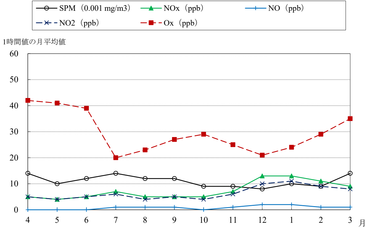
左京 経月変化グラフ (2024年4月 ~ 2025年3月)
