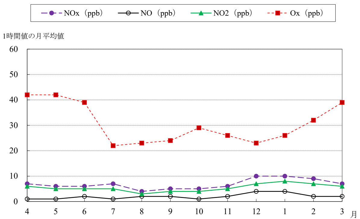
北 経月変化グラフ (2024年4月 ~ 2025年3月)
