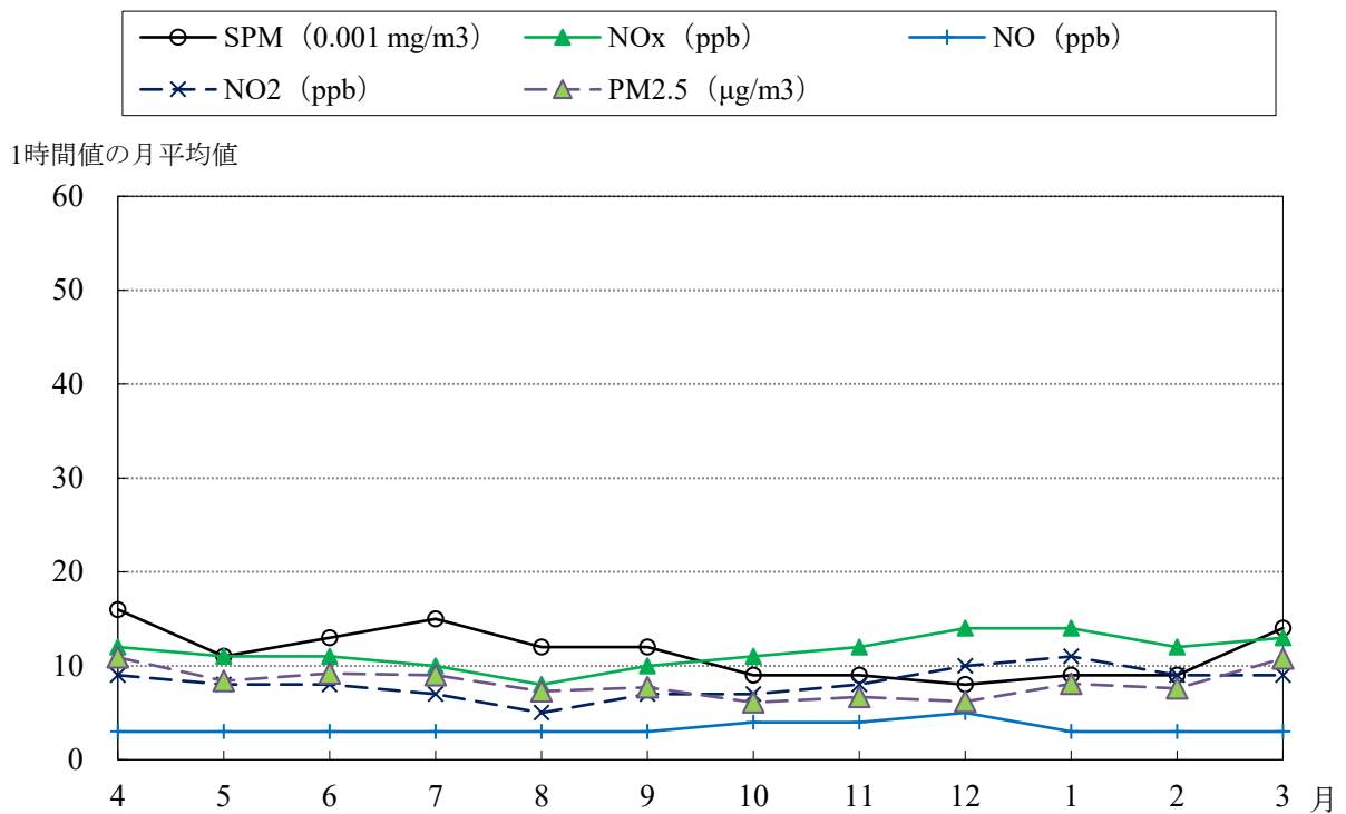
自排西ノ京 経月変化グラフ (2024年4月 ~ 2025年3月)
