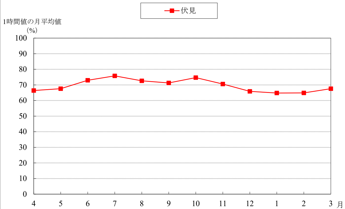
HUM 経月変化グラフ (2024年4月 ~ 2025年3月)
