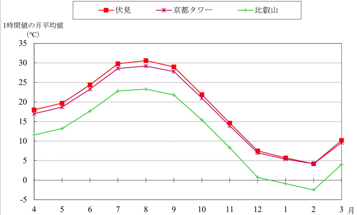
TEMP 経月変化グラフ (2024年4月 ~ 2025年3月)
