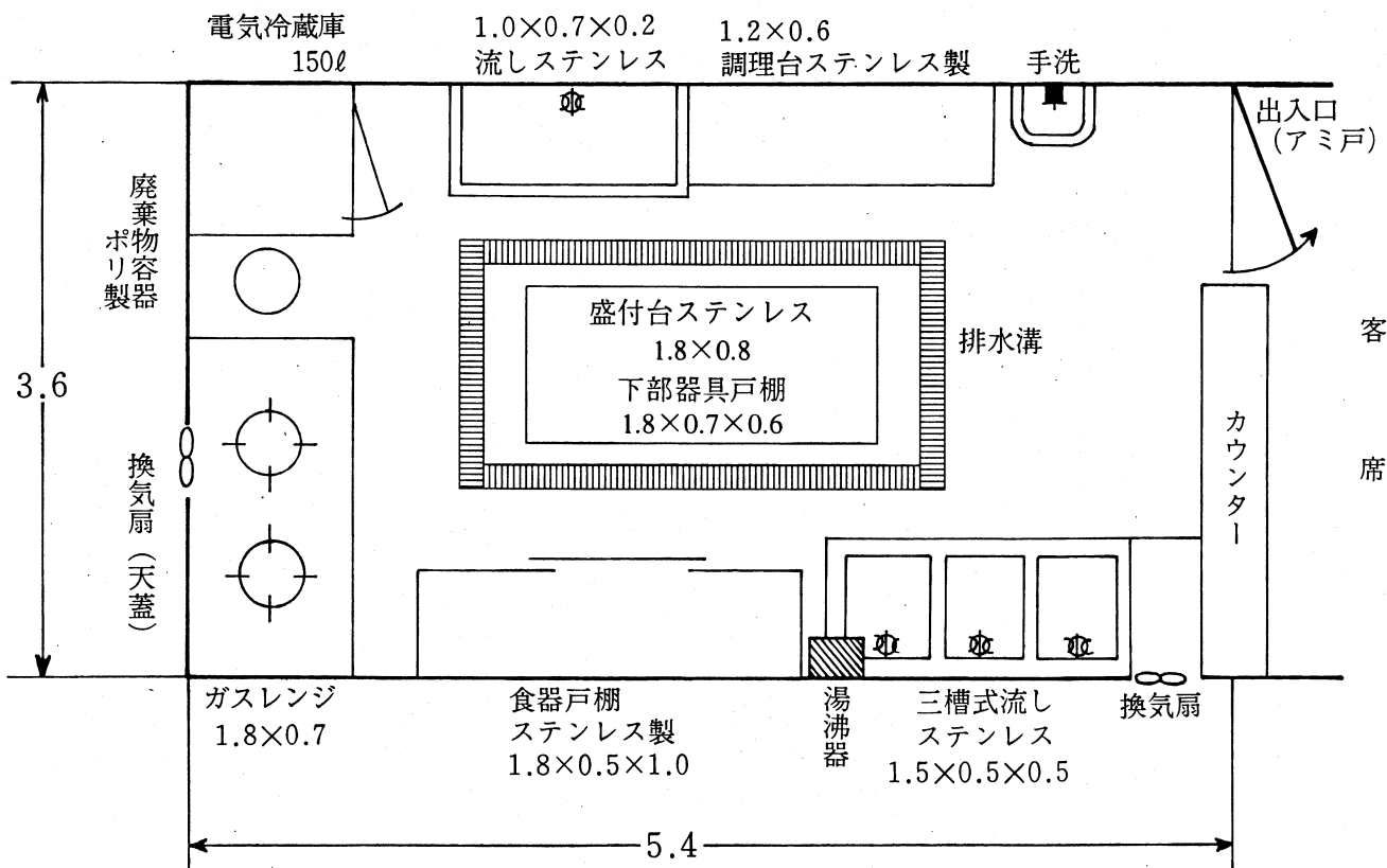
[営業所内の設備の配置図記入例]
