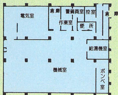
1 階平面図
