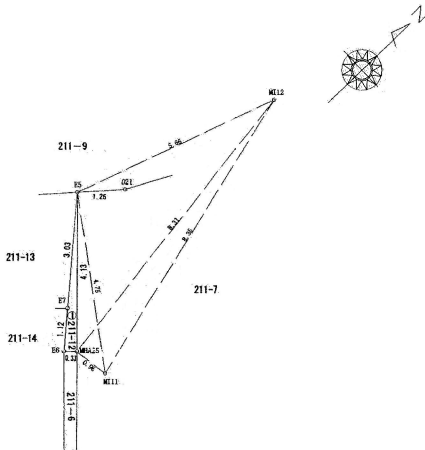
求積表
