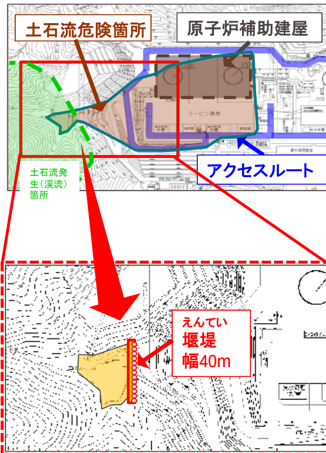
工事位置図
