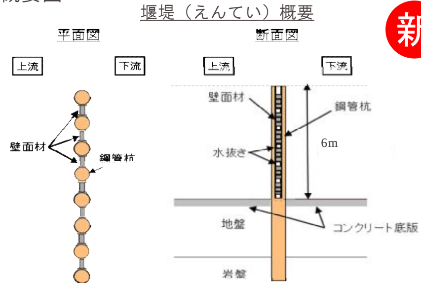
工事概要図
