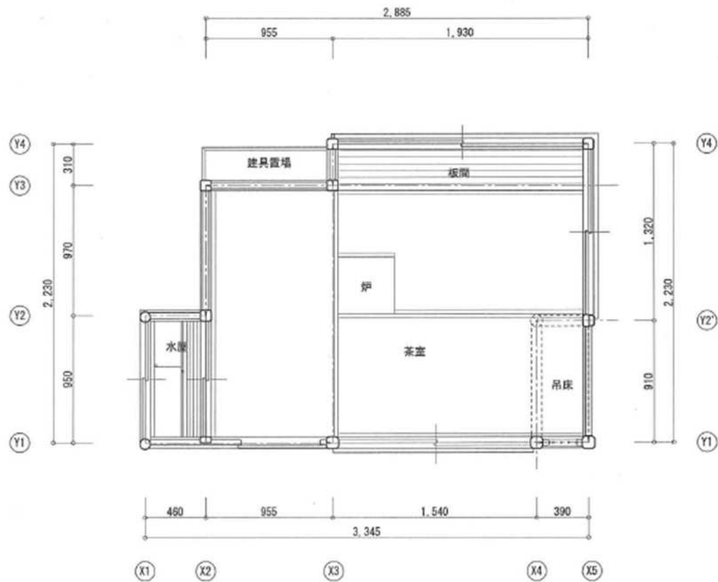
平面図
