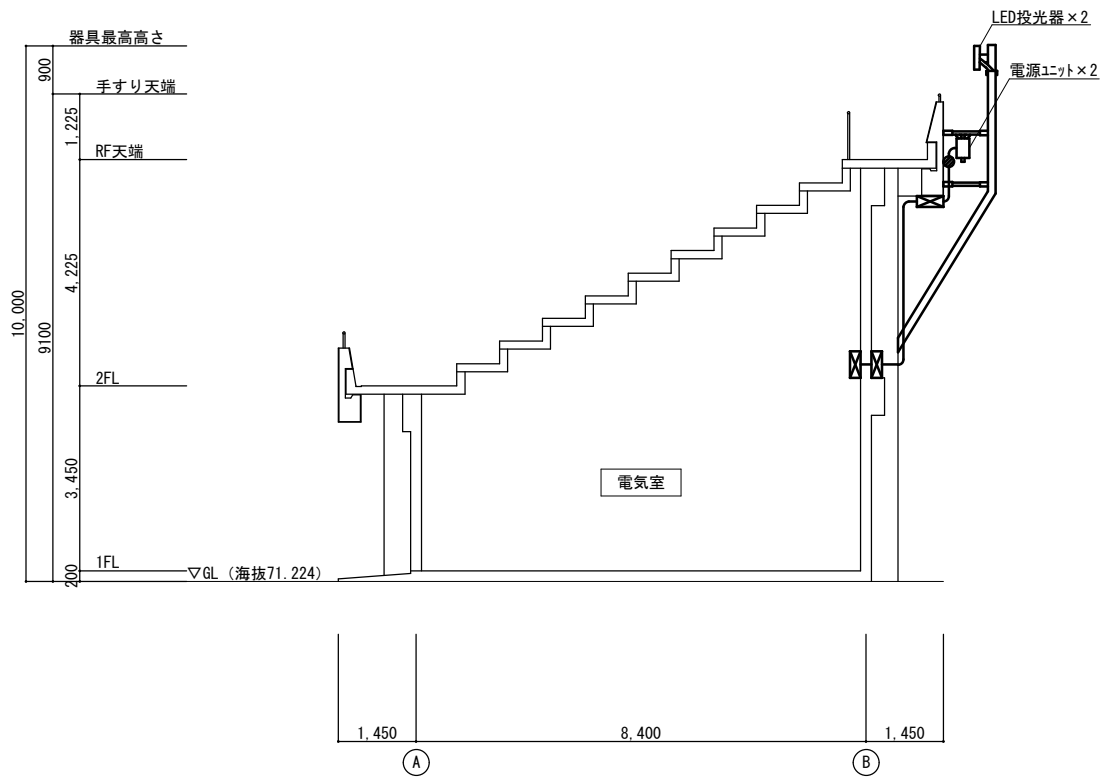
②通 断面図 S=1/100
