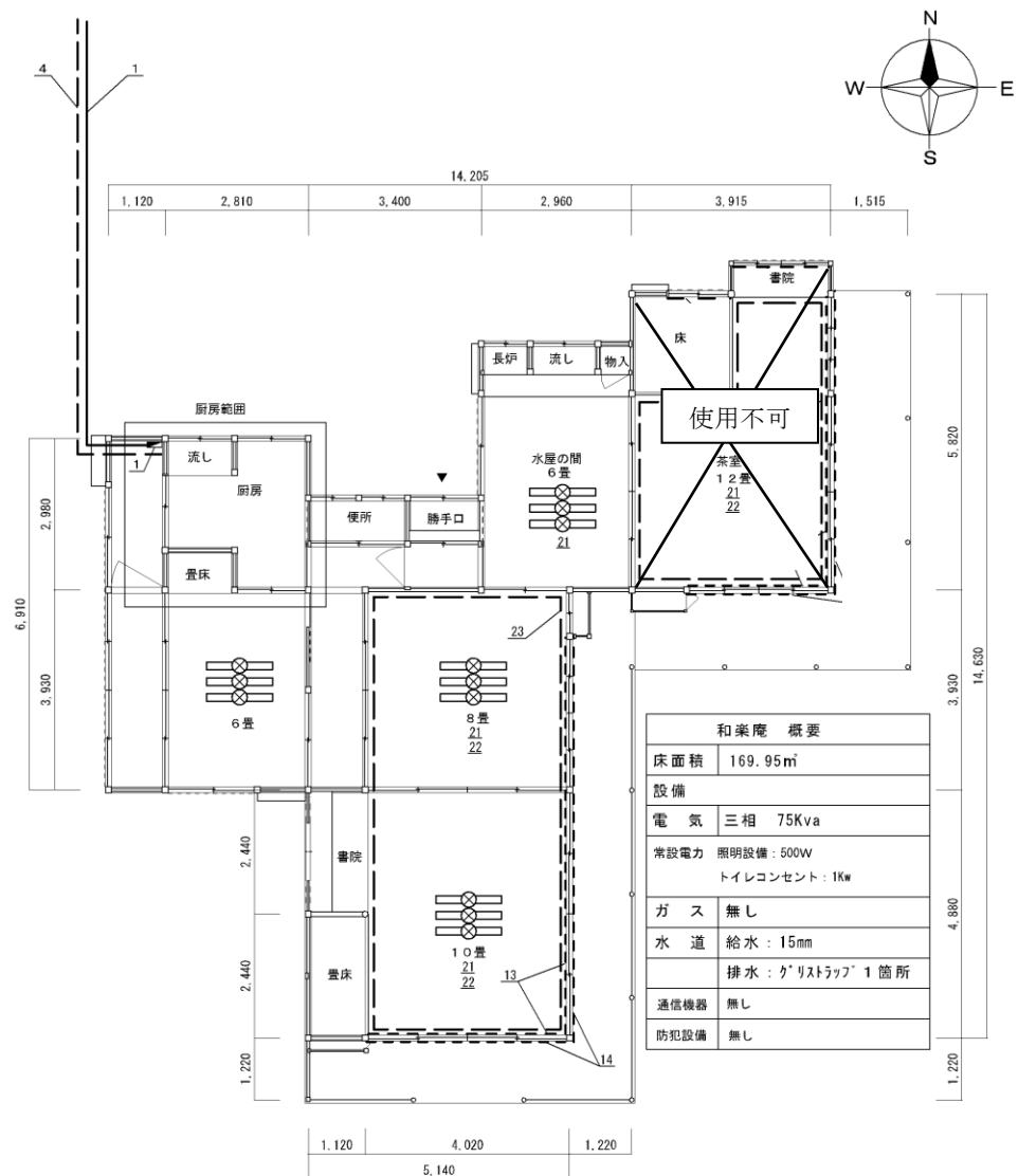
和楽庵 平面図 (1:100)
