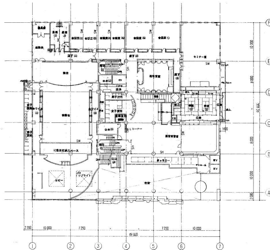
2階平面図 1:200
