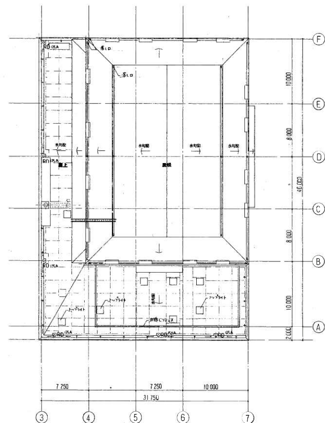
屋根伏図 1:200
