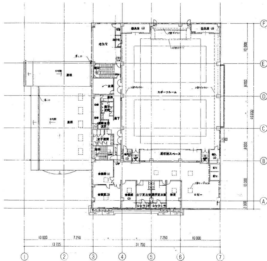
4階平面図 1:200
