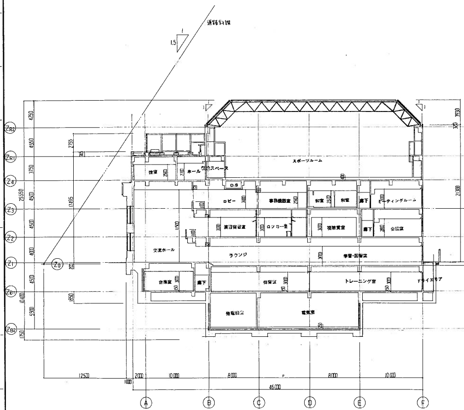
Y-Y 断面図
