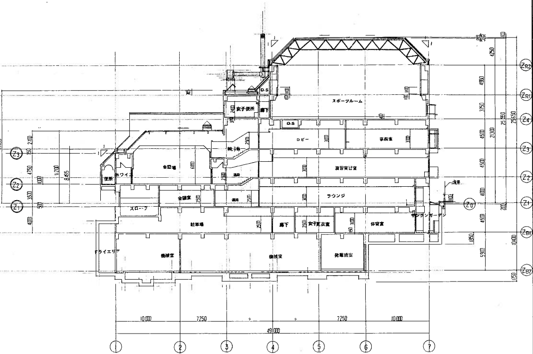
X-X 断面図
