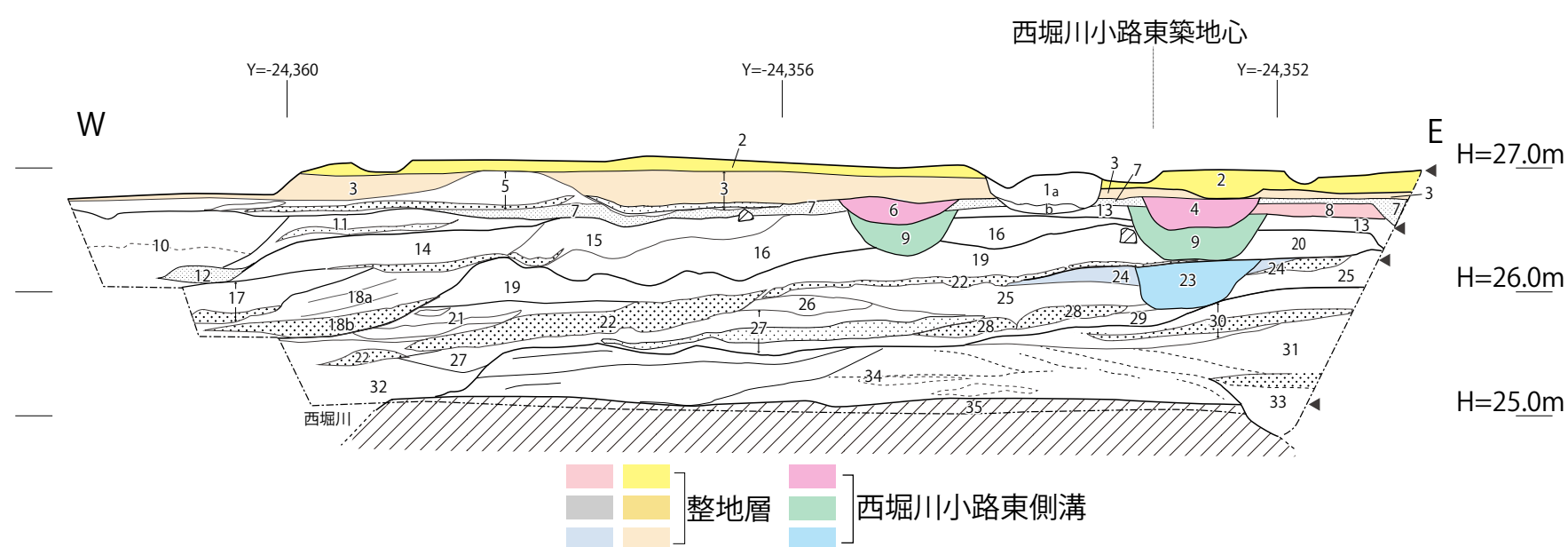
図4 1区中央壁（図3）の断面図
