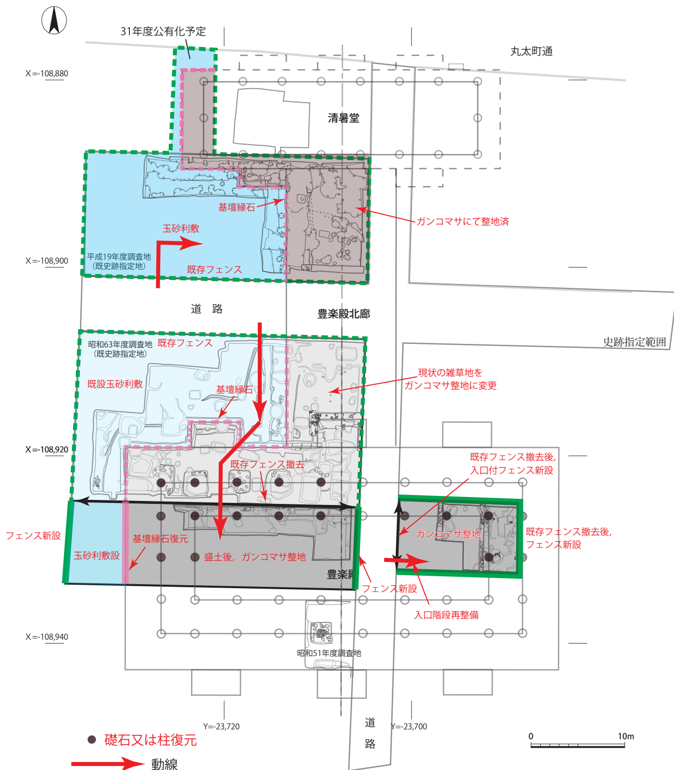
事業計画図 (S=1:400)
