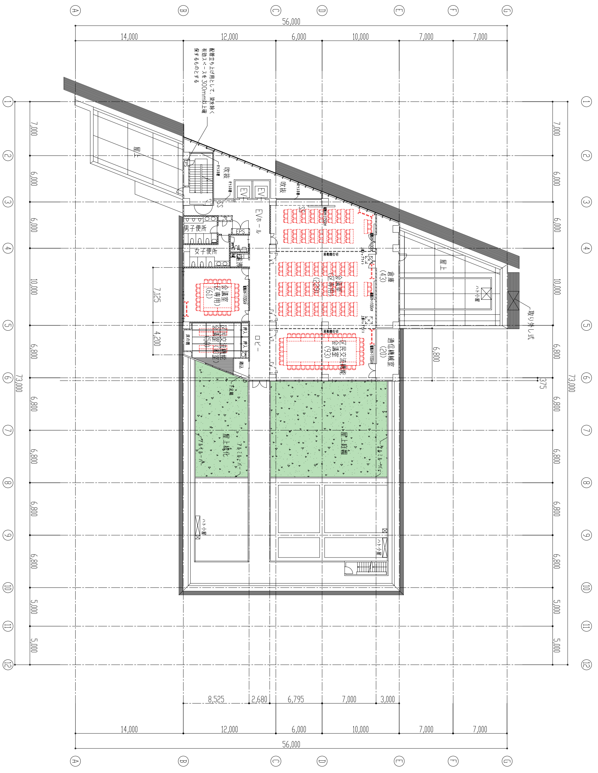
4階平面図 1/300
