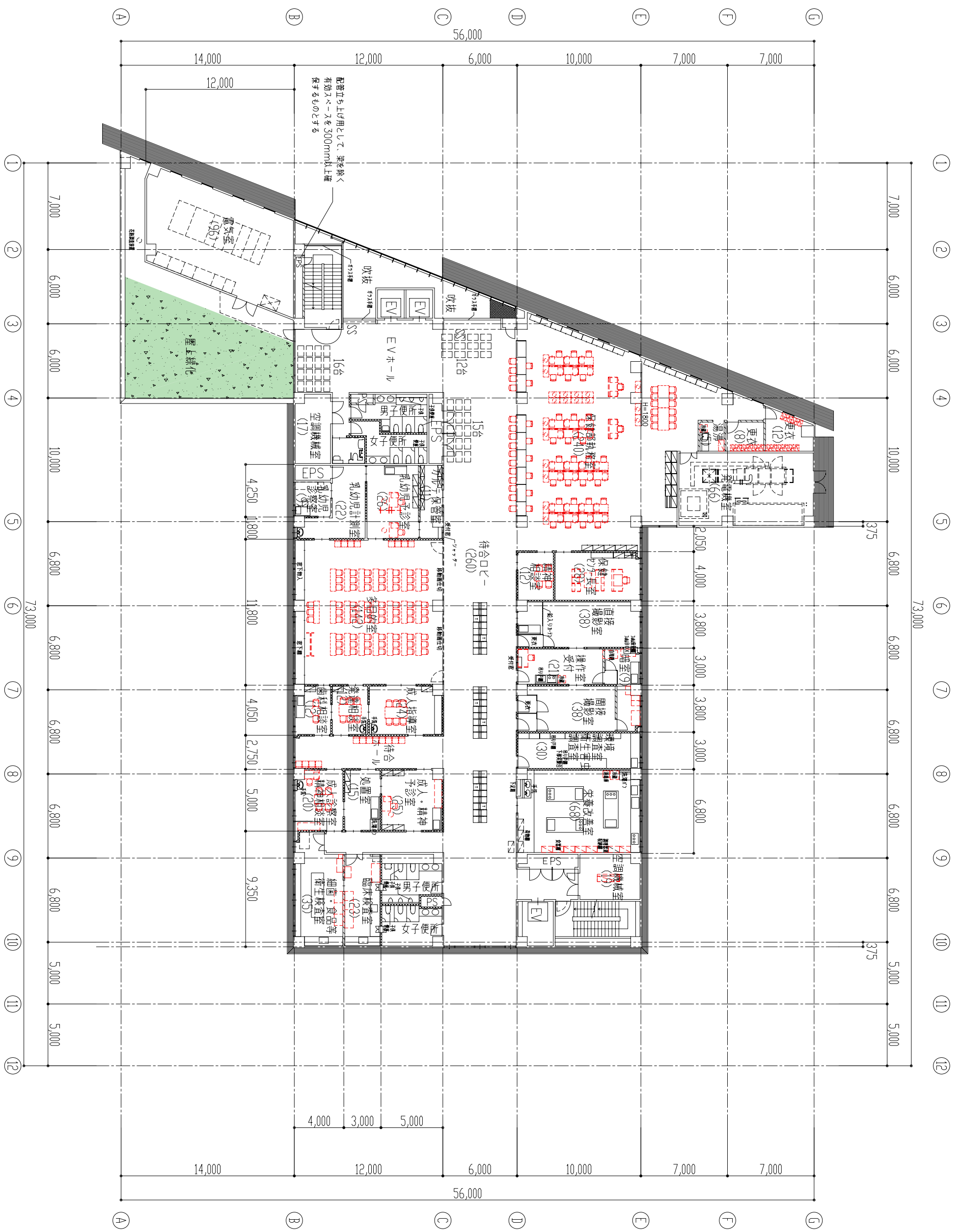
3階平面図 1/300
