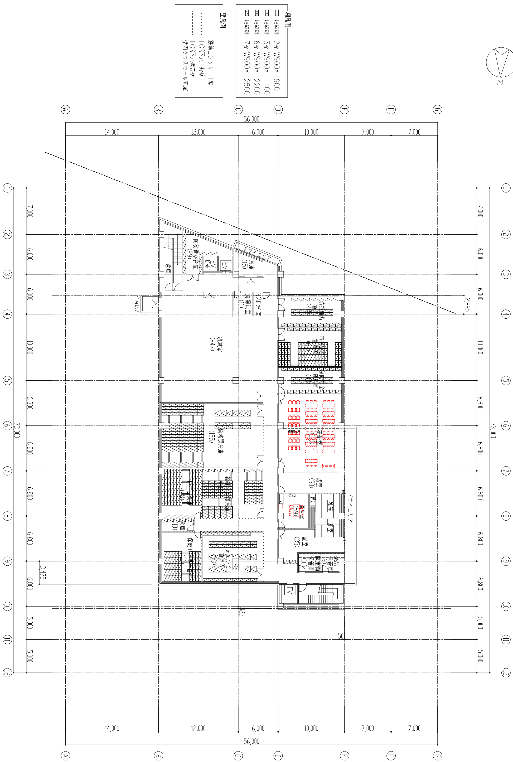
地下1階平面図 1/300
