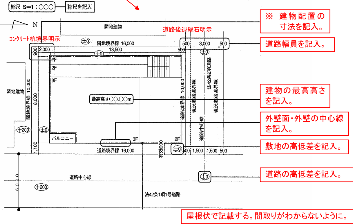
配置図
