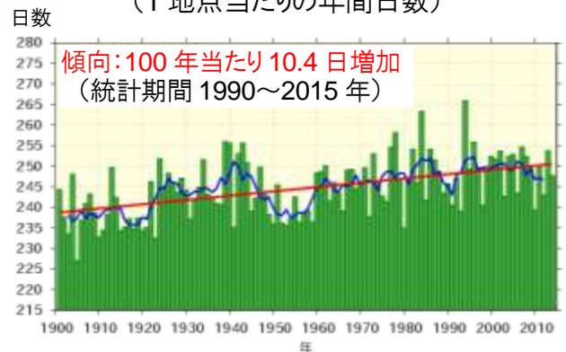
日降水量 1.0mm 未満の日数 (全国) 日数 (1 地点当たりの年間日数)
