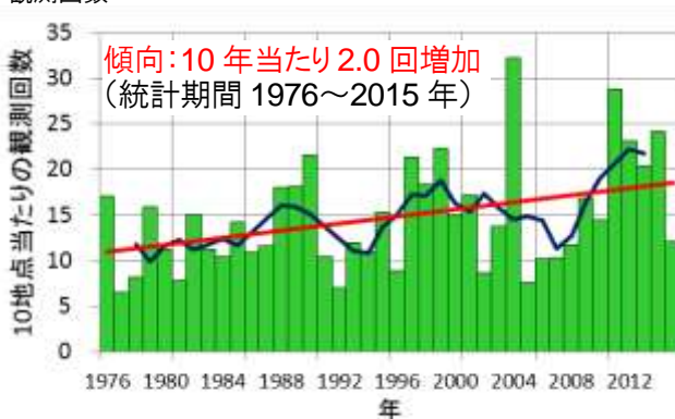
1 時間降水量 30mm 以上の年間観測回数 (近畿) 観測回数 (10 地点当たりの観測回数)
