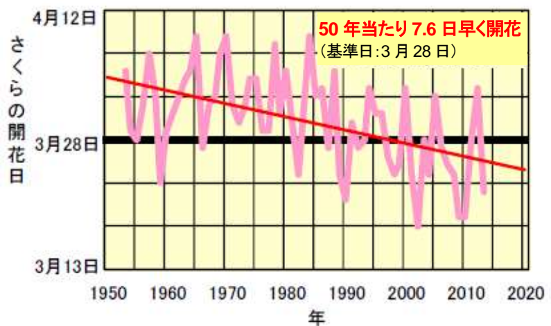
図25 京都(京都地方气象台)のソメイヨシノの開花日の経年変化
