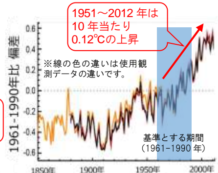
図4 世界の年平均気温
