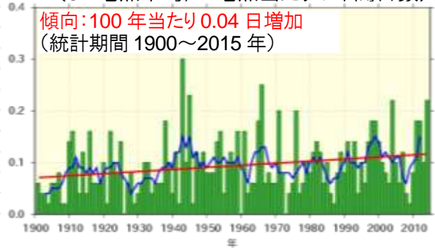
日降水量 200mm 以上の日数 (全国) 日数 (51 地点平均, 1 地点当たりの年間日数)
