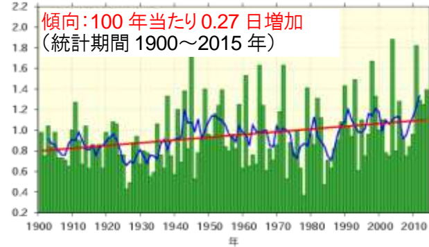
日降水量 100mm 以上の日数 (全国) 日数 (51 地点平均, 1 地点当たりの年間日数)
