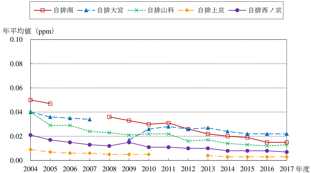
NO 経年変化グラフ (2004～2017年度)
