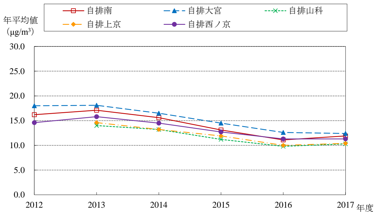
PM2.5 経年変化グラフ (2012～2017年度)
