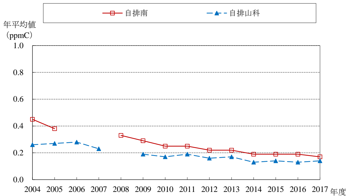
NMHC 経年変化グラフ (2004～2017年度)
