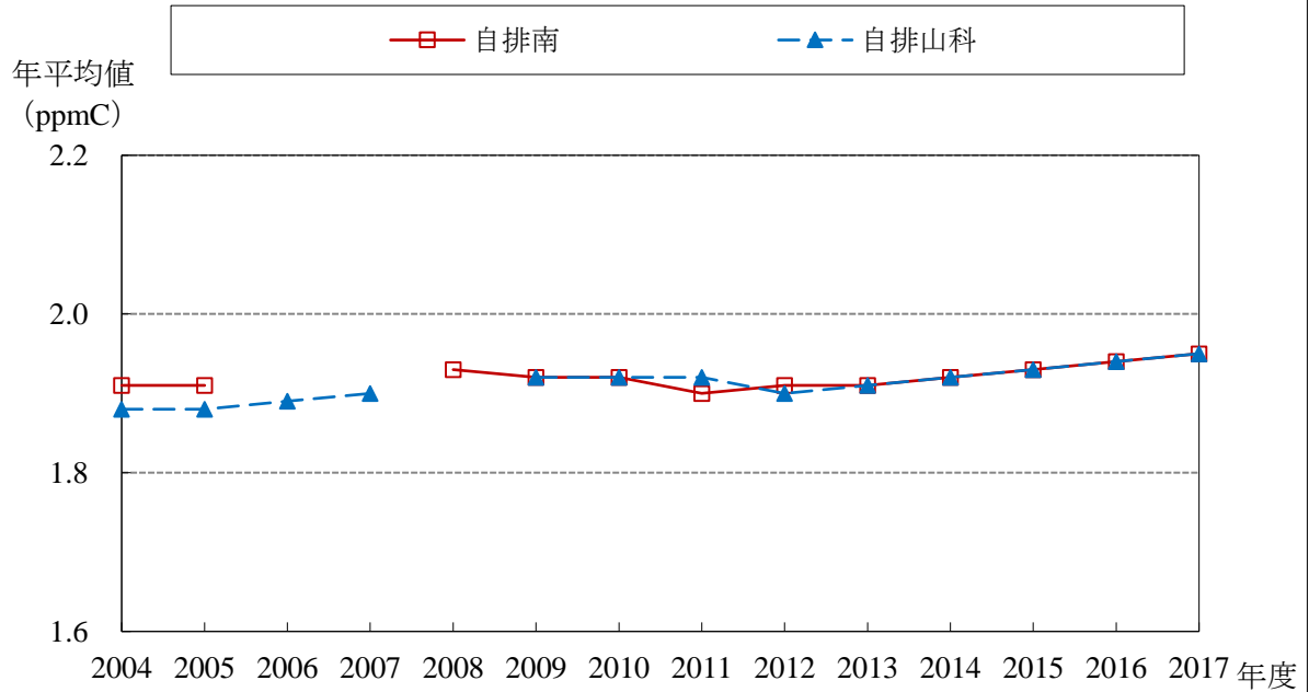
CH 4 経年変化グラフ (2004～2017年度)
