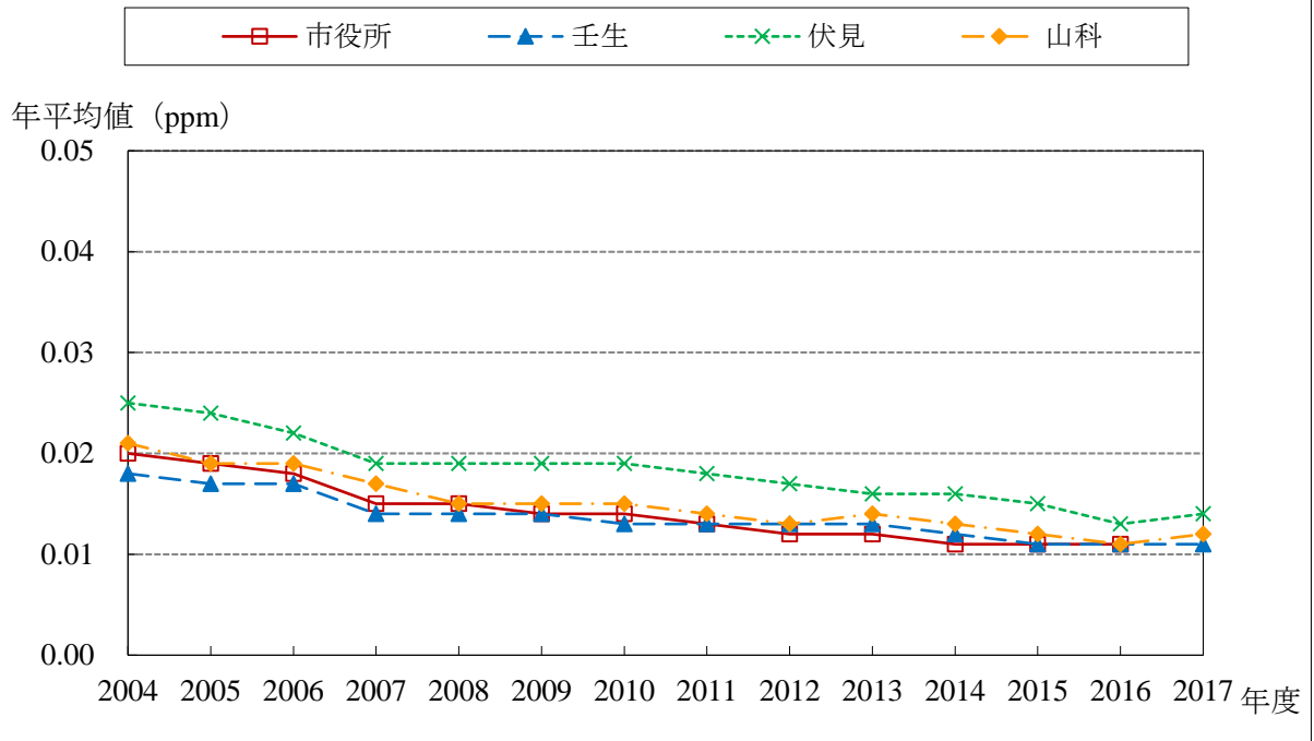
NO 2 経年変化グラフ (2004～2017年度)
