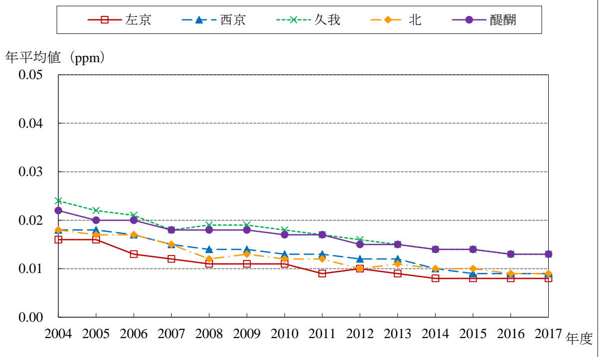
NO 2 経年変化グラフ (2004～2017年度)
