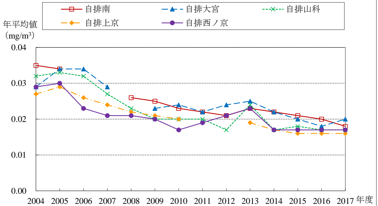
SPM 経年変化グラフ (2004～2017年度)
