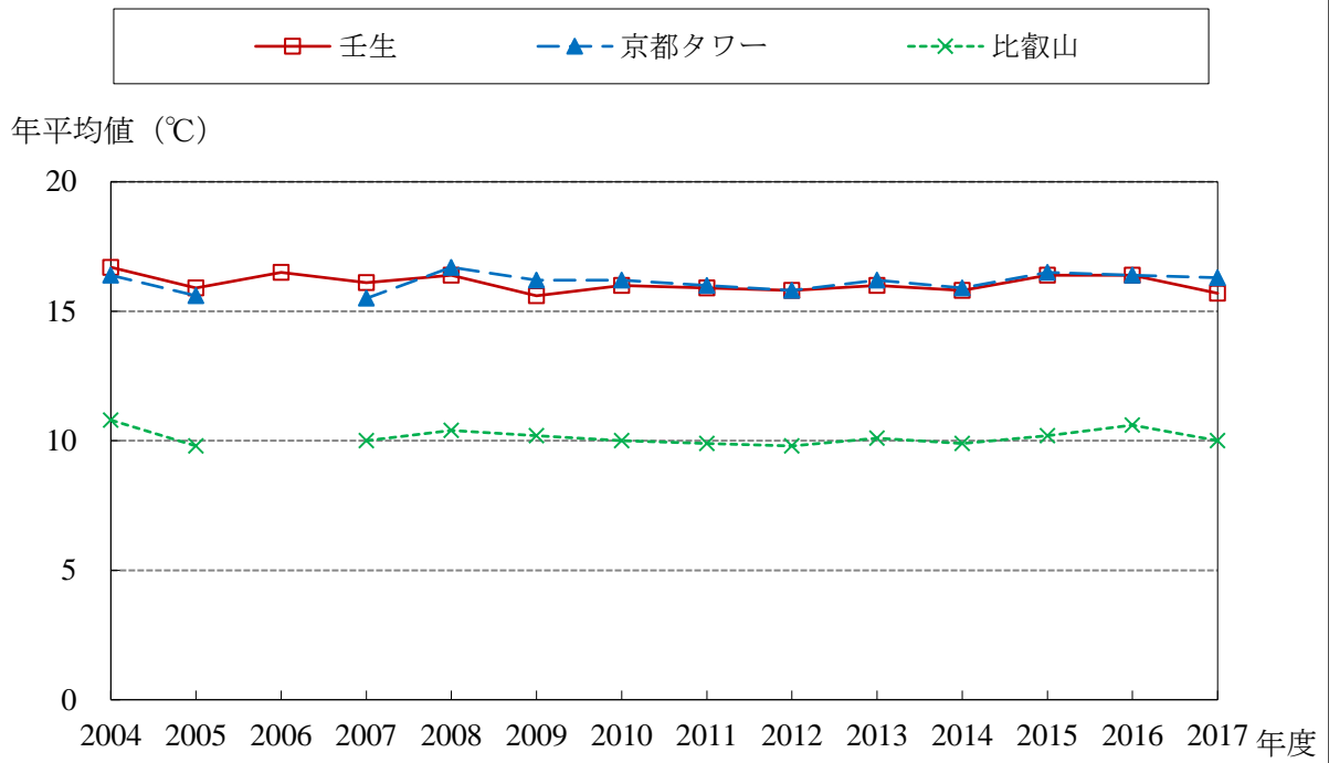
TEMP 経年変化グラフ (2004～2017年度)
