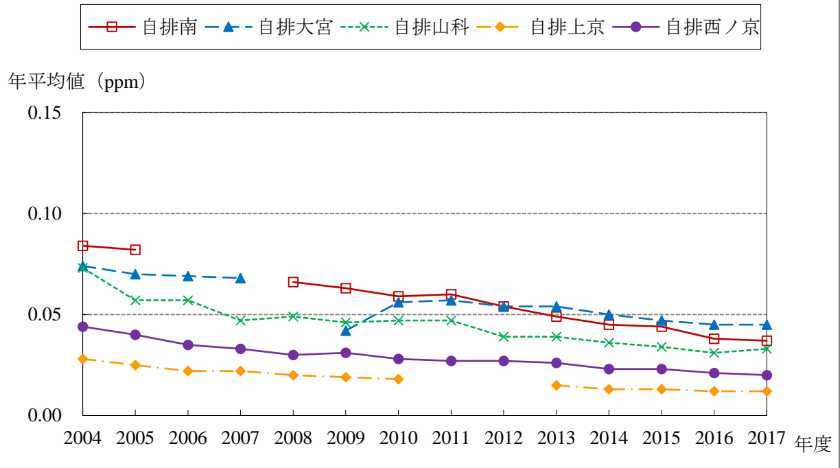
NOx 経年変化グラフ (2004～2017年度)
