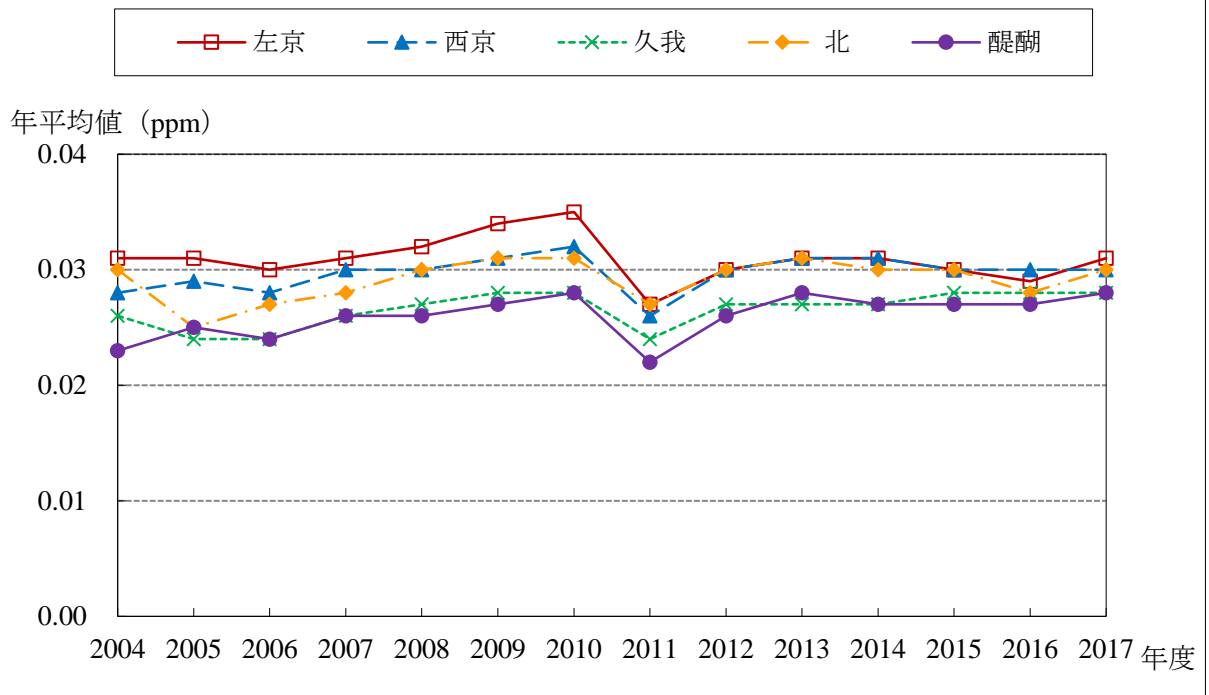
Ox 経年変化グラフ (2004～2017年度)
