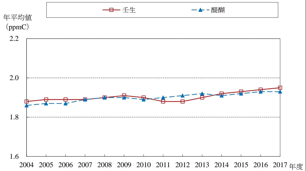
CH 4 経年変化グラフ (2004～2017年度)
