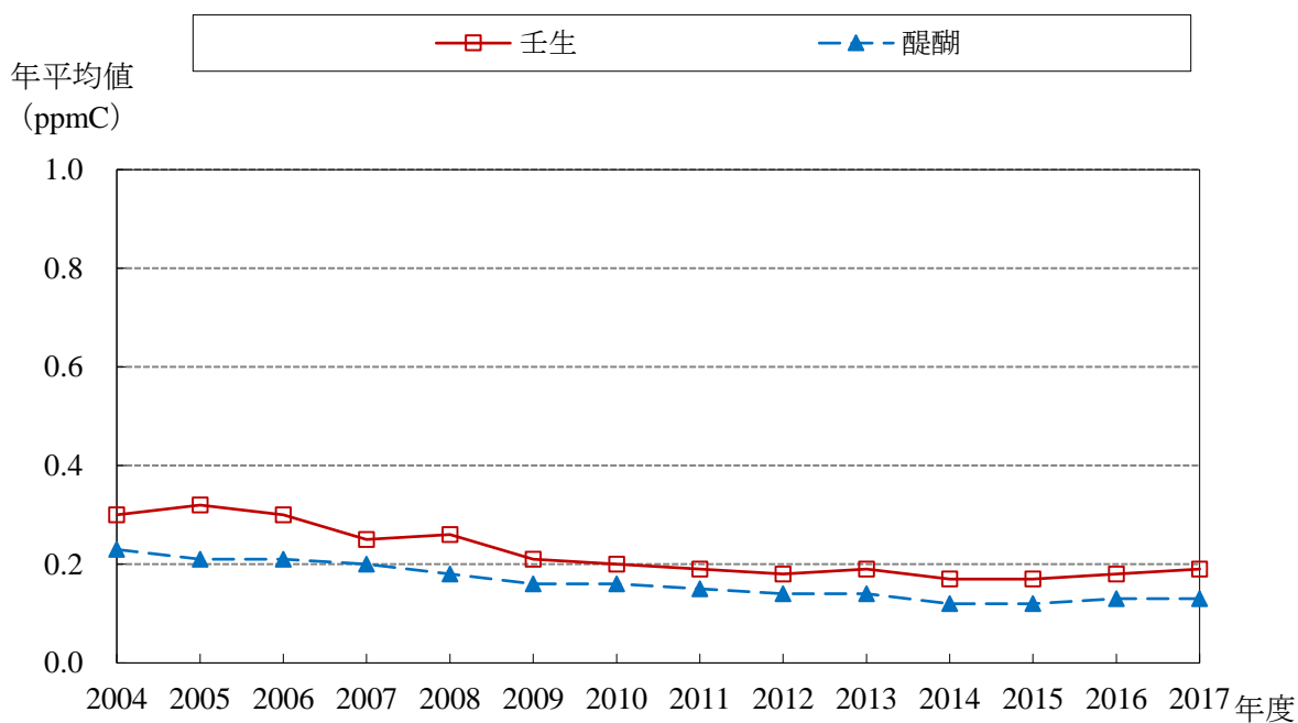
NMHC 経年変化グラフ (2004～2017年度)
