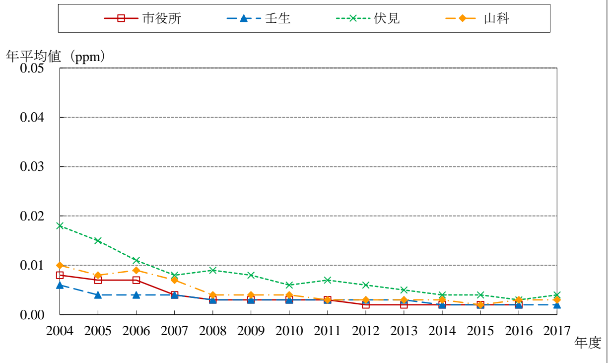
NO 経年変化グラフ (2004～2017年度)
