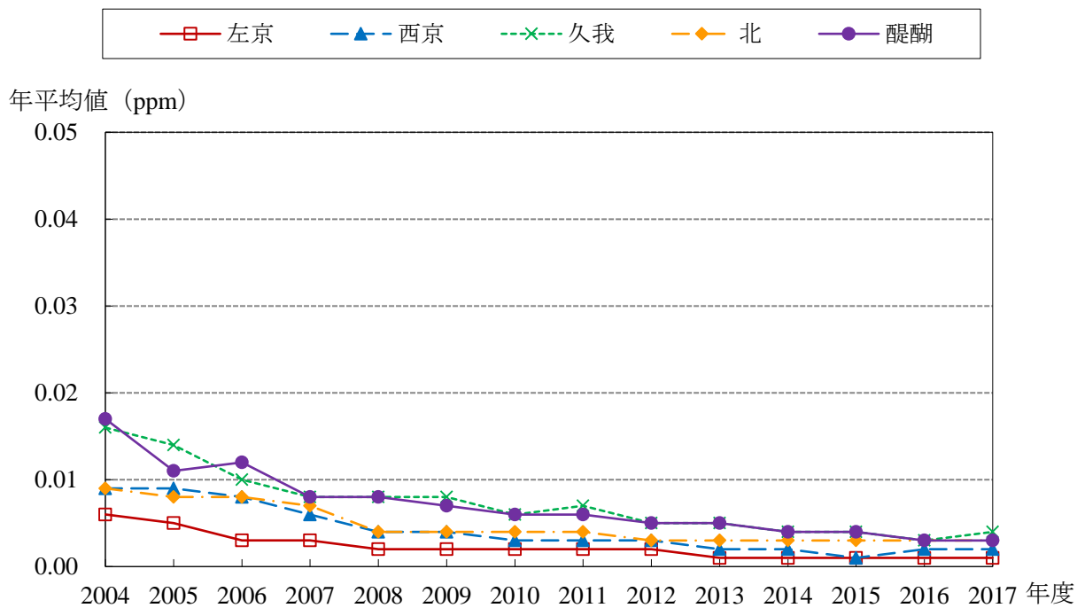
NO 経年変化グラフ (2004～2017年度)
