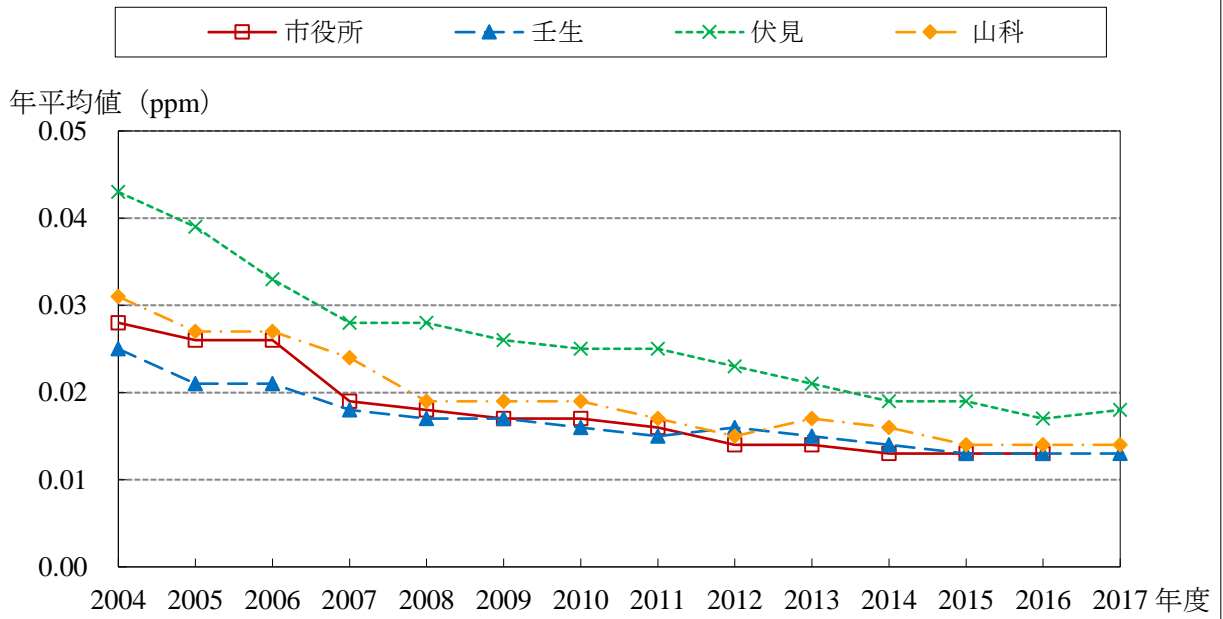
NOx 経年変化グラフ (2004～2017年度)
