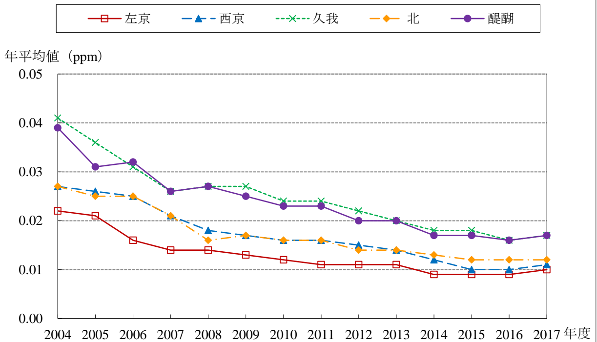
NOx 経年変化グラフ (2004～2017年度)
