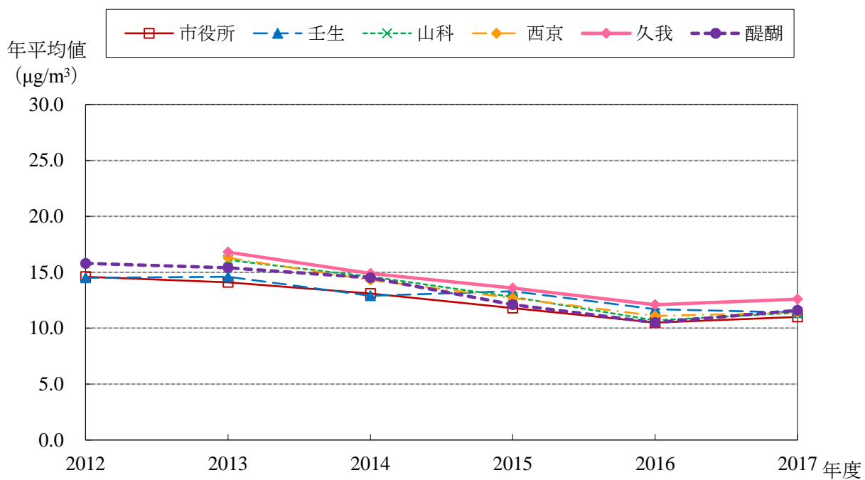
PM2.5 経年変化グラフ (2012～2017年度)
