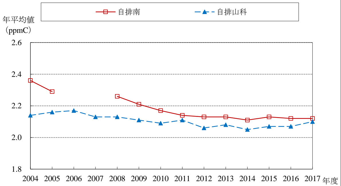
THC 経年変化グラフ (2004～2017年度)
