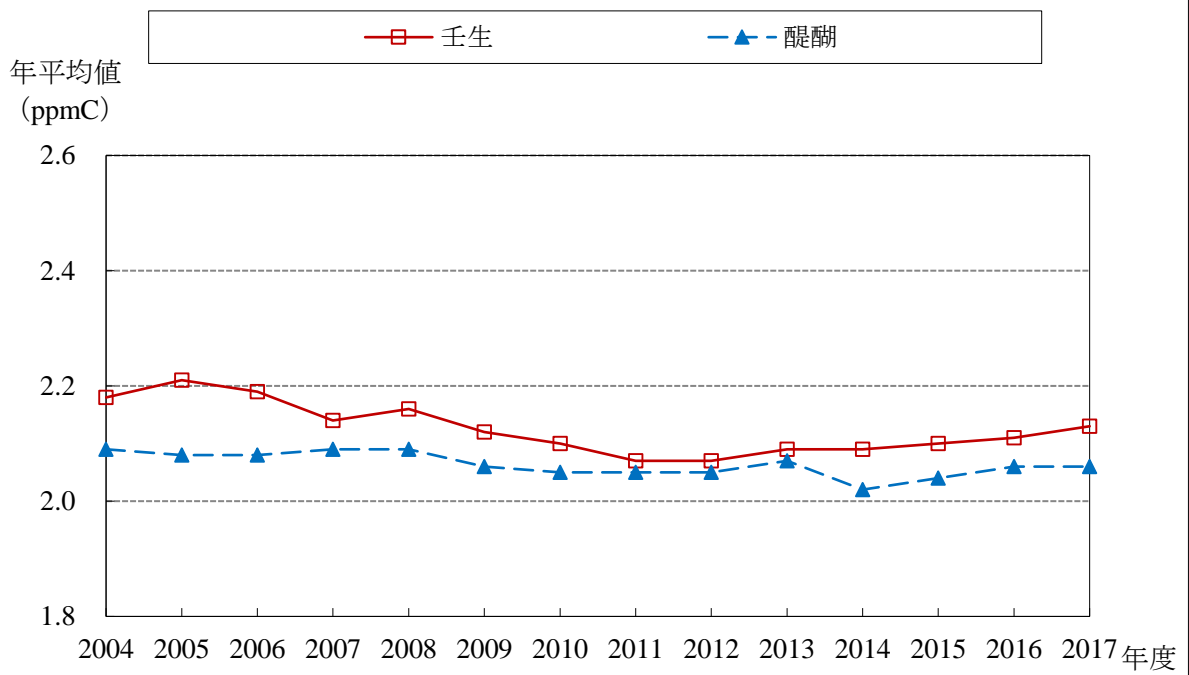
THC 経年変化グラフ (2004～2017年度)
