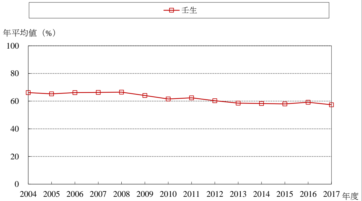
HUM 経年変化グラフ (2004～2017年度)
