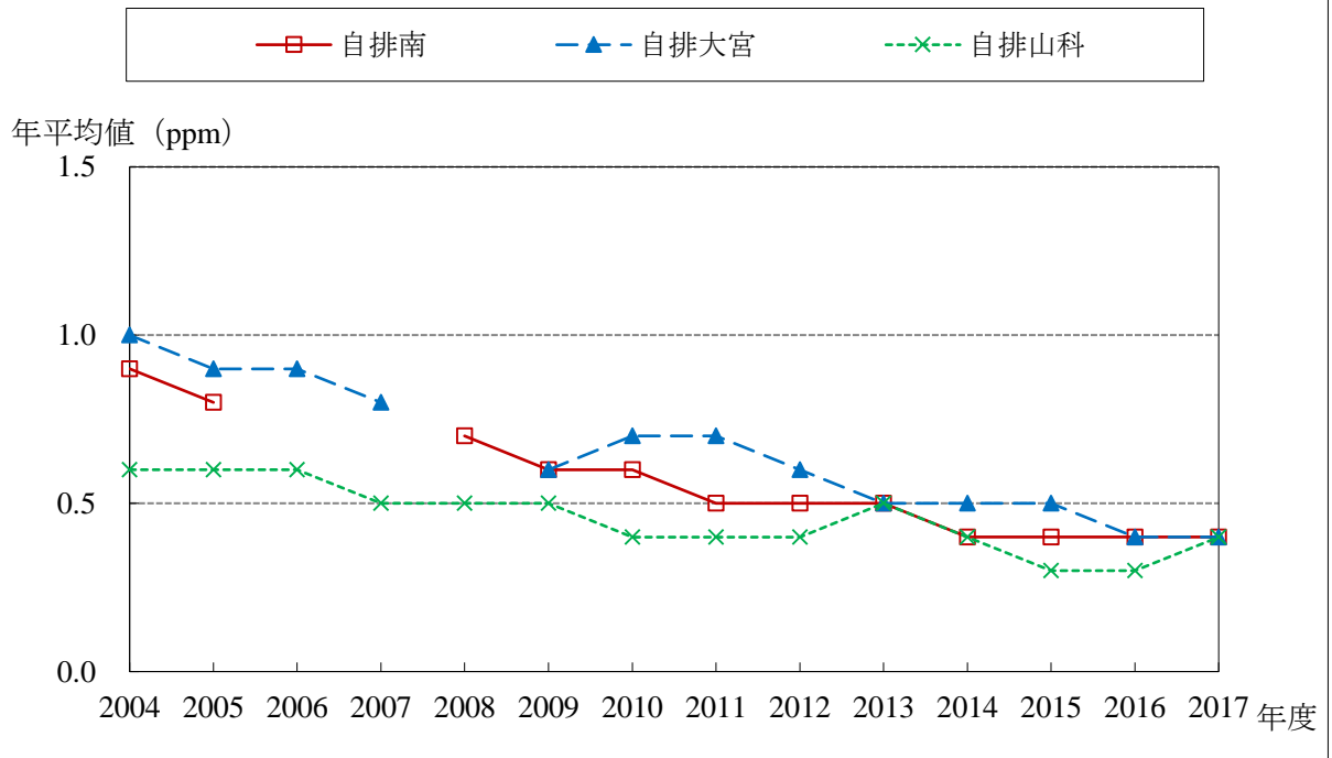
CO 経年変化グラフ (2004～2017年度)
