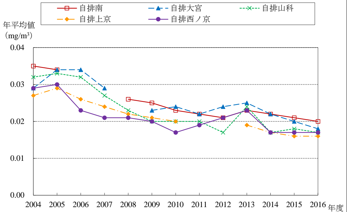
SPM 経年変化グラフ (2004～2016年度)
