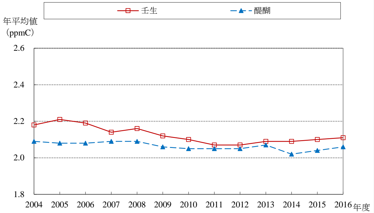
THC 経年変化グラフ (2004～2016年度)
