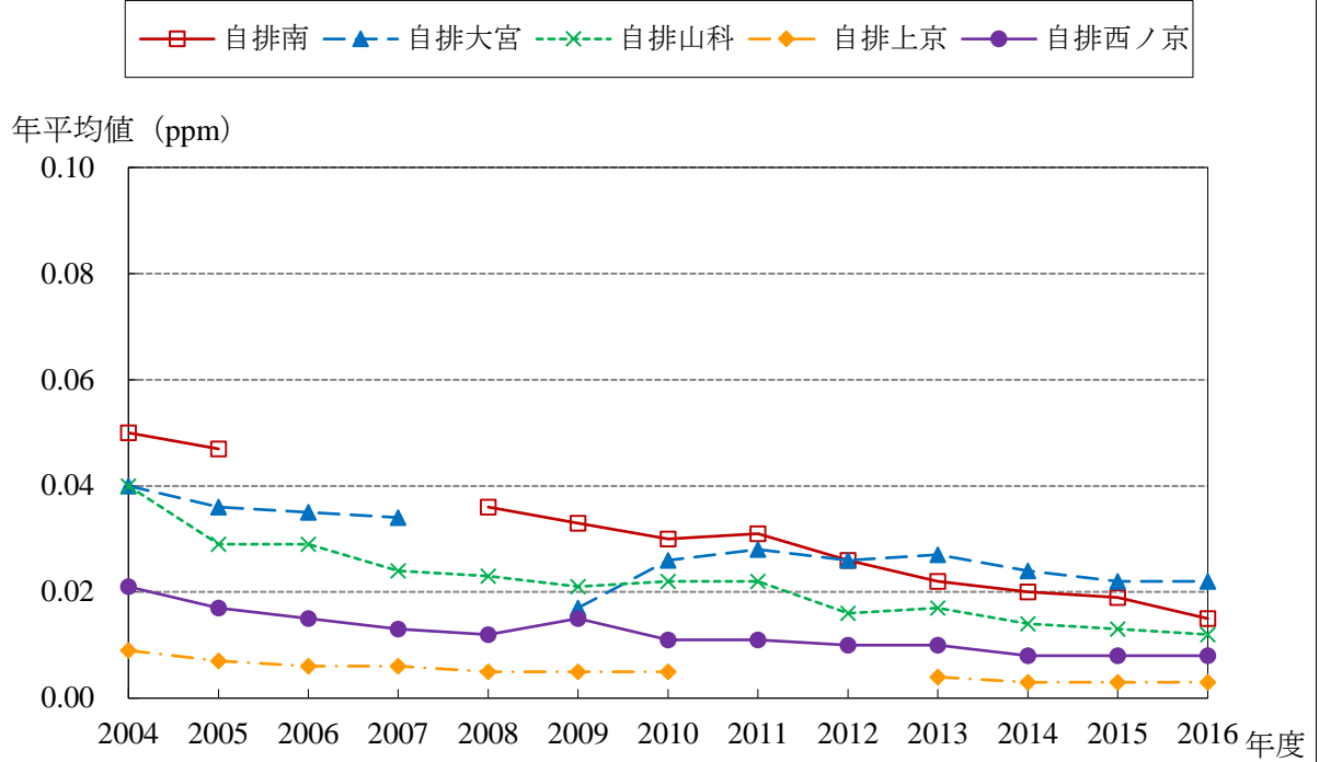
NO 経年変化グラフ (2004～2016年度)
