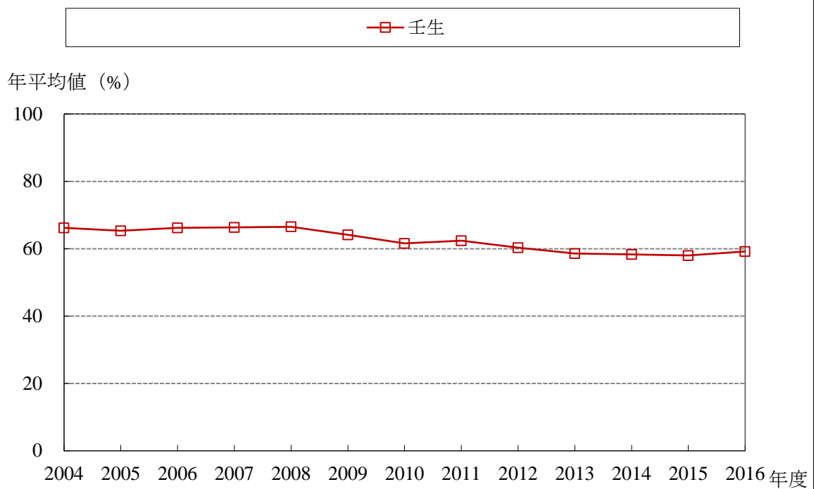
HUM 経年変化グラフ (2004～2016年度)
