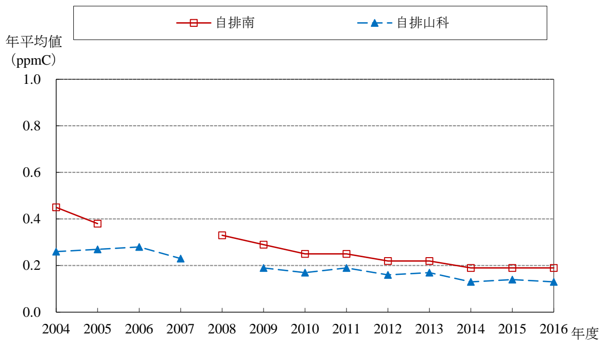
NMHC 経年変化グラフ (2004～2016年度)
