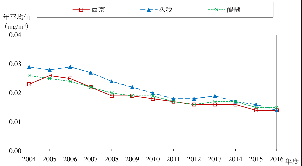
SPM 経年変化グラフ (2004～2016年度)
