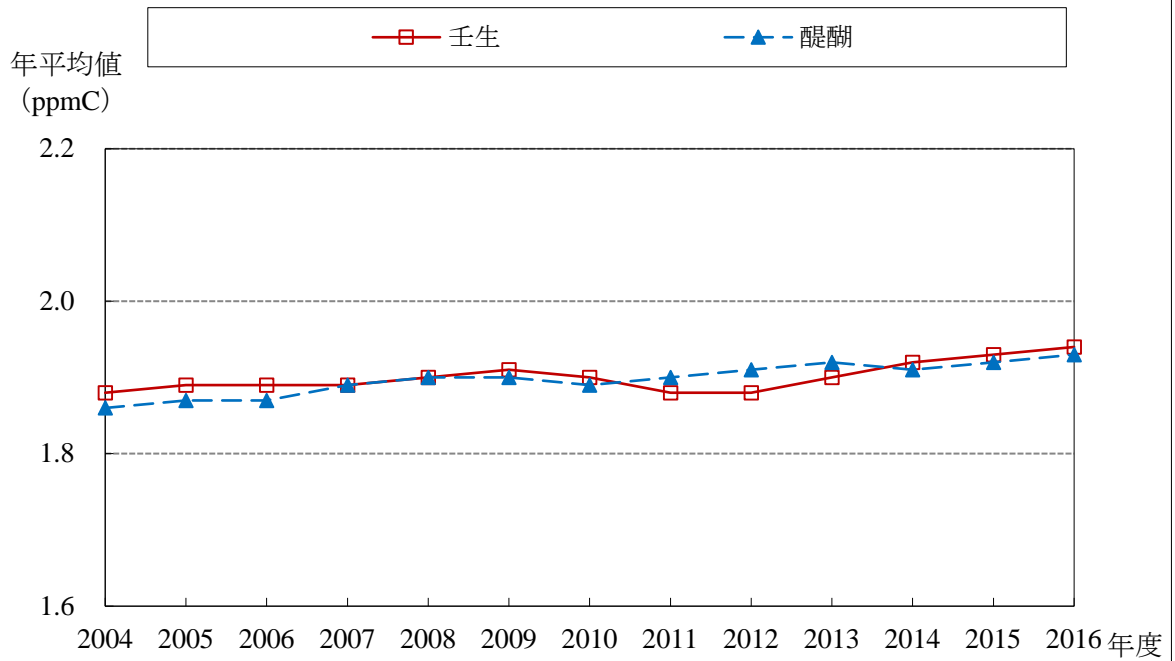
CH 4 経年変化グラフ (2004～2016年度)
