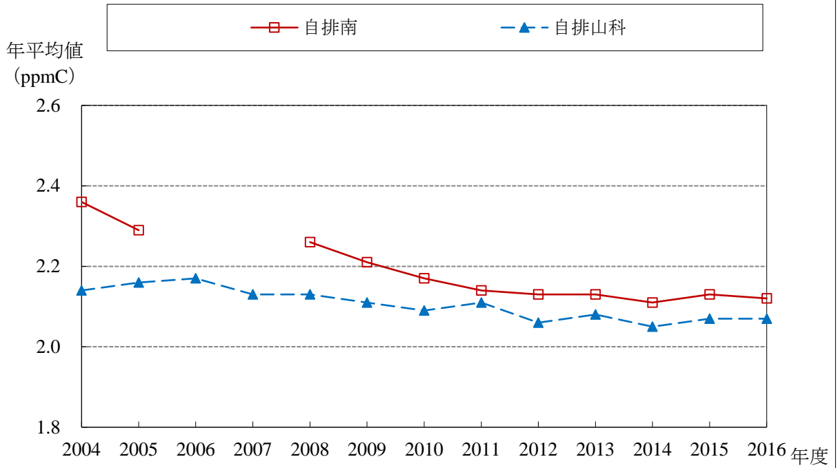
THC 経年変化グラフ (2004～2016年度)
