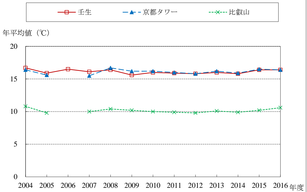
TEMP 経年変化グラフ (2004～2016年度)
