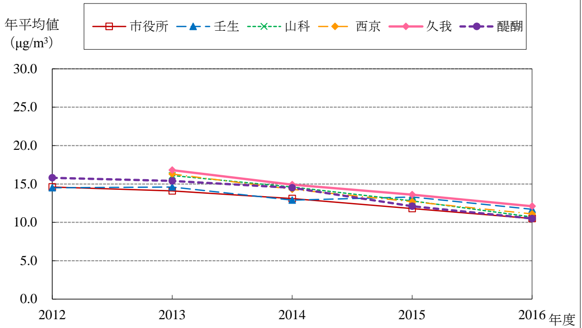
PM2.5 経年変化グラフ (2012～2016年度)
