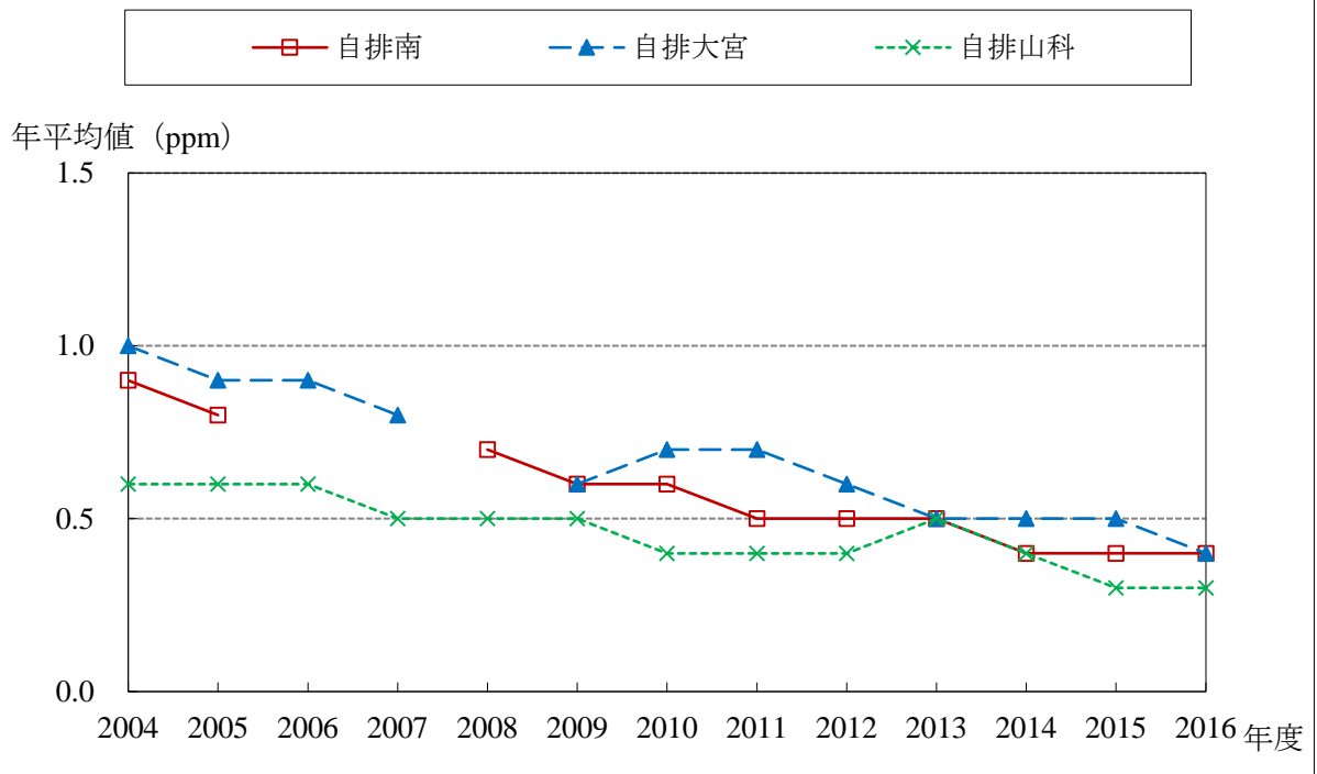
CO 経年変化グラフ (2004～2016年度)
