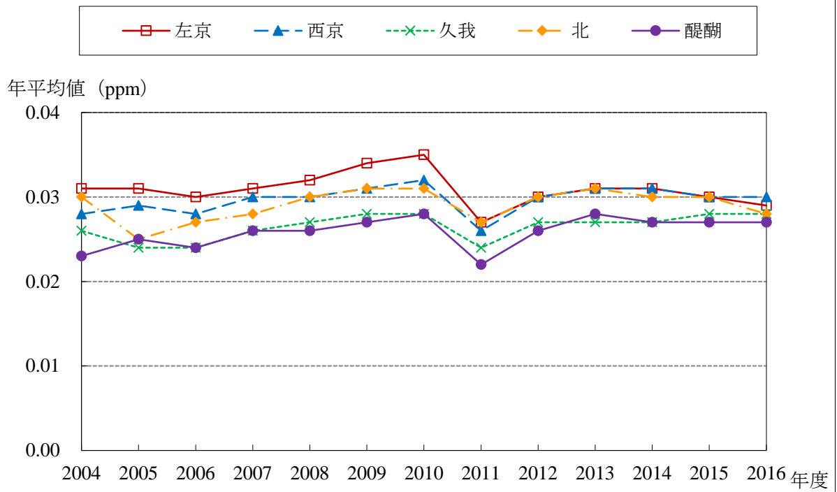
Ox 経年変化グラフ (2004～2016年度)
