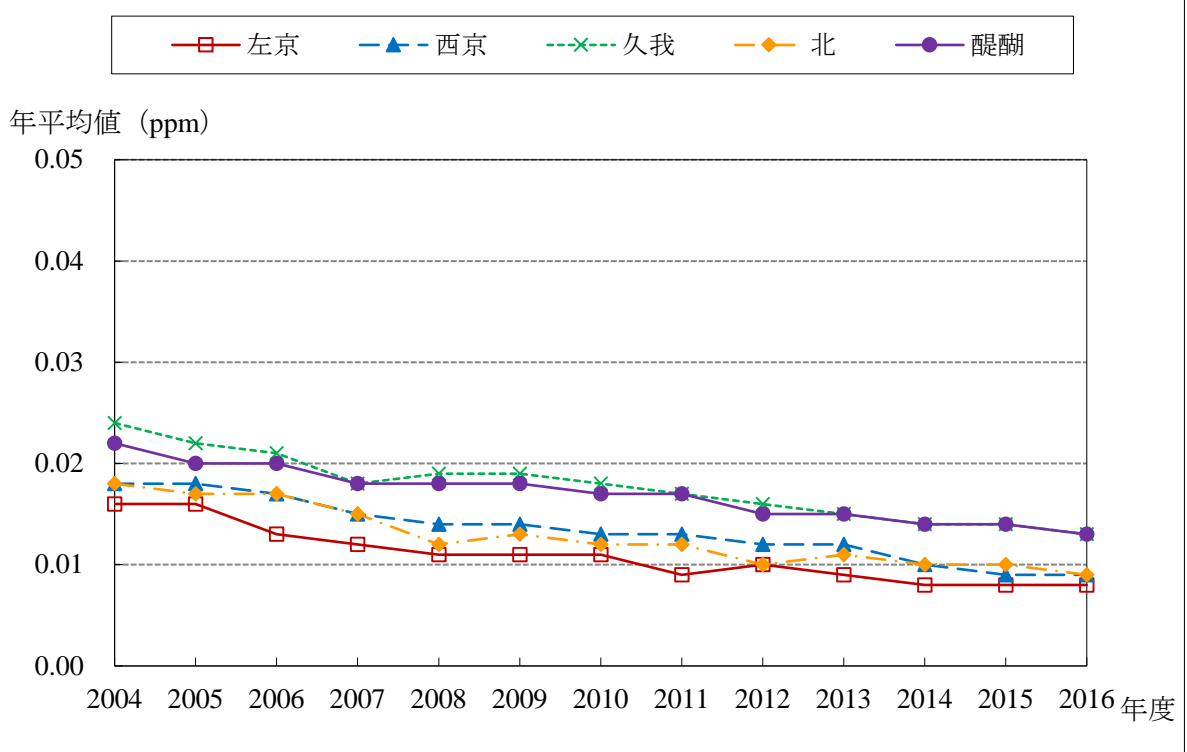
NO 2 経年変化グラフ (2004～2016年度)
