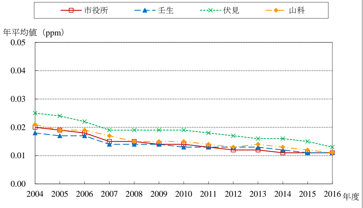
NO 2 経年変化グラフ (2004～2016年度)
