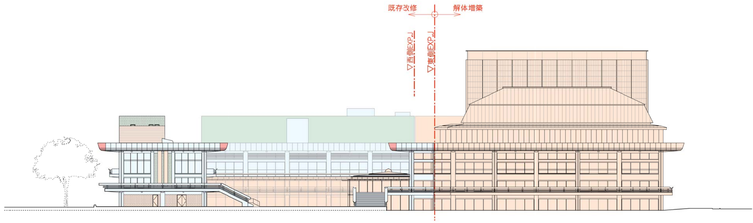
東側(岡崎公園・美術館別館側)立面図 改修部分色分け図
